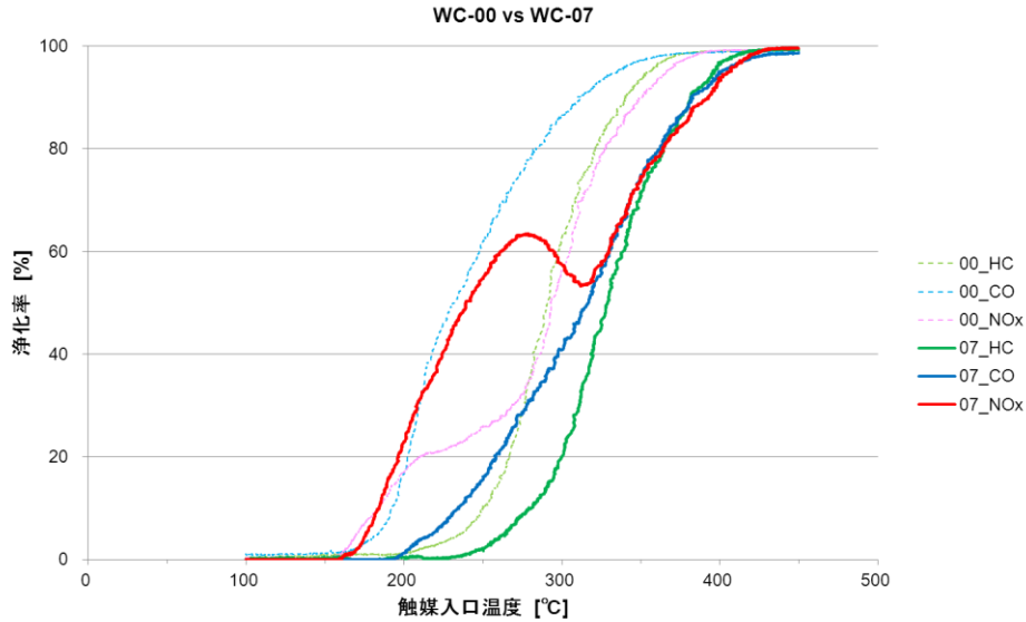
図 3-6 WC-07 の単体評価結果
