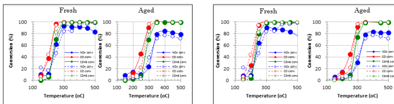
耐熱性アルミナ + セリア混合方法の改良によるセリア削減触媒のTWC結果(その1)
