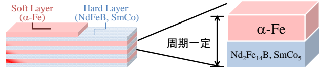
図1 人工積層型磁石の計算モデル
