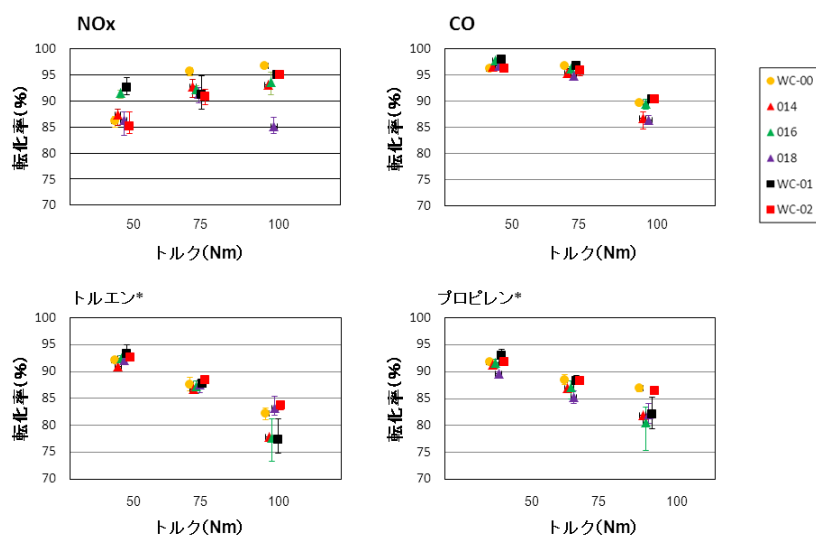
図 2-5-2-7 各触媒の転化率（回転数 2000rpm でトルクを変化）
