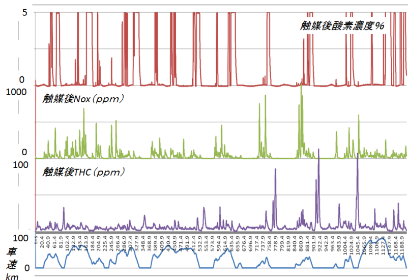
図 2-5-3-14 JC08 走行時の劣化触媒後の酸素、NO x 、THC 濃度
