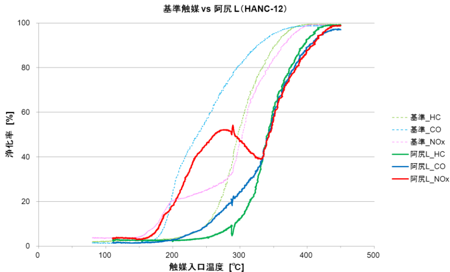
図 3-7 WC-07 同等材料の単体評価結果
