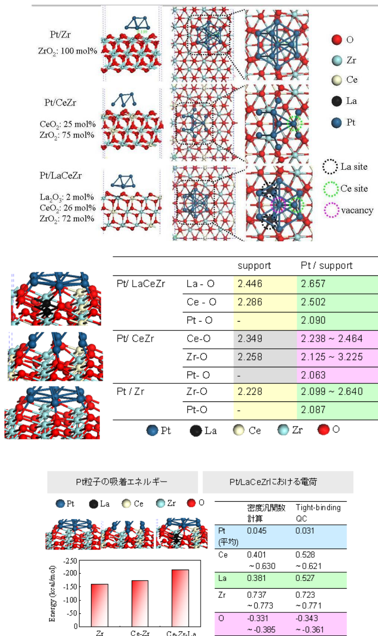
図 1-1-15 Pt/ZrO 2 , Pt/CeO 2 -ZrO 2 , Pt/La-dopedCeO 2 -ZrO 2 触媒の構造と電子状態、結合状態の計算結果
