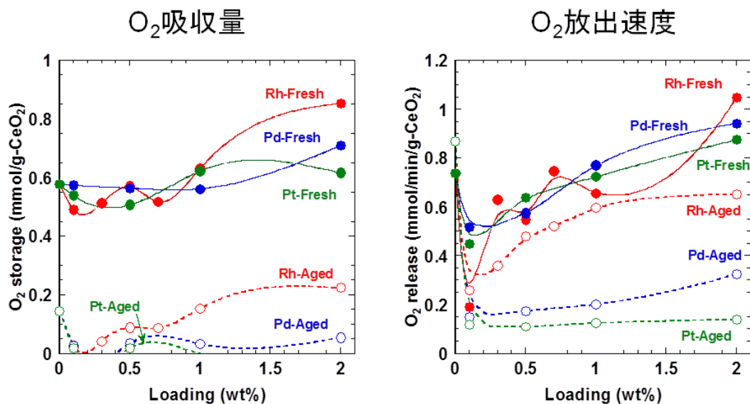
図 2-5-1-3 基準触媒 OSC 測定
