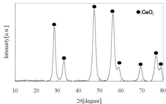
図 2-4-1-4 1.2wt%Rh/CeO 2 の XRD パターン
