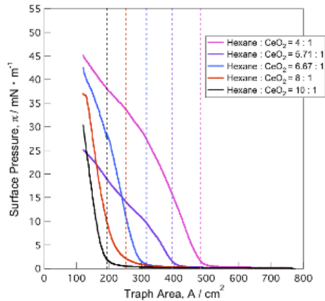
図 1-2-2 セリアナノ粒子コロイドの \Pi -A 曲線
