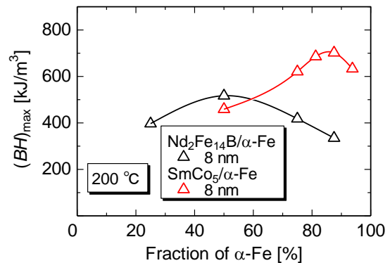
図3 200°Cにおける \text{SmCo}_5/\alpha\text{-Fe} 及び \text{Nd}_2\text{Fe}_{14}\text{B}/\alpha\text{-Fe} 人工積層型磁石で得られる (BH)_{\max} 値の \alpha\text{-Fe} 量依存性。積層周期は 8 nm に固定。
