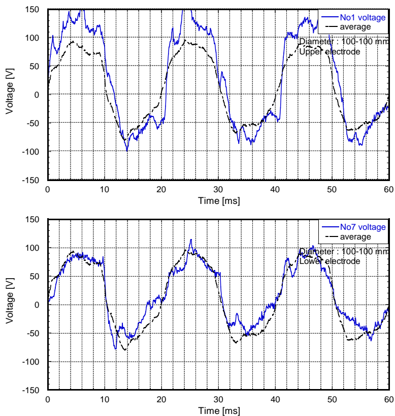
図Ⅲ-2-①-2-16 ハイブリッドプラズマ運転中の代表的な電圧波形：(a)上段電極，(b)下段電極
