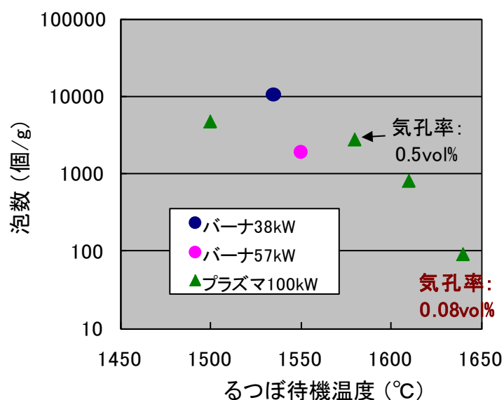
図Ⅲ-2-①-2-41 気中溶融したガラスブロック体におけるるつぼ待機温度と泡数の関係
