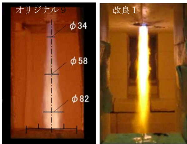
図Ⅲ-2-①-1-12 フレーム形状測定
