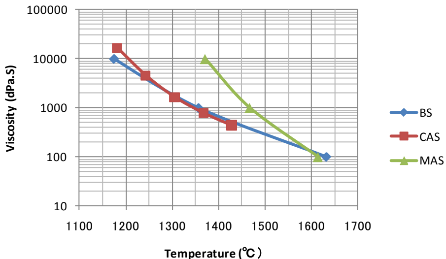
図III-2-①-2-70 CAS, MAS ガラスの粘性
