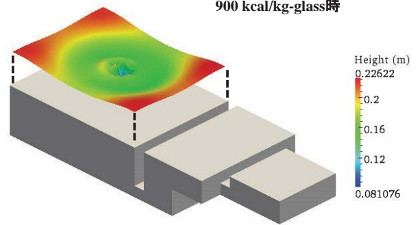
東洋ガラス試験炉の泡層厚さ(鳥瞰図)
