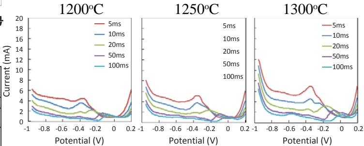
気中溶融ガラスCについて測定した矩形波ボルタノグラム
