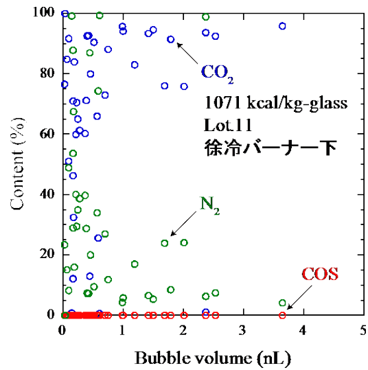
図III-2-①-3-15 冷却後にバーナー下より取り出した徐冷ガラス中の残存気泡ガス組成
