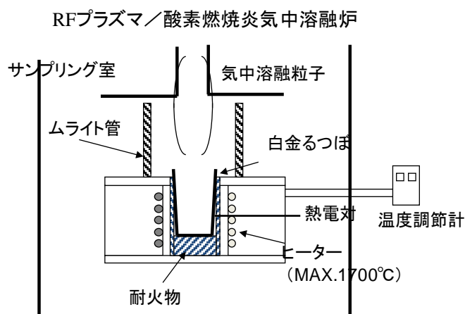
図Ⅲ-2-①-2-40 メルト採取実験装置模式図
