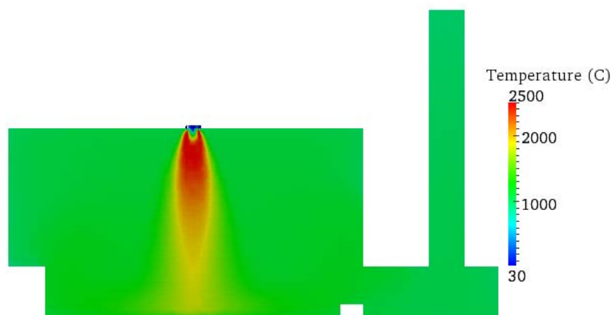
図Ⅲ-2-①-1-31 気中溶融時の温度分布 (35,000 step)
