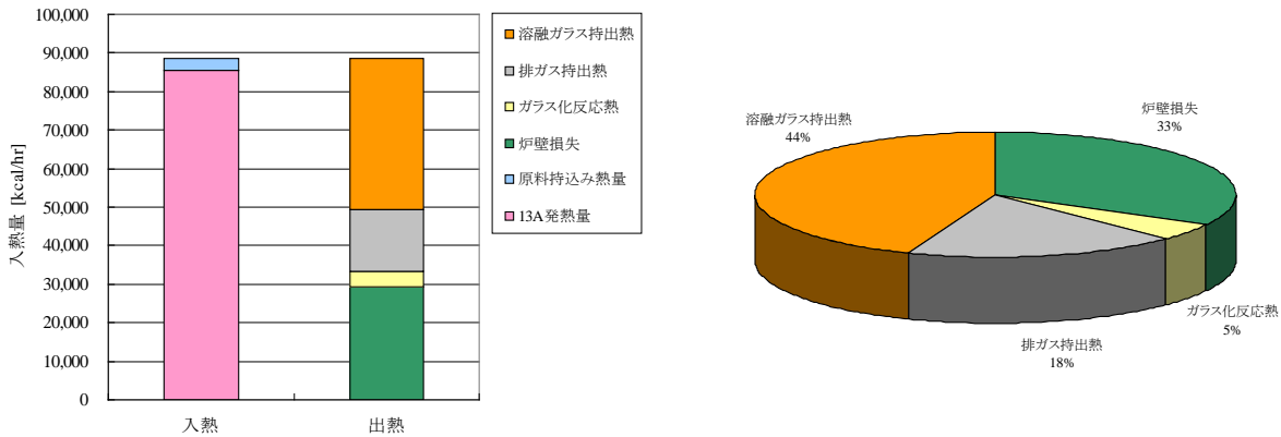
図III-2-①-3-77 気中溶融炉の熱精算
