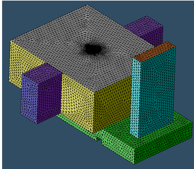
図Ⅲ-2-①-1-23 燃焼室メッシュ図（全体）
