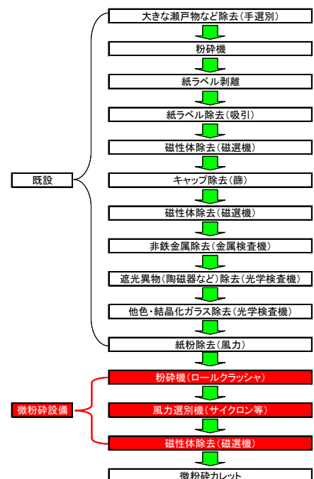
図Ⅲ-2-②-1-1 微粉砕フローチャート
