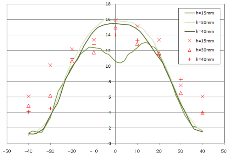
図III-2-①-3-47 ケース 2 の電子の放出面から 15mm( z=30\text{mm} )、電子の放出面から 30mm( z=15\text{mm} )、電子の放出面から 40mm(5mm)と x=0\text{mm} の軸上の流速[m/s]
