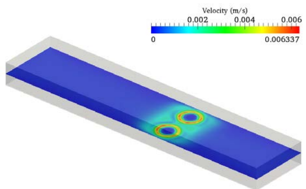
b) 流速絶対値 (スターラー形状非表示)
