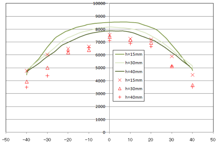
図III-2-①-3-48 ケース 2 の電子の放出面から 15mm( z=30\text{mm} )、電子の放出面から 30mm( z=15\text{mm} )、電子の放出面から 40mm(5mm)と x=0\text{mm} の軸上の鉛直方向下向きの温度[K]
