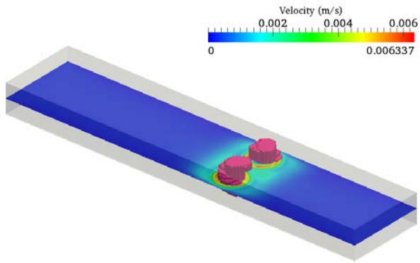
a) 流速絶対値
