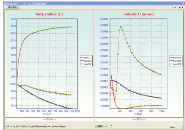
図Ⅲ-2-①-3-95 指定点の物理量変化
