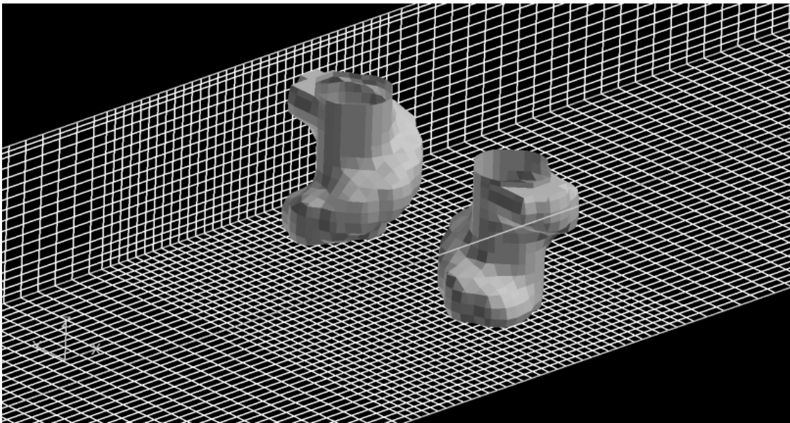
図Ⅲ-2-①-3-63 識別子によるスターラー形状の認識
