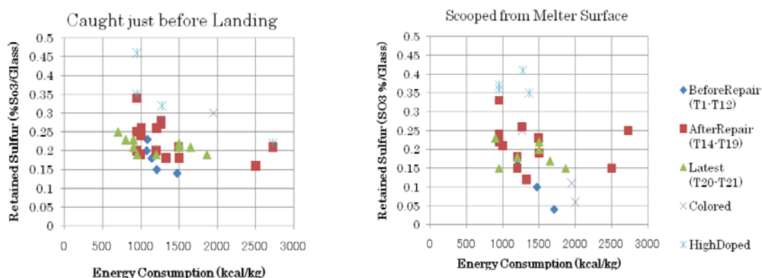
図Ⅲ-2-①-1-63 着地寸前の飛行粒子、着地後の採取素地における SO 3 残存量と原単位との関係
