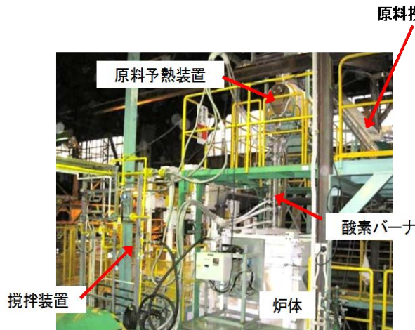
図Ⅲ-2-①-1-6 試験炉外観
