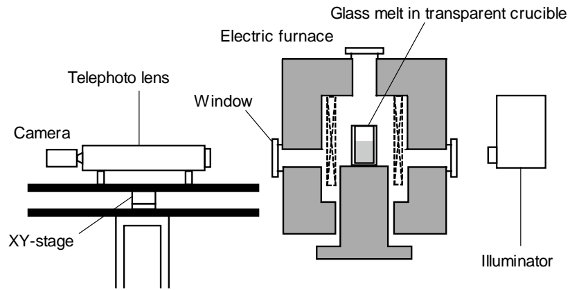
図Ⅲ-2-①-3-27 気中溶融ガラス融液直接観察装置概略図
