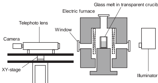
気泡挙動観察のための直接観察炉
