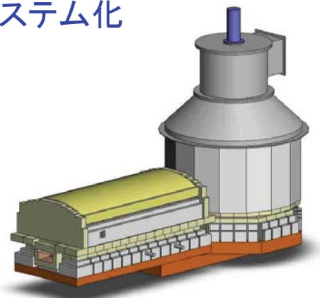
生産炉100ton/day炉のイメージ
