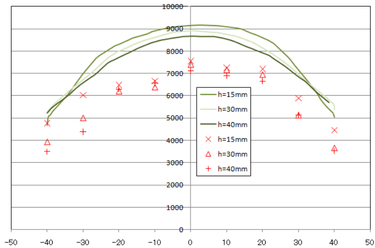
図Ⅲ-2-①-3-50 ケース 3 の電子の放出面から 15mm( z=30\text{mm} )、電子の放出面から 30mm( z=15\text{mm} )、電子の放出面から 40mm(5mm)と x=0\text{mm} の軸上の鉛直方向下向きの温度[K]
