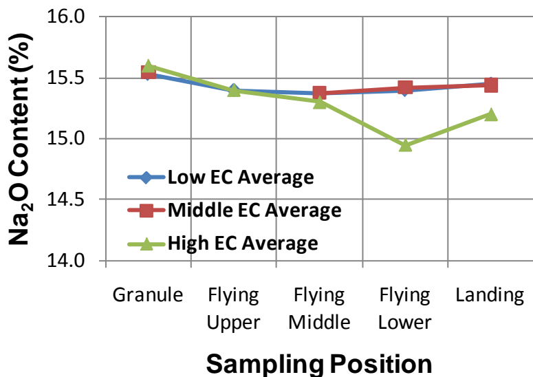
図Ⅲ-2-①-1-64 気中溶融過程でのアルカリの減損
