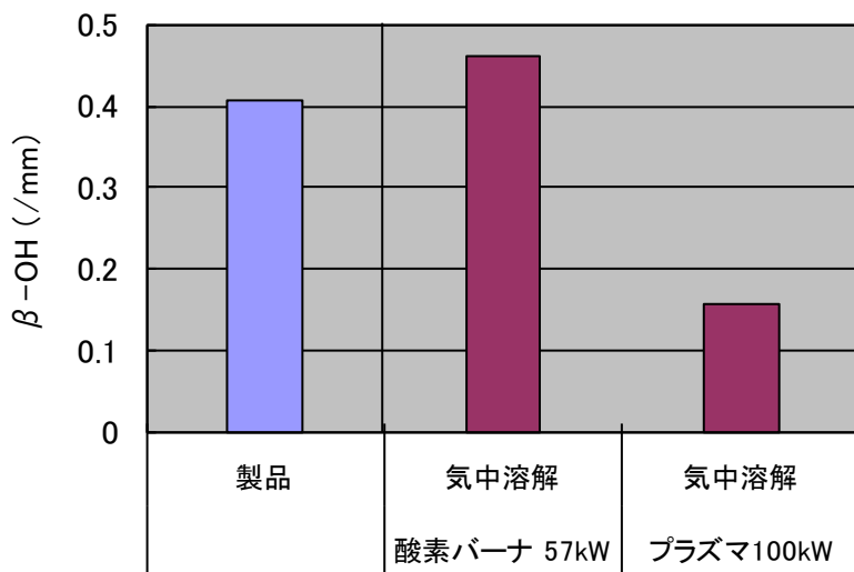
図Ⅲ-2-①-2-42 気中溶融ガラスと市販品の含水量の比較
