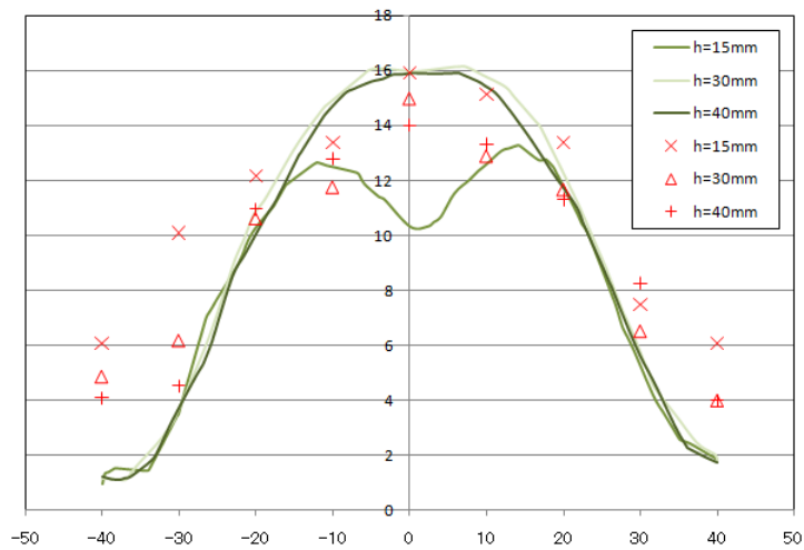
図Ⅲ-2-①-3-49 ケース 3 の電子の放出面から 15mm( z=30\text{mm} )、電子の放出面から 30mm( z=15\text{mm} )、電子の放出面から 40mm(5mm)と x=0\text{mm} の軸上の流速[m/s]
