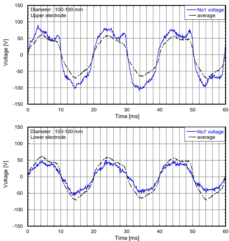
図Ⅲ-2-①-2-15 多相交流放電中の代表的な電圧波形：(a)上段電極，(b)下段電極
