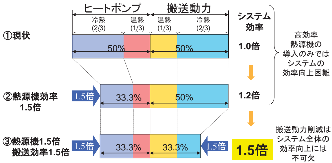
地域全体の業務用空調用エネルギー内訳概念図
