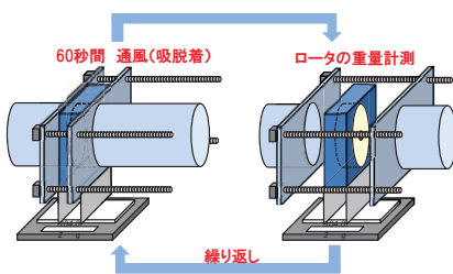
重量法による吸・脱着速度を計測
