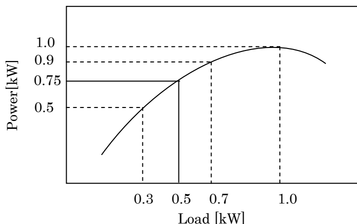
図-7 ヒートポンプの負荷率と消費電力の関係
