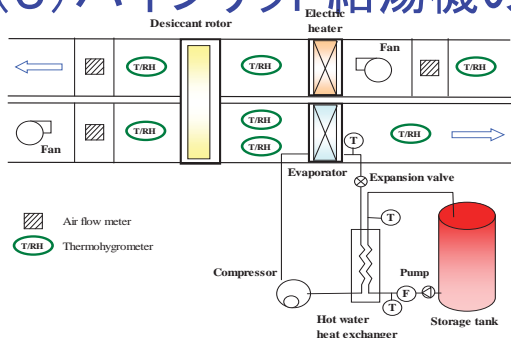
給湯機ハイブリッドサイクル1
