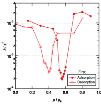
Zr-MPS粉末の25℃における水蒸気吸脱着緩和速度
