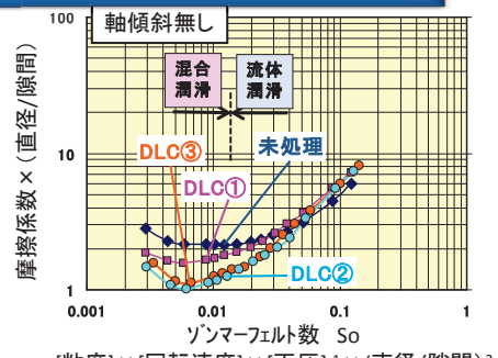
「最適化計算と効率予測」シミュレーションにより仕様を明確化
