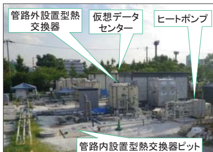
下水熱を利用した熱融通の実証
