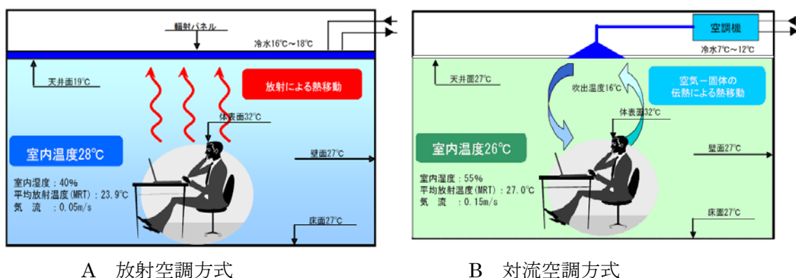
図-6 空調方式の違い（冷房の場合） <出典：清水建設 HP より>
