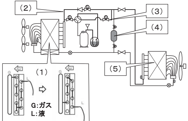
蒸気圧縮方式のパス 自然循環方式と蒸気圧縮方式の共用パス
