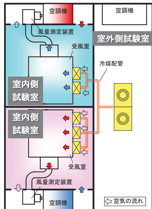
空調試験室のレイアウト (冷暖同時機)
