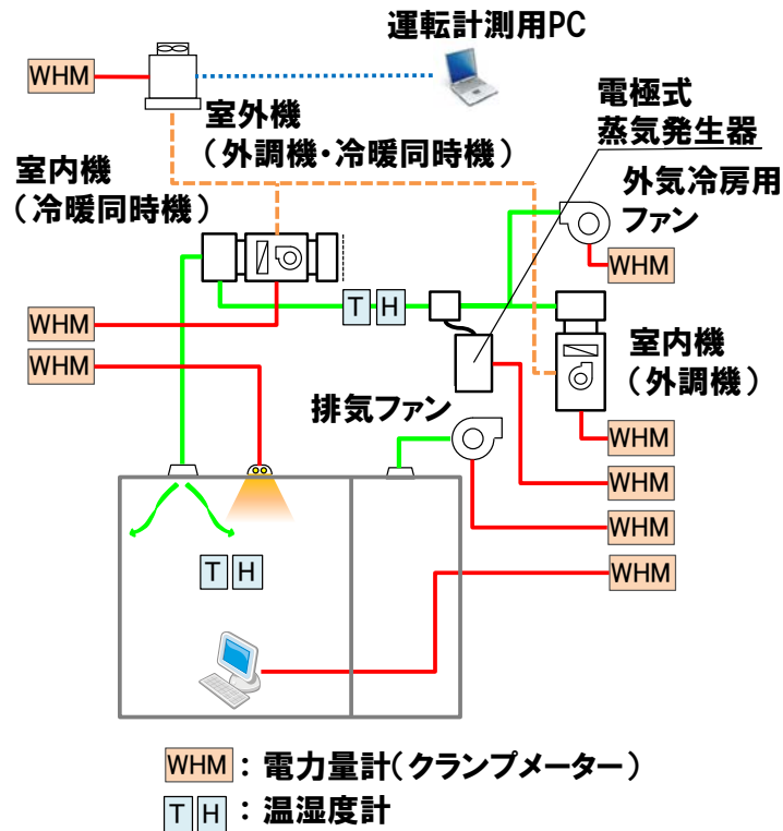
添付図 21 実証ビルでの計測概要
