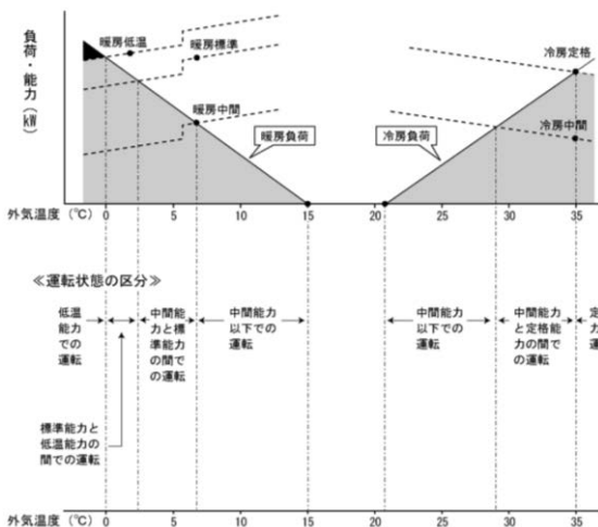
図 4.6.2 測定ポイントと外気温度による能力の変化
