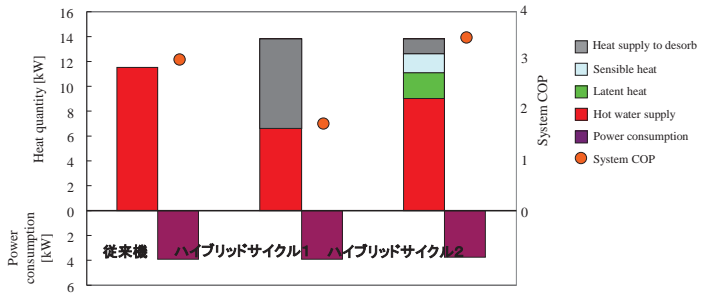
システム効率比較
