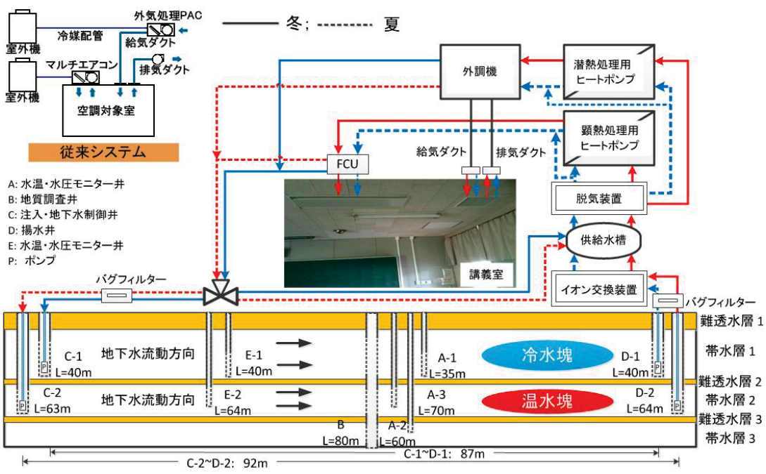
地下水制御型HPシステム概要
