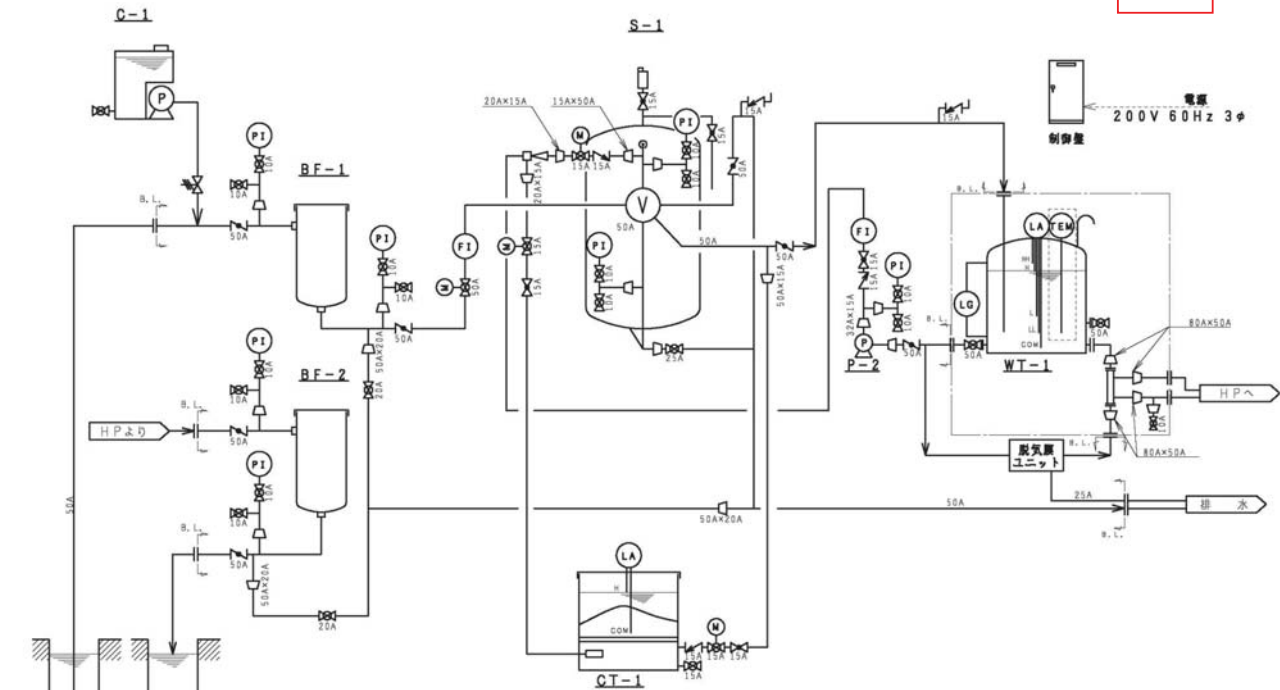
実証試験に採用したシステム系統図
