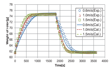
吸脱着速度への空気流速の影響
