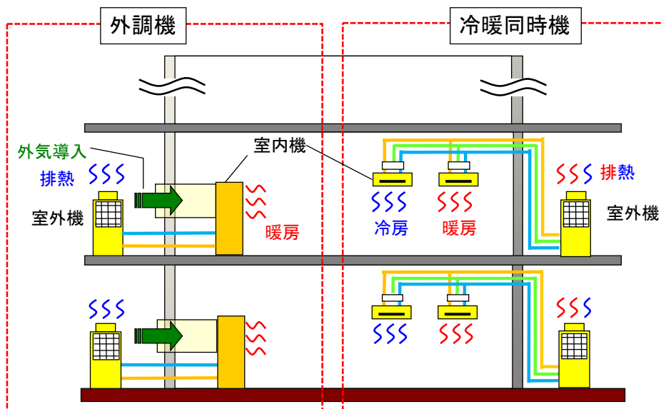
添付図2 研究開発対象の空調用ヒートポンプシステム (ビル用マルチエアコン)
