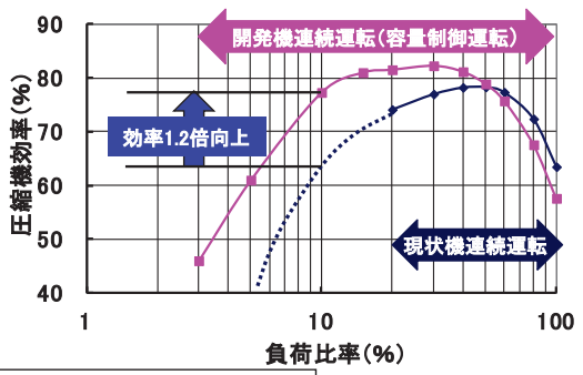
「最適化計算と効率予測」シミュレーションにより仕様を明確化
