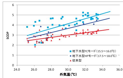
夏季の地下水利用フリークーリング運転、ヒートポンプ運転、従来型システムのCOP
