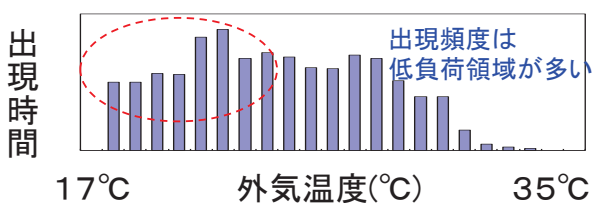
現在のヒートポンプ特性と外気温度出現時間 (JIS B 8616 事務所, 冷房期間, 東京)
