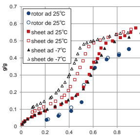
デシカントロータ・シートの常温・低温吸脱着特性
