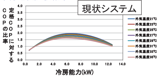
冷房運転試験結果
