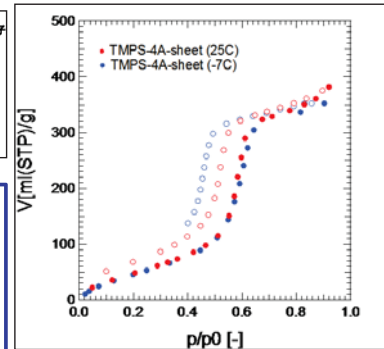
TMPS4A(シート上に塗布)の吸着・脱着等温線(-7℃と25℃)
