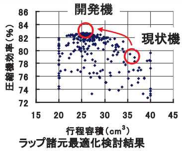
「最適化計算と効率予測」シミュレーションにより仕様を明確化
