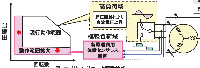
図 ワイドレンジモータ駆動技術
