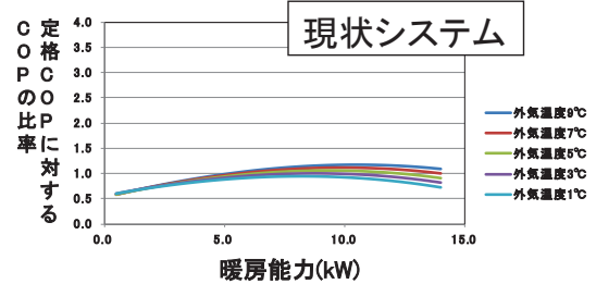
暖房運転試験結果
