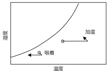
図 4.6.9 ハイブリッドシステム（暖房）
