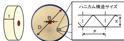
デシカントロータのシミュレーションモデル
