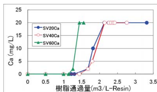
Caイオンに関する1再生あたり樹脂通水量
