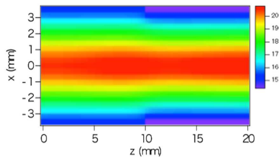
(b) 結晶内部温度分布
