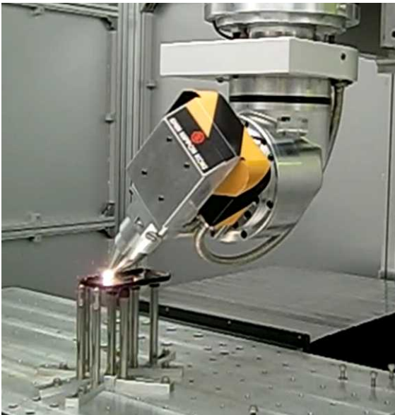
図IV-2.4(2).2 5軸加工機用倣い加工ヘッド
