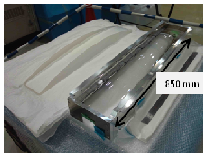
図Ⅲ-2-7-5 大型シリンドリカルレンズ(金型組み込み済みの組み合わせ集光レンズ) Ⅲ-2-7-(3)(事後)
