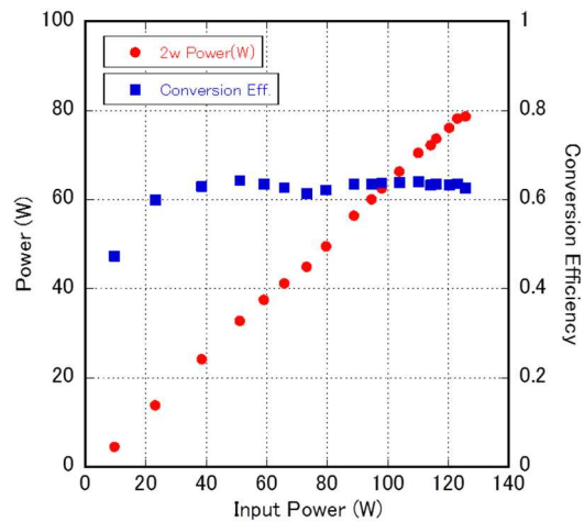
図Ⅲ2.2.4-41 ジグザク伝播波長変換の結果
