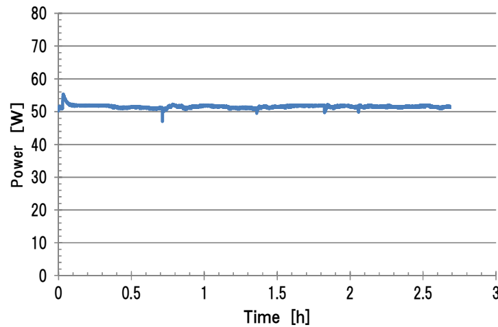
図Ⅲ2.1-16 10ns パルスシードレーザーの出力安定性
