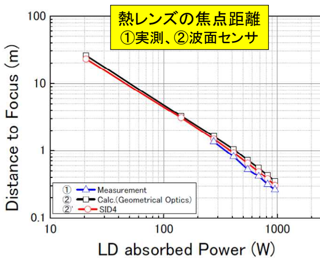
図Ⅲ-2.7.3 熱レンズ焦点距離
