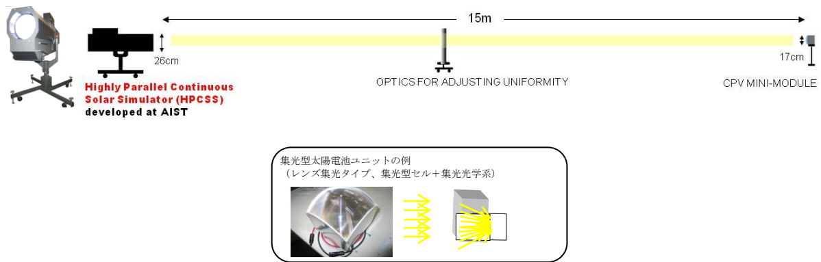
図 37. 集光型太陽電池ユニット評価用光源および性能評価の基本設計。光源の光出射部から被照射面までの距離を 15m とすることにより照射面中心からの視野角±0.5 度を実現した。また光路上に金属製メッシュを配置することにより、有効照射面における照度均一性が調整可能である。
