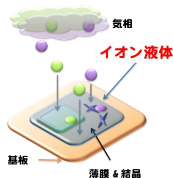
図 21. フラックス気相成長法
