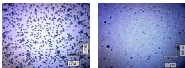
図 17. Si0G 基板上にバッファ層無 (左) 有 (右) で反応性 CVD 成長した \text{Si}_{0.5}\text{Ge}_{0.5} 膜のエッチング後顕微鏡写真
