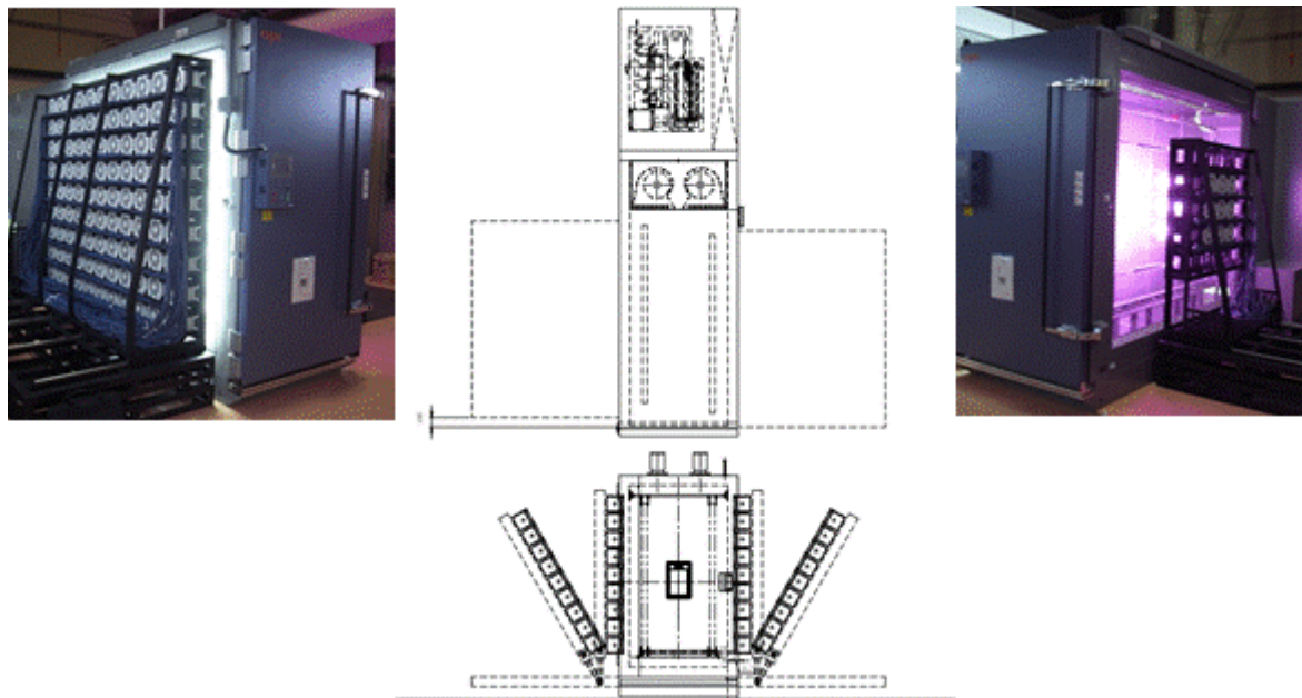
図 48. LED 式光照射試験装置
