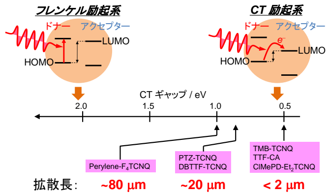
図 25. 拡散長と CT ギャップの関係
