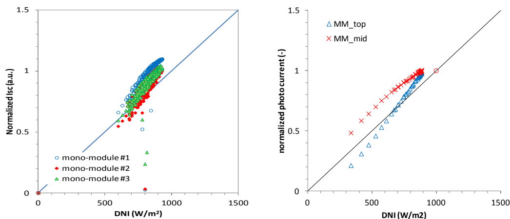
図 42. スペクトルによる発電性能変化（左：実測、右：シミュレーション）
