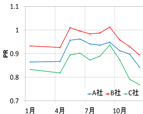
図 43. 3社のセル性能 (PR) 比較
