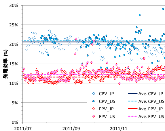
図 41. 日米発電効率比較 (集光型および非集光型)
