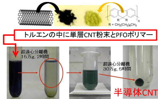
図 23. 半導体 CNT の抽出工程
