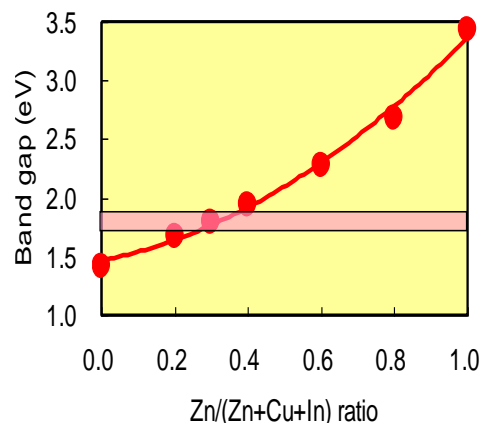
図 32. ZCIS の組成とバンドギャップ
