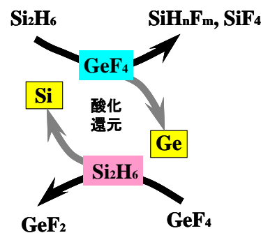
図 18. \text{GeF}_4 - \text{Si}_2\text{H}_6 系の反応
