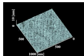
図 22. ピコステップガラスの AFM 像
