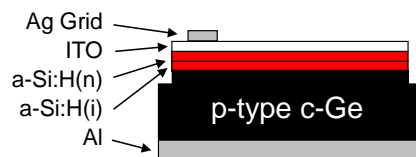
図 11. 作製したデバイス構造
