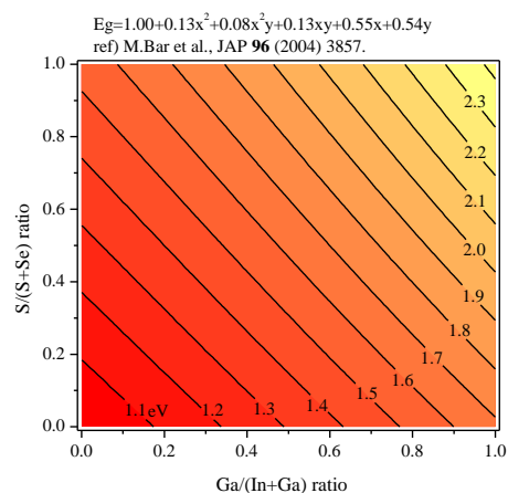
図 30. CIGSSe の組成とバンドギャップの関係
