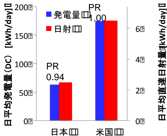
図 40. 日米発電性能 (PR) 比較 (日平均発電量と日平均直達日射量)
