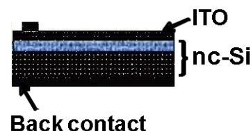
図 28. ナノ結晶シリコン自立膜セルの構造
