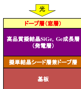
図 19. 目標とする SiGe 系薄膜ボトムセルの構造
