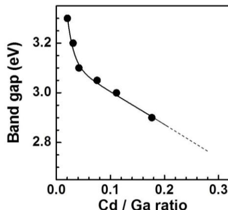
図 33. アモルファス Cd-Ga-O のバンドギャップ
