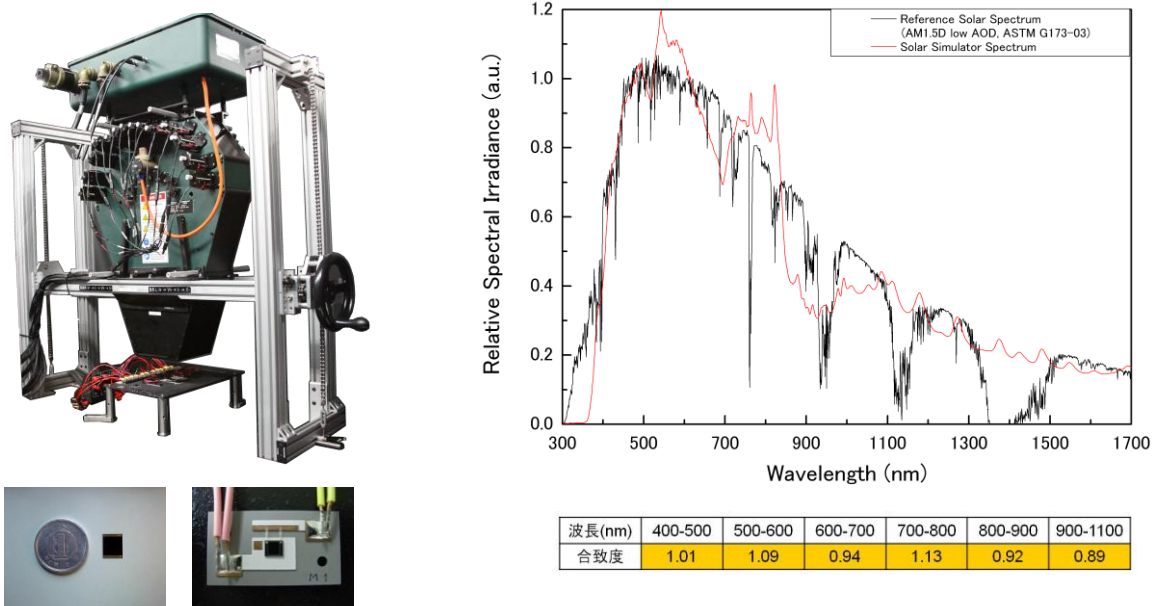
図 35. 照度および分光放射照度スペクトル調整機構を備えた集光型太陽電池セル評価用光源（左上図）および集光型太陽電池セルの一例（左下図）。高精度測定を行う上で必須となる性能の一つである基準太陽光とのスペクトル合致度（右図）は約±10%以内であり、ASTM 規格 E927-10 において class A を満たしている（黒線：基準太陽光の分光放射照度スペクトル、赤線：ソーラーシミュレータの分光放射照度スペクトルの一例）。
