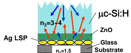
図 15. プラズモン効果の概念図
