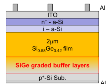
図 16. 試作した SiGe ヘテロ太陽電池の構造
