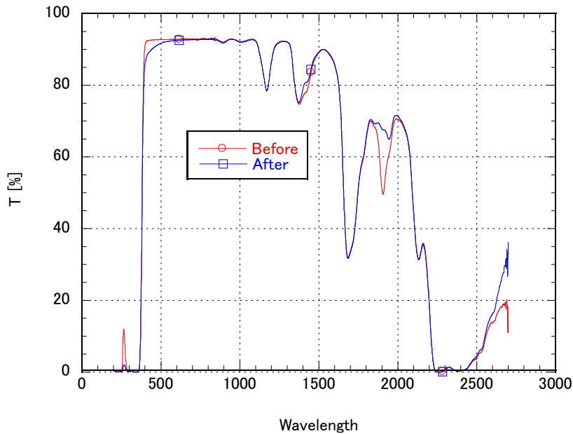
図 49. 集光型太陽電池のレンズ部材（アクリル）の光照射試験結果
