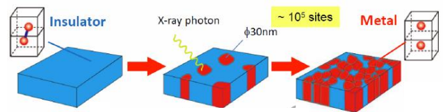
図 26. W:VO 2 における多重キャリア生成
