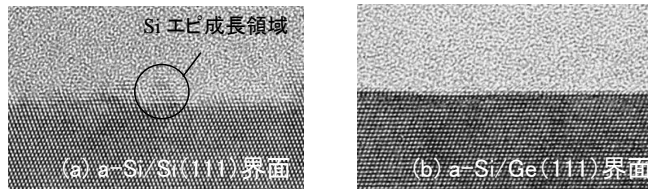
図 12. ヘテロ界面の TEM 断面像
