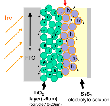
図 29. コア/シェル構造 Si 量子ドット増感型太陽電池の構造
