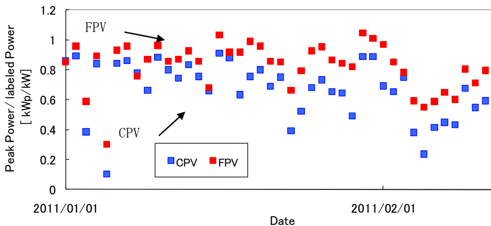
図 45. ラベル出力値あたりのピーク AC 出力比較 (2011 年 1 月 1 日～2 月 12 日) 青■：集光型太陽光発電システム (CPV)、赤■：レファレンス PV システム (FPV)
