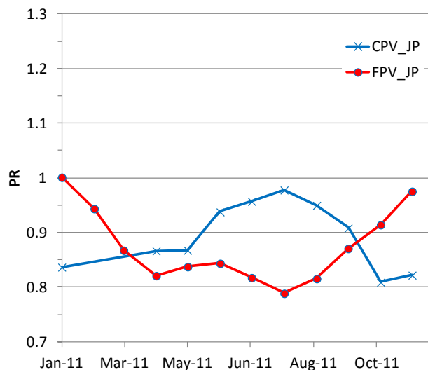
図 46. パフォーマンスレシオ (PR) の比較 (日本サイト) 青線：集光型太陽光発電システム (CPV)、赤線：レファレンス PV システム (FPV)
