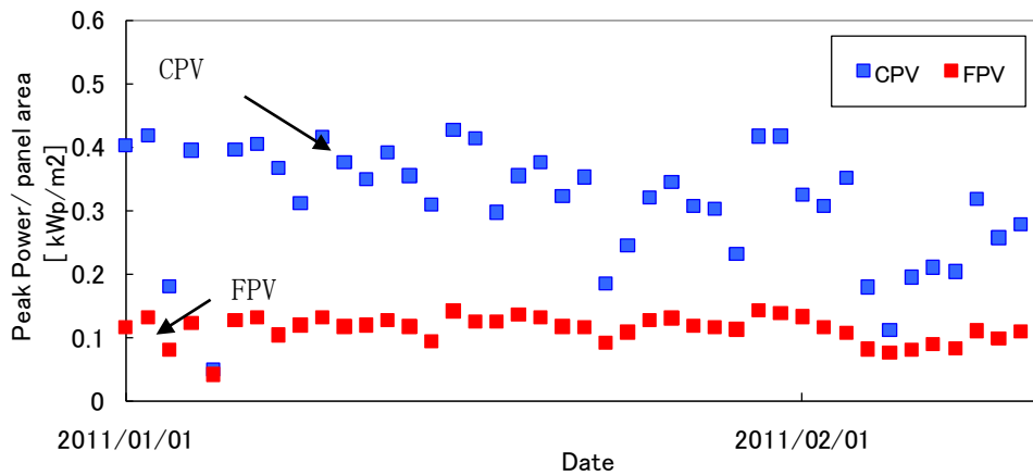
図 44. 単位面積あたりのピーク AC 出力比較 (2011 年 1 月 1 日～2 月 12 日) 青■：集光型太陽光発電システム (CPV)、赤■：レファレンス PV システム (FPV)
