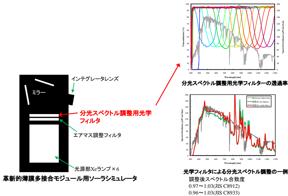
図 47. 革新的薄膜多接合モジュール性能評価用ソーラシミュレータと、3 接合以上に対応したスペクトル調整技術
