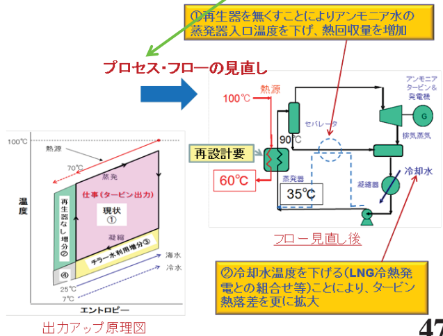
出力アップ原理図
