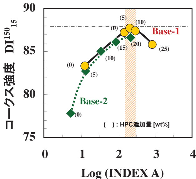
INDEXとコークス強度の関係
