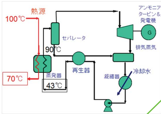
カーリーナ発電設備
