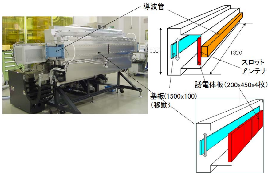
図Ⅲ-2. 2B. 1-5 大型基板検証用 SWP-CVD 装置
