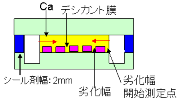
図Ⅲ-2.2A.1-3 デシカント膜の封止特性の評価セル構造
