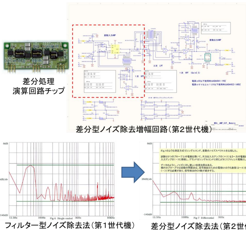
図 2 信号ノイズ除去のためのハードウェア開発 (第2世代機用差分型ノイズ除去回路)
