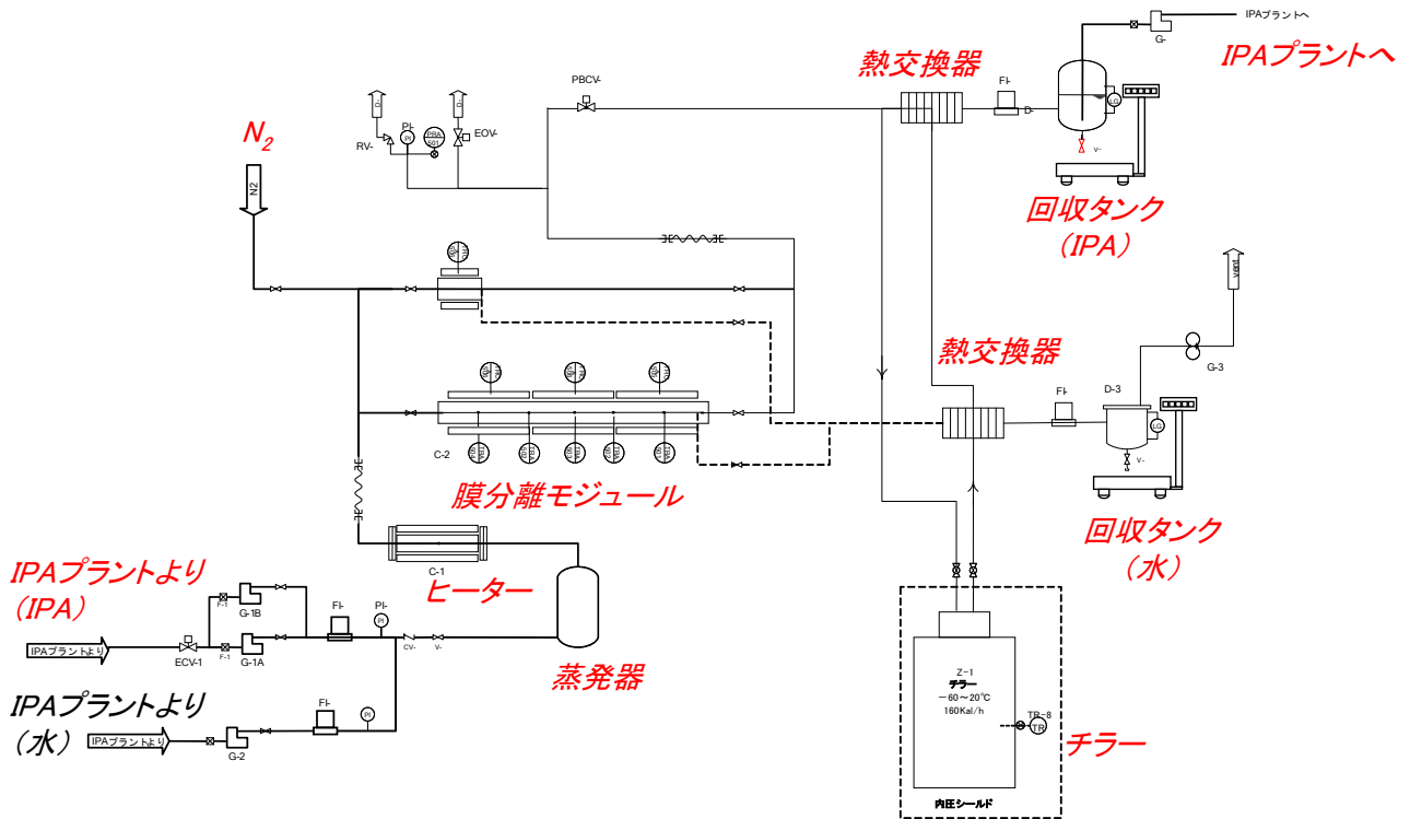
図 2.4.1-5 実証試験装置フロー概略図
