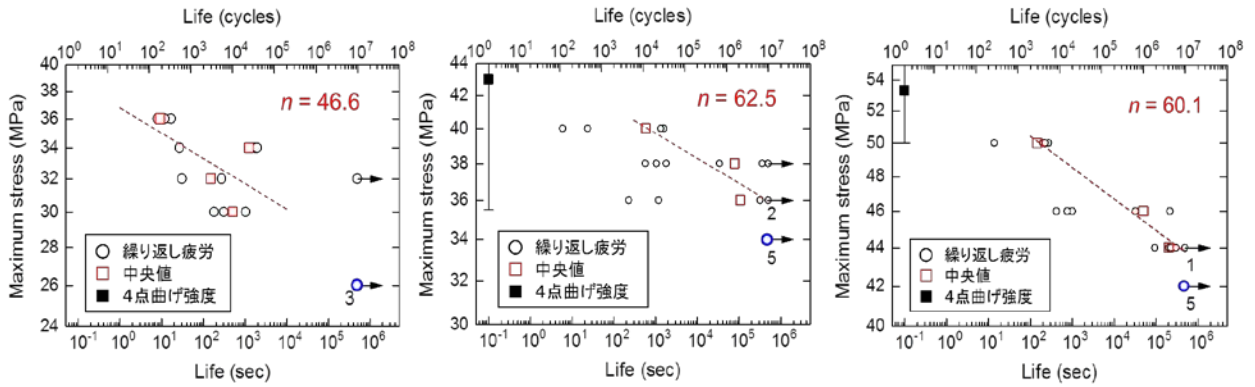
図 2.2.2-12 繰り返し疲労試験の S-N プロット(左)d017-P45(中)d070-P45(右)d970
