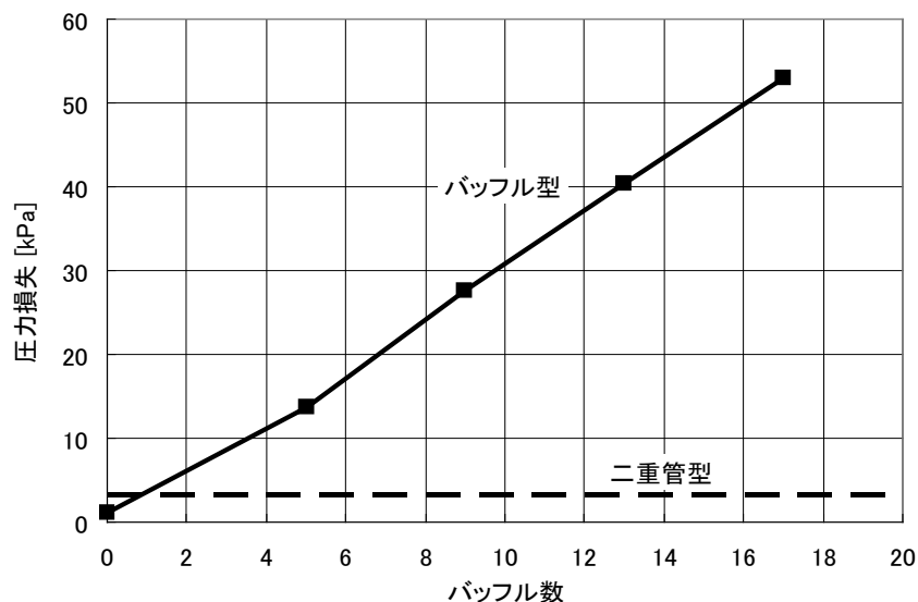
図2.3.1-12 熱移動モデルの解析結果（圧力損失）
