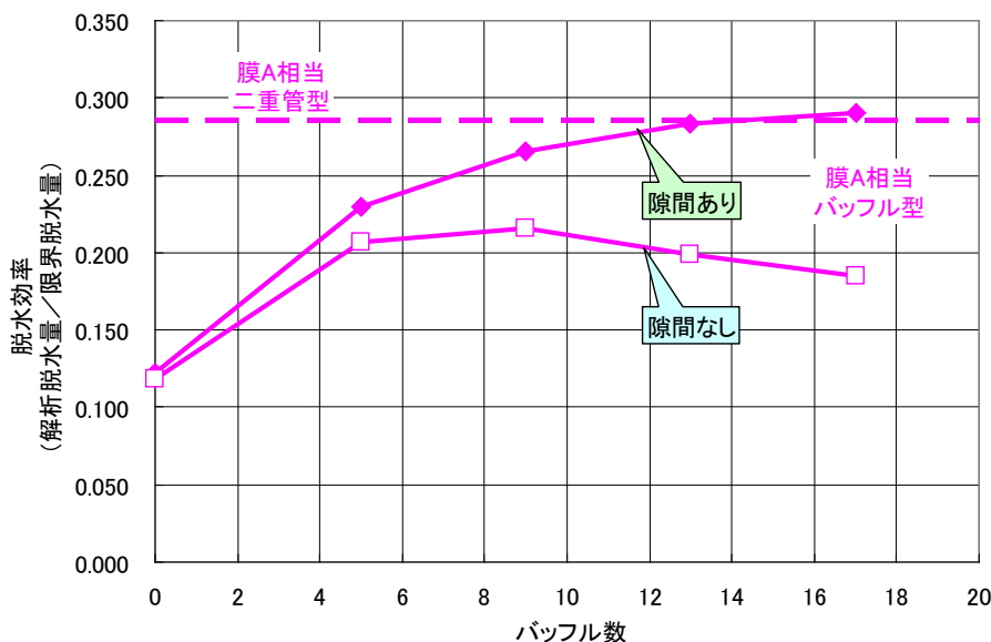
図2.3.1-16 バブル型モジュールの改良案
