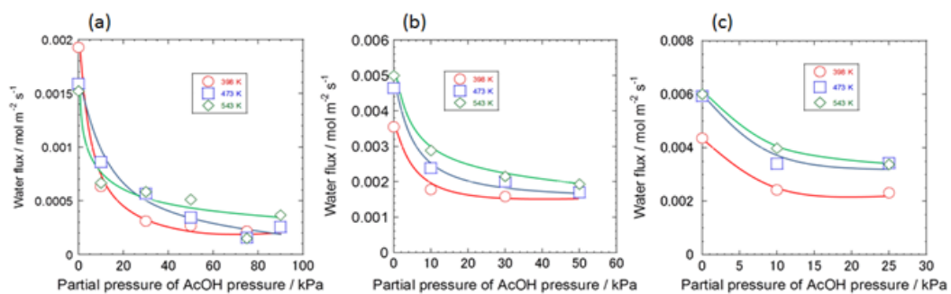
図 2.1.1-9 水供給分圧一定条件下での酢酸供給分圧が MOR 型ゼオライト膜の水/酢酸混合蒸気透過分離特性に及ぼす影響
