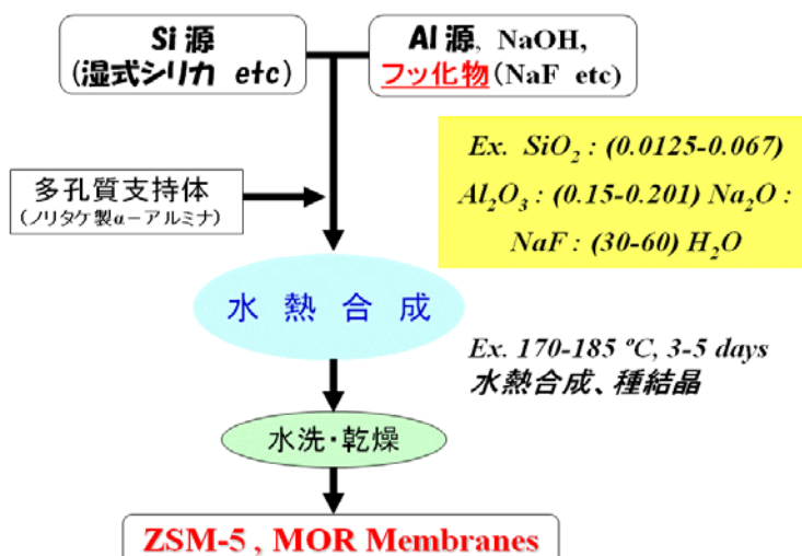
図 2.1.1-60 F イオン含有ゲルでの ZSM-5 膜製膜手順
