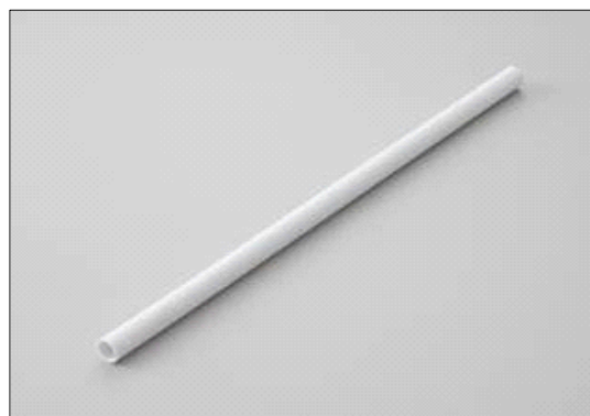
図 2.2.1-2 規則性ナノ多孔膜精密分離膜用多孔質アルミナ基材 (NS-1) の外観 (仕様：外径 10mm 内径 7mm 長さ 400mm)
