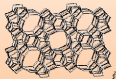
ZSM-5 { 0.56 nm × 0.53 nm 0.55 nm × 0.51 nm
