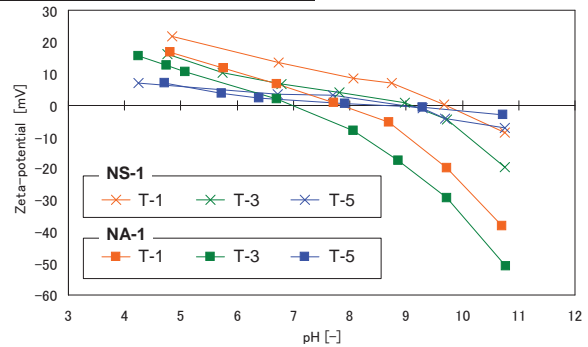
焼成温度を変更した基材NS-1, NA-1の 細孔表面ゼータ電位測定結果
