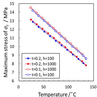
図 2.3.2-18 ガラスシール部の最大応力値の温度変化
