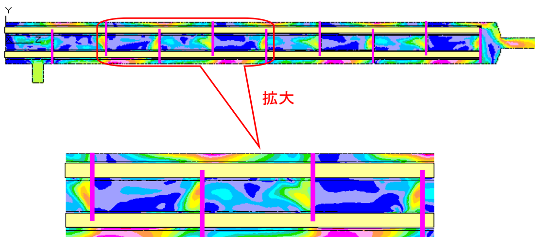
図2.3.1-12 熱移動モデルの解析結果（圧力損失）
