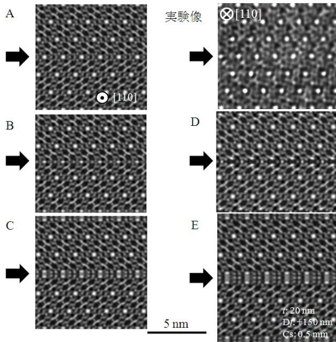
図 2.1.2-12 理論計算によって得られた緩和構造の TEM 計算像 A が実験結果と最も良く一致している。
