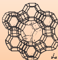
Y型 0.74 nm
