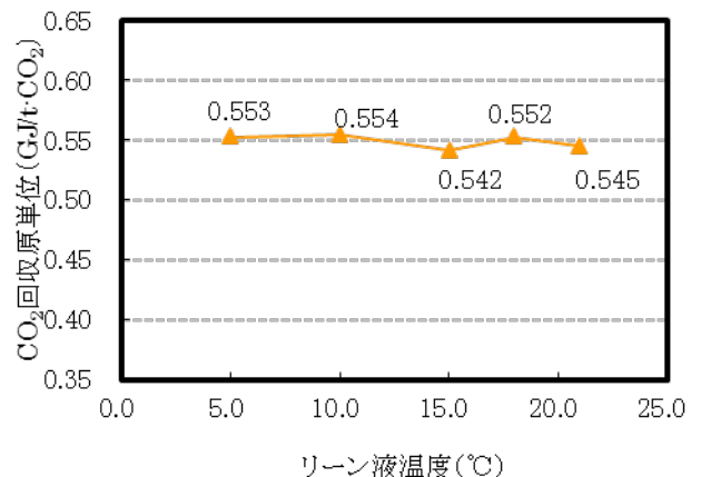
図III-2-41CO 2 回収原単位
