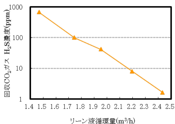
図Ⅲ-2-21 回収 \text{CO}_2 中 \text{H}_2\text{S} 濃度
