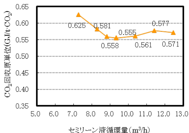
図Ⅲ-2-27 CO 2 回収原単位
