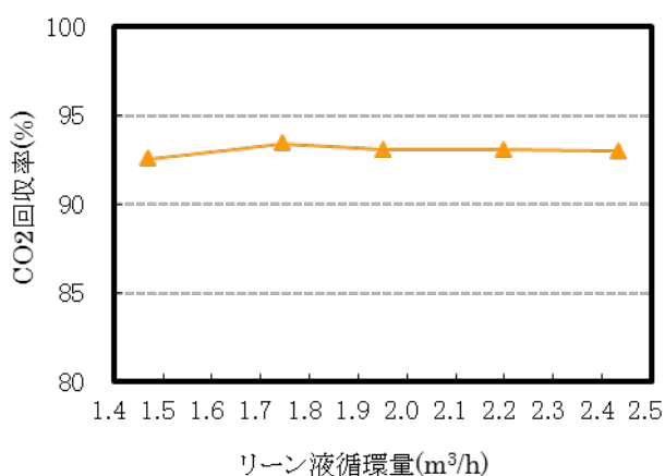
図Ⅲ-2-20 \text{CO}_2 回収率
