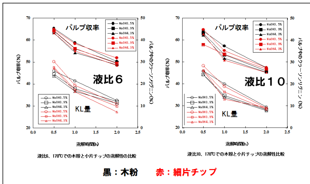
図Ⅲ-2.2.2.2-5 スギ木粉および細片チップの静置蒸解による蒸解性の差異
