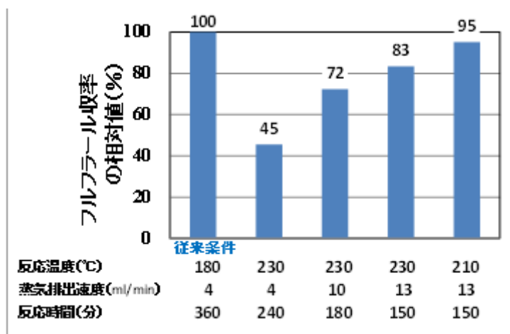
図Ⅲ-2.1.2-6 反応温度変更によるフルフラール収率の相対値
