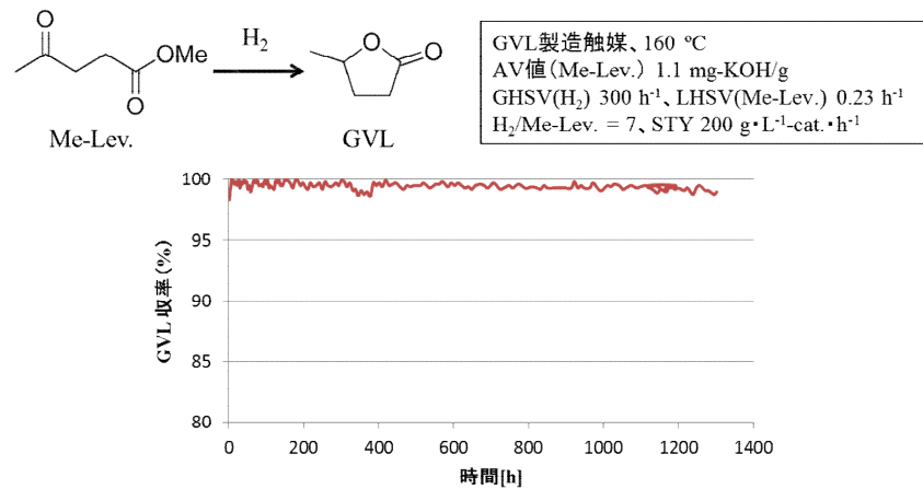
図Ⅲ-2.2-2.8-4 GVL 製造触媒の寿命評価
