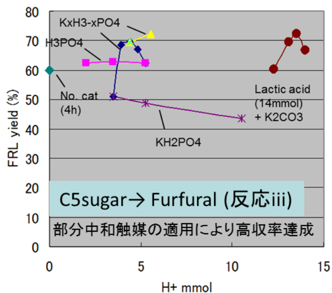
図 III-2.2.2.5-20 C5 糖脱水反応におけるフルフラール収率
