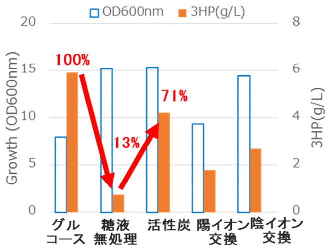
図III-2.2.2.10-15 木質由来糖液の前処理の3HP生産量低下軽減効果
