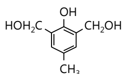
図Ⅲ-2.2.2.9-3 2,6-ビスヒドロキシメチル- p -クレゾールの分子構
