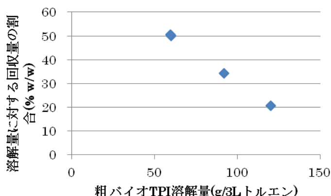
図Ⅲ-2.1.1-3 粗バイオ TPI の溶解量とその回収物の割合
