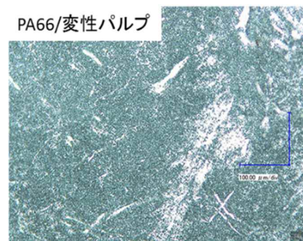
図Ⅲ-2.2.1-14 CNF/PA66 の CNF 分散状態の光学顕微鏡像
