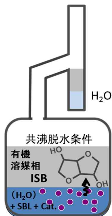
図 III-2.2.2.10-18 2相反応法概念図
