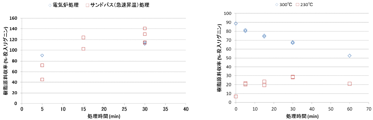
図III-2.2.2.4-5 処理時間が樹脂原料収率に与える影響 左：アセトン/水処理 右：高温高压水処理
