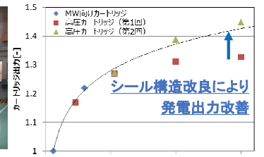
カートリッジのシール構造改良
