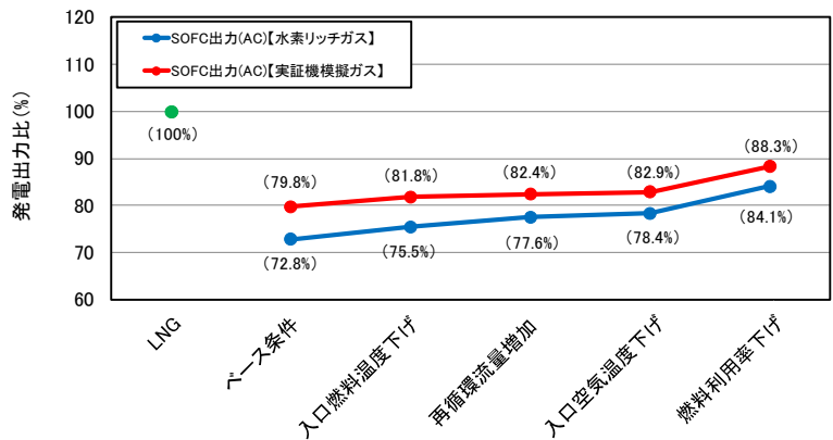
図 3-2-3-26 実証機模擬ガス最大負荷試験における発電出力推移
