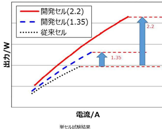
図 3-2-1-29 高性能セルスタックによる出力増加（独自開発）
