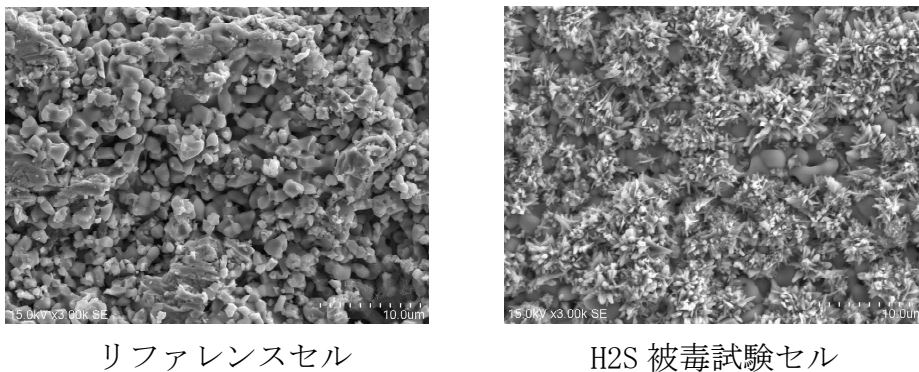
図 3-2-2-10 基体管内表面における SEM 観察結果
