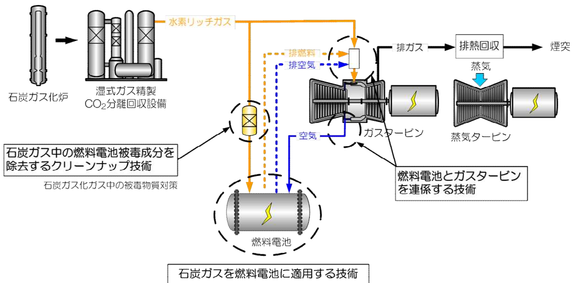
図 3-2-4-1 IGFC を構成する要素技術
