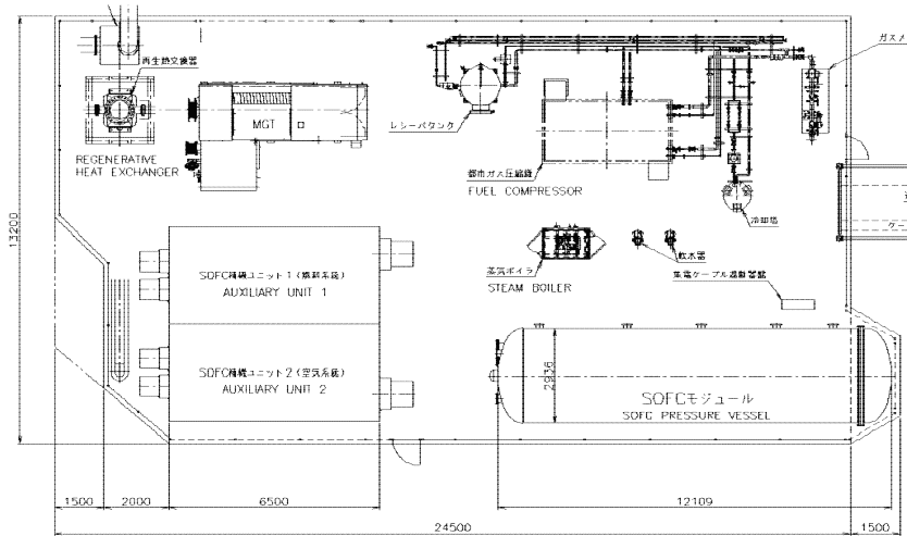
設備配置
