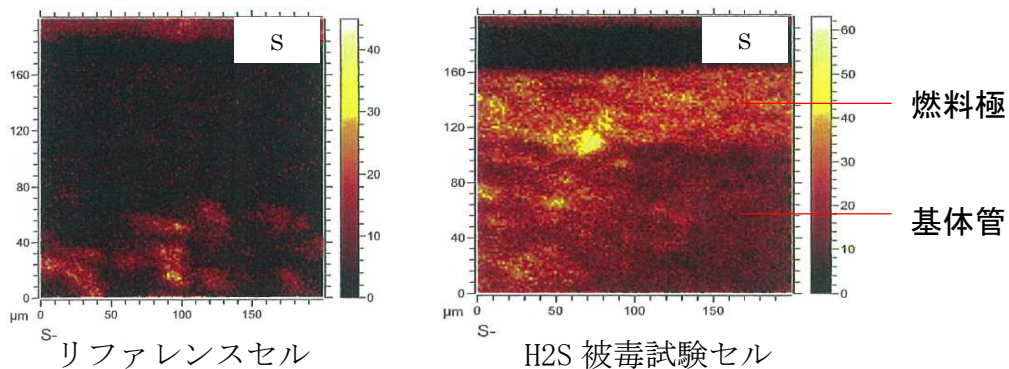
図 3-2-2-11 燃料極/基体管全体における SIMS 分析結果
