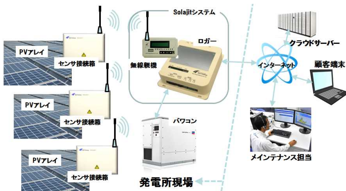
図Ⅲ-2-②-(2)-8 遠隔監視システム
