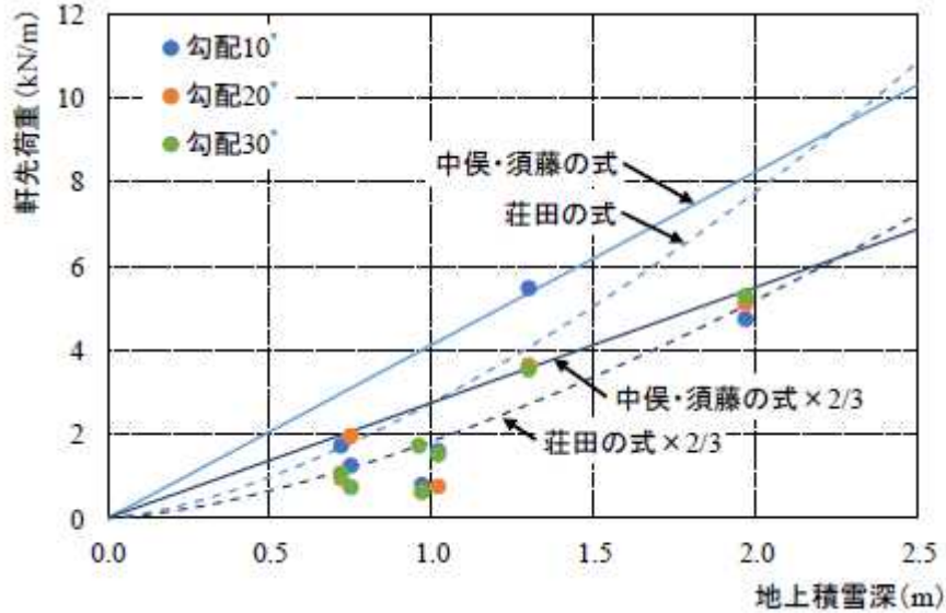
図Ⅲ-2-④-(1)-5 地上積雪深の軒先荷重との関係
