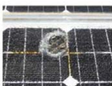
①モジュールの破壊やジャンクションボックスの事故例調査
