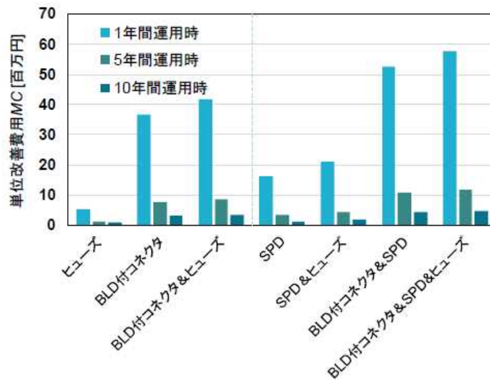
図Ⅲ-2-④-(1)-4 単位改善費用 (1年, 5年, 10年運用時)
