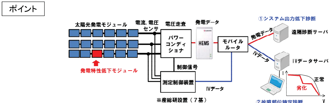
遠隔自動診断のモニタリングシステムイメージ
