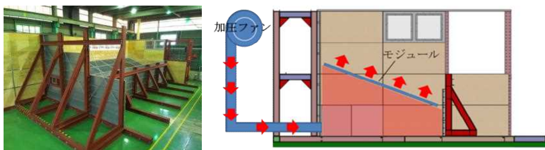
図Ⅲ-2-①-(5)-6 試験装置概要（左：試験装置全景，右：負圧载荷の例）
