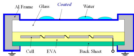
図 III-2-②-(4)-4 抗PID化コーティング（青の部分）
