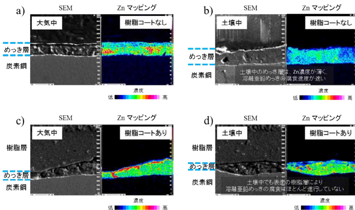
図Ⅲ-2-④-(3)-27 表面処理を施した一般構造用炭素鋼鋼管を浅層土壌中で1年間暴露後の断面観察結果
