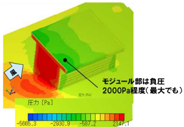
図Ⅲ-2-①-(6)-5 耐風性のシミュレーション
