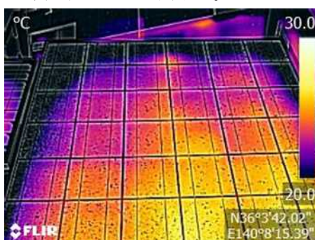
図Ⅲ-2-②-(3)-22 【バイパスダイオード／発熱前】
