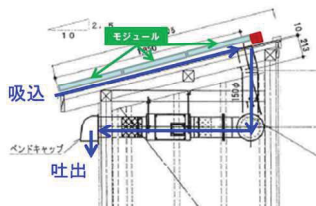
通風冷却方式
