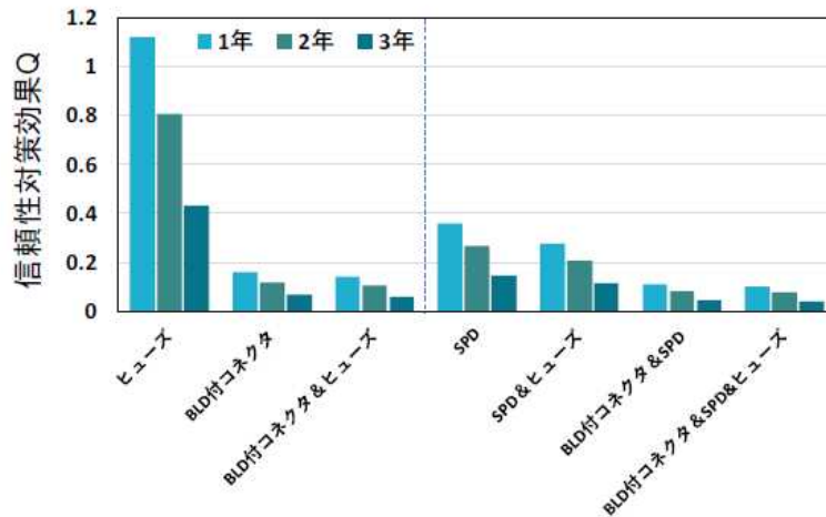
図Ⅲ-2-④-(1)-3 信頼性対策効果Q (1年, 2年, 3年運用時)
