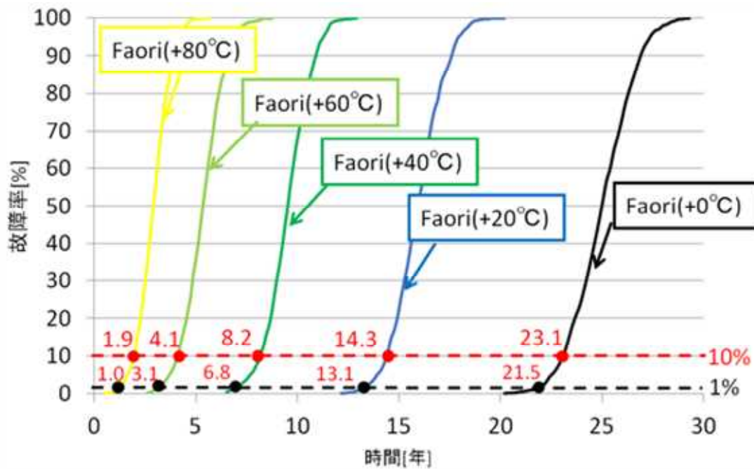
図Ⅲ-2-①-(1)-27 電解コンデンサ使用システムの寿命計算結果
