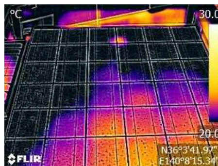
【バイパスダイオード／発熱後】
