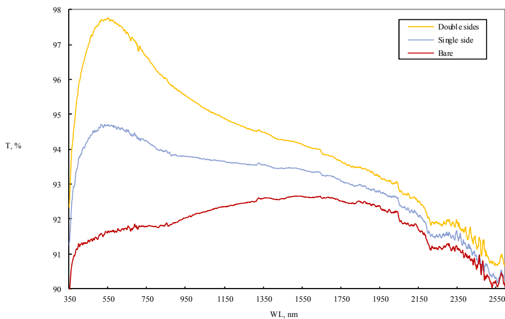
図 III-2-②-(4)-10 コートガラスの透過率
