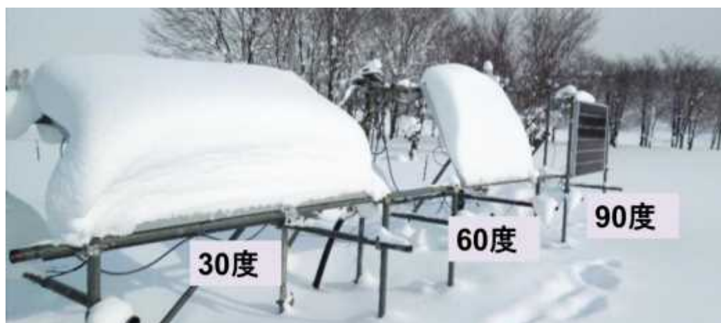
図Ⅲ-2-①-(2)-17 北海道深川市実証実験 (2016年1月16日13時 気温-8度)
