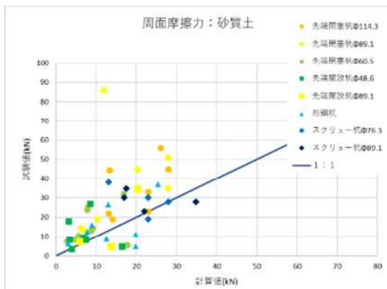
図III-2-④-(3)-8 周面摩擦力の計算値と試験値の関係(砂質土)
