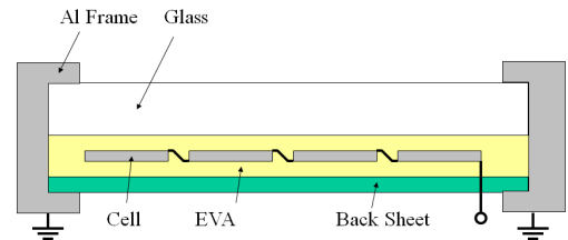
図 III-2-②-(4)-1 一般的な太陽電池の断面
