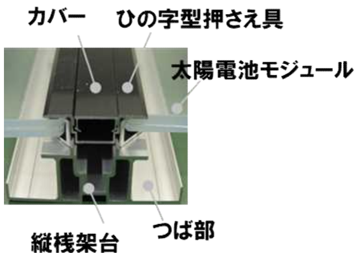
図Ⅲ-2-①-(6)-3 縦棧架台
