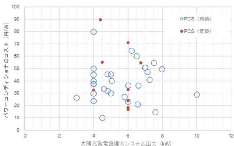
図Ⅲ-2-③-(1)-2 住宅用システムにおけるパワーコンディショナ(PCS)のコスト分布（新築、既築）
