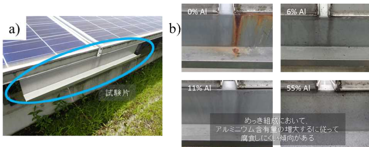
図III-2-①-(5)-11 a) 水みち腐食 試験片と b)各試験片の外観観察結果
