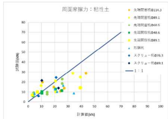
図III-2-④-(3)-9 周面摩擦力の計算値と試験値の関係(粘性土)
