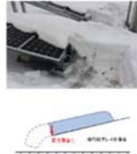
②軒先荷重の作用形態
