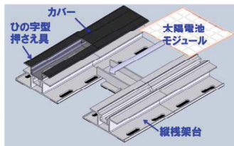
開発した設置工法
