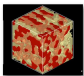
実電極 X線CT像
