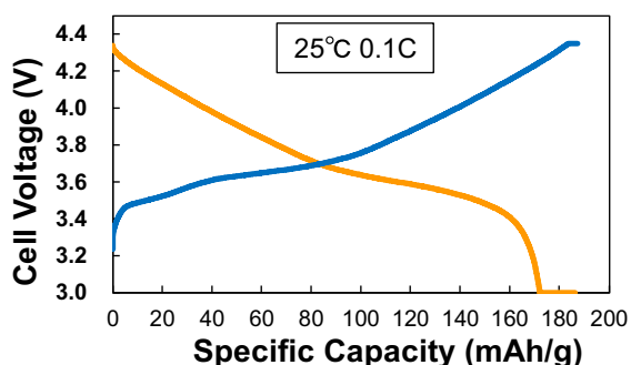
充放電特性
