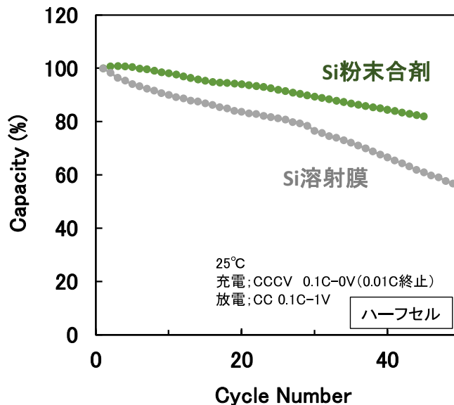
Si系活物質のサイクル耐性評価
