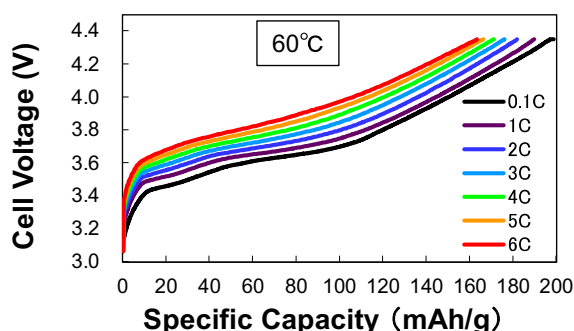
充電レート特性
