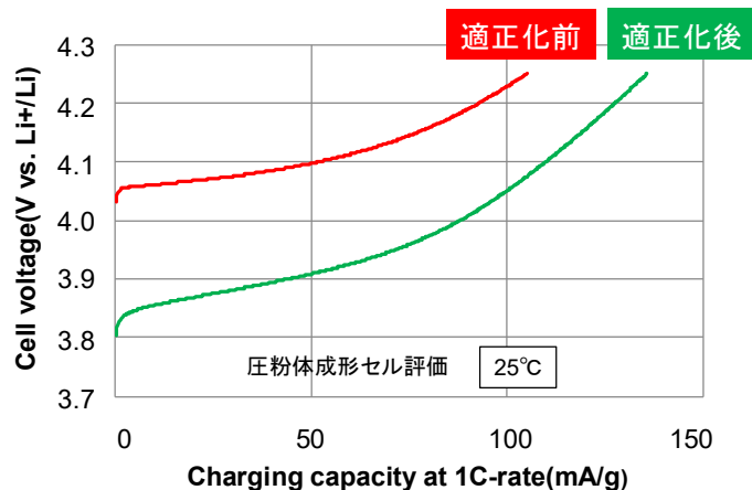
図 3.1.1-7 プロセス条件の異なる圧粉体成形 In-Li ハーフセルの充電容量試験結果
