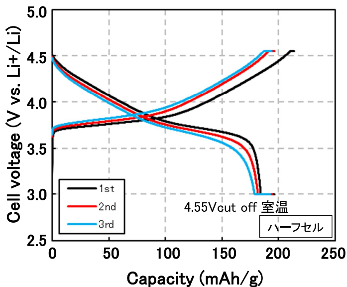
LiNbO 3 被覆三元系正極の中電位化
