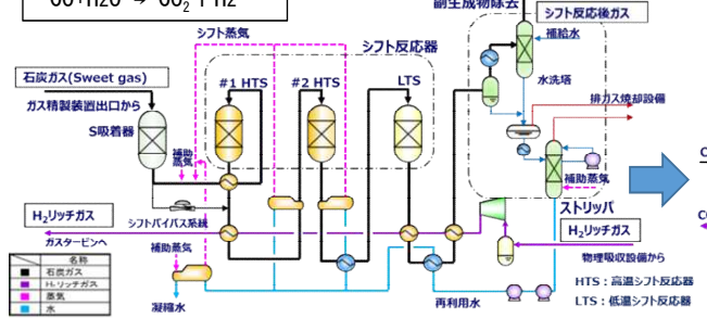
COシフト系統 プロセスフロー図
