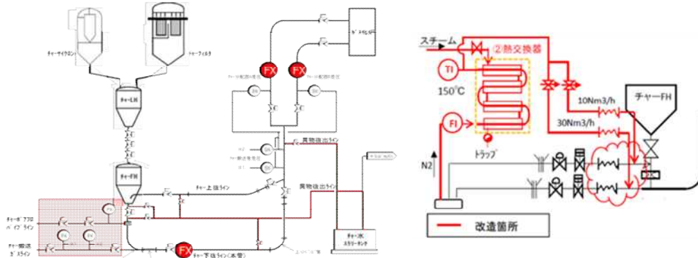
図 3-40 チャー供給・異物取出系統
