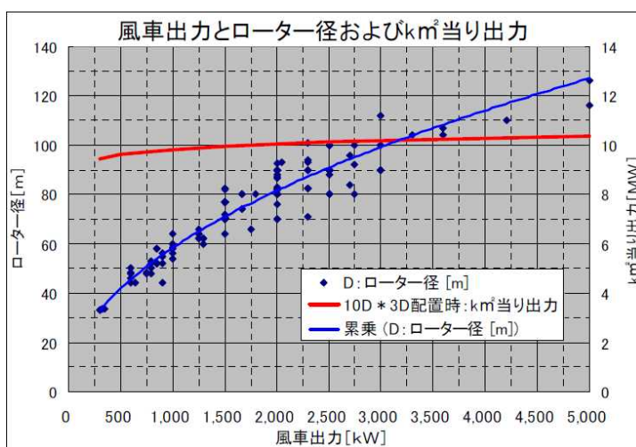
図 3-1-6 風車出力とローター系および 100×3D 配置時の 1km 2 当たり出力値
