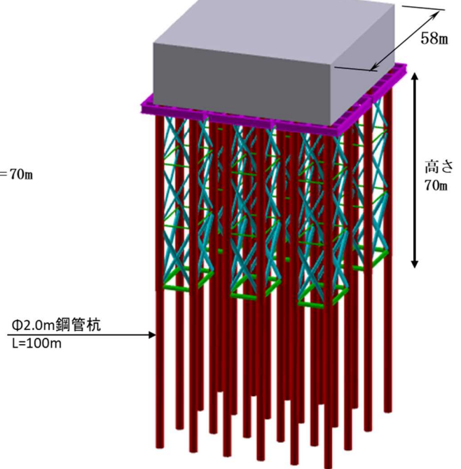
図 3-6-79 鋼製サクシヨン基礎、鋼製ジャケツト基礎鳥観図 (水深 50m)
