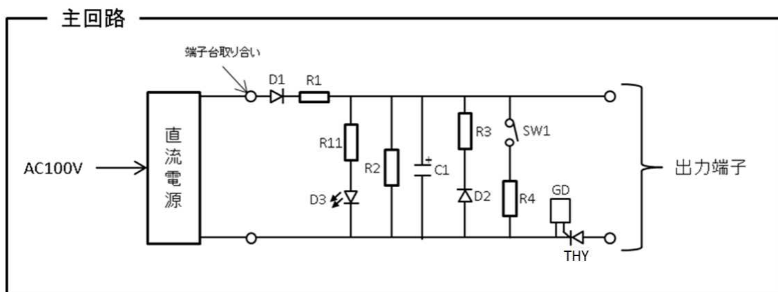
図 3-4-41 開路用・閉路用の制御主回路図
