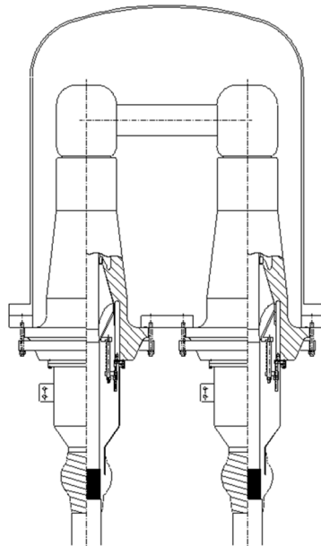
図 3-5-16 ガス終端接続箱 (EB-G) の概略図
