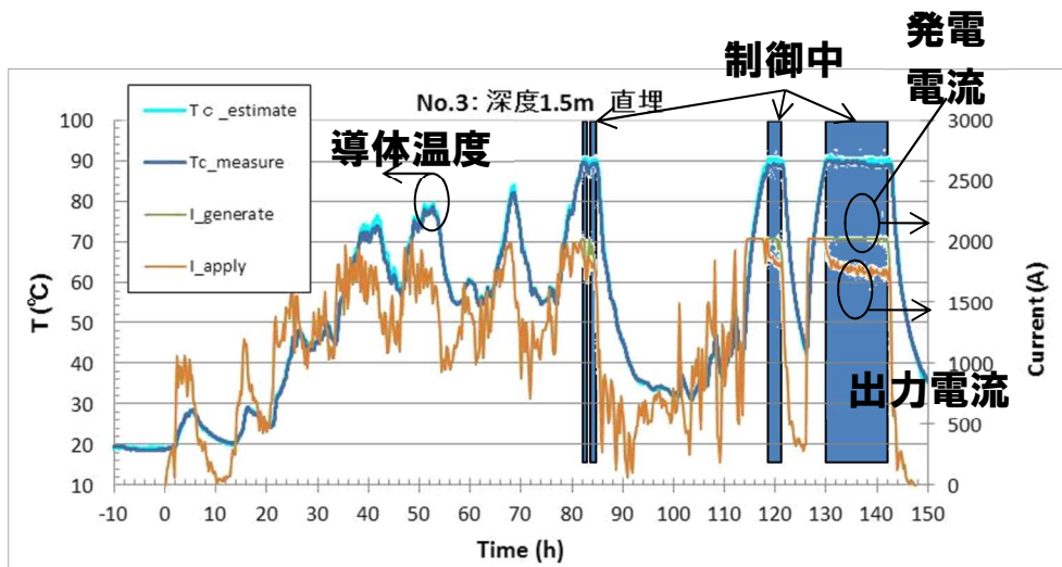
図 3-5-9 ダイナミックレイトィング制御例—風車模擬電流
