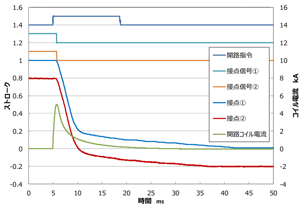
図 3-4-160 操作試験結果 (開路動作)
