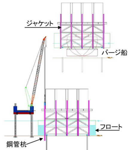
図 3-6-53 施工フロー
