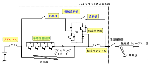
図3-6 ハイブリッド直流遮断器の構成
