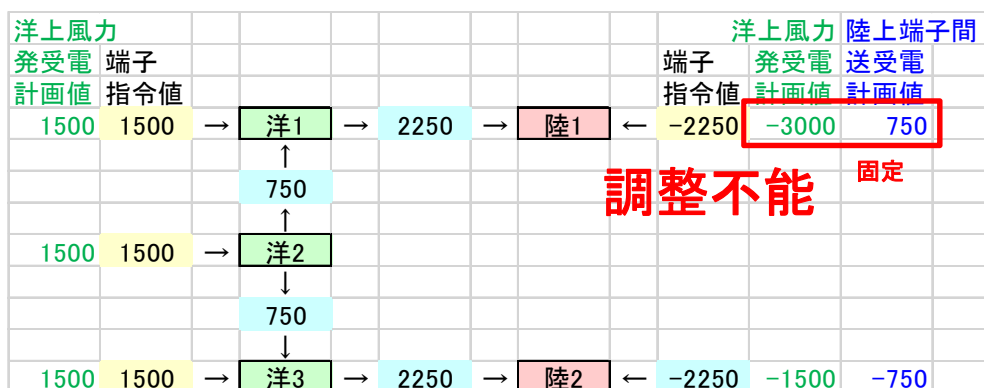
図7.24 パターン5：洋上風力発電計画および洋上風力受電計画（端子1）優先
