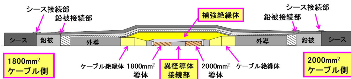
図 3-5-10 異径ケーブルの工場接続部断面図
