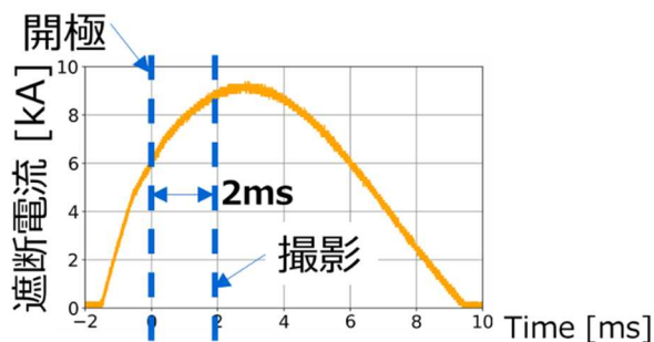
図 3-4-157 試験波形
