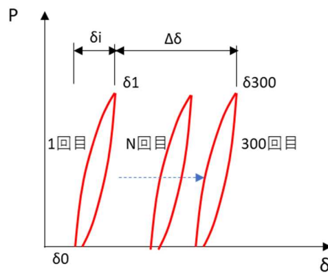
図 3-6-61 繰り返し载荷中の変位量
