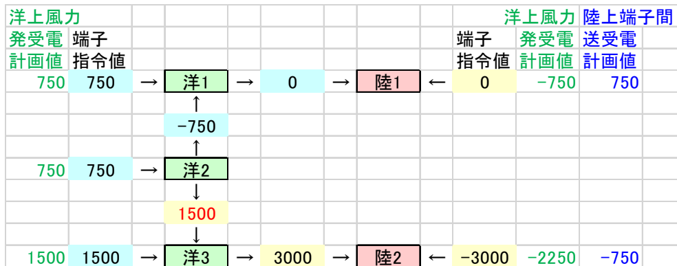
図7.23 パターン3：洋上風力発電計画および陸上端子間送受電計画優先（均等抑制）
