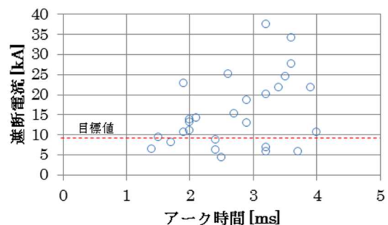
図 3-4-33 遮断試験結果
