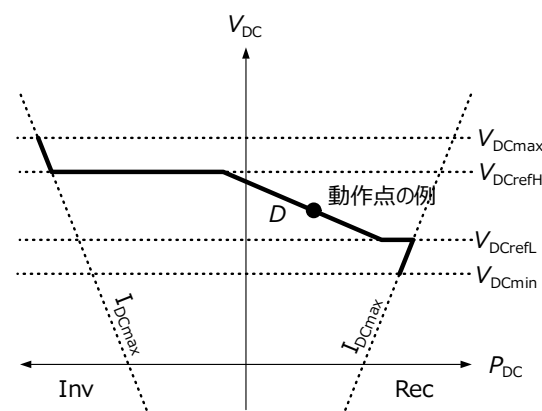
図4.3.6 緊急時直流電圧一定制御
