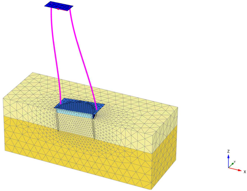
図 3-6-32 変形図 (case2) d=0.50m
