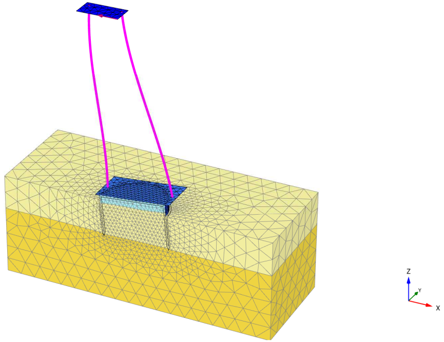
図 3-6-34 変形図 (case3) d=0.53\text{m}
