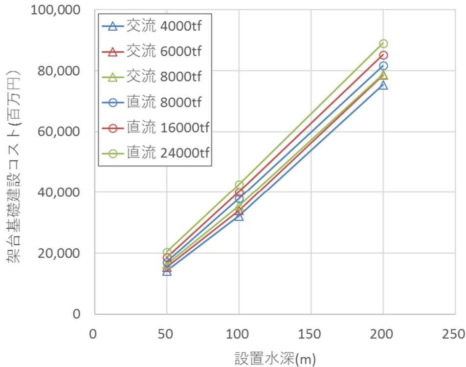
図 3-6-47 設置水深一建設コスト（交流および直流）
