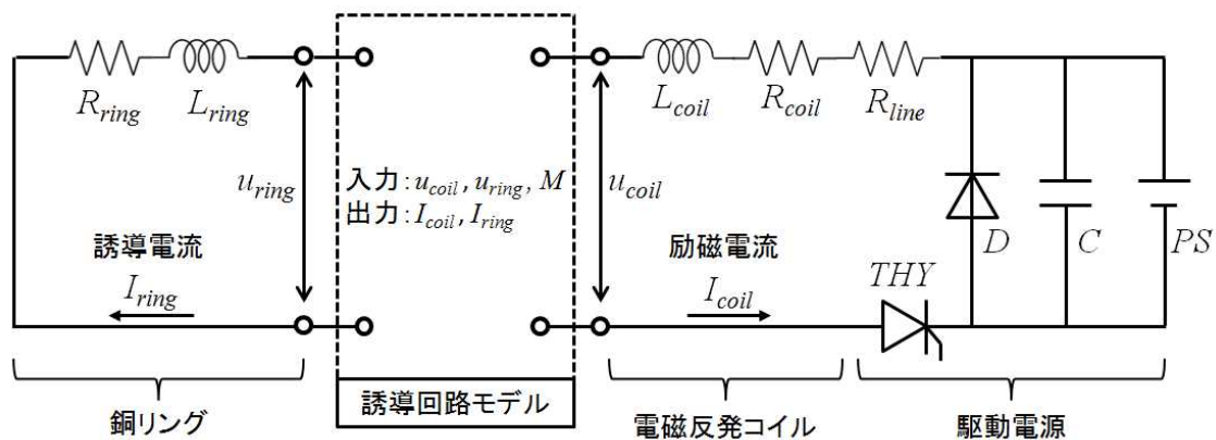
図 3-4-49 電磁反発部の電気回路モデル
