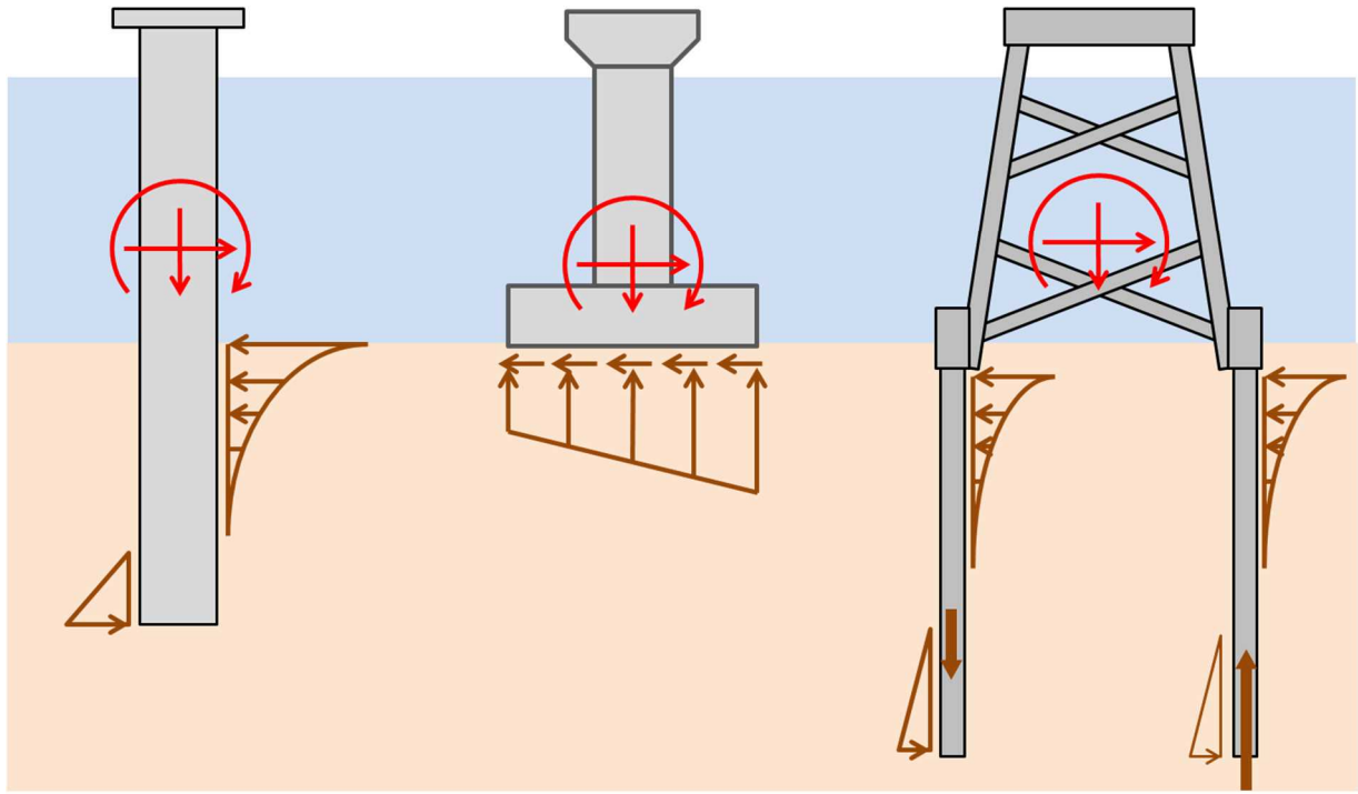
モノパイル
