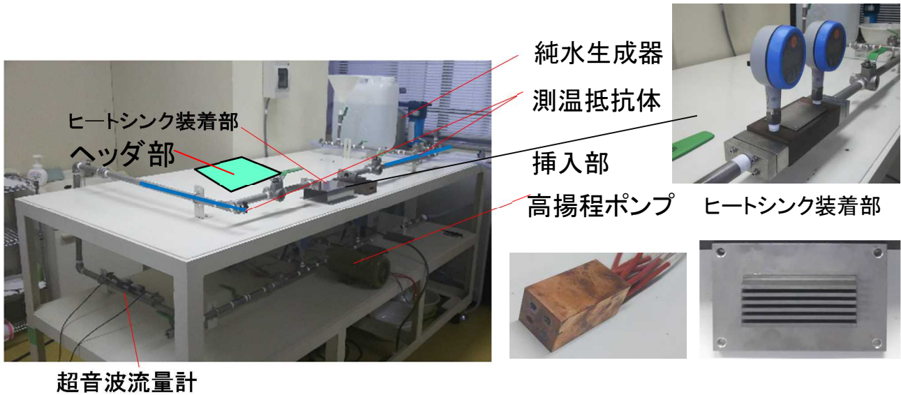
図 3-7-8 純水循環装置とヒータブロック及び楕形ヒートシンク
