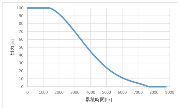
図 3-2-2 洋上 WF の想定出力-累積時間特性
