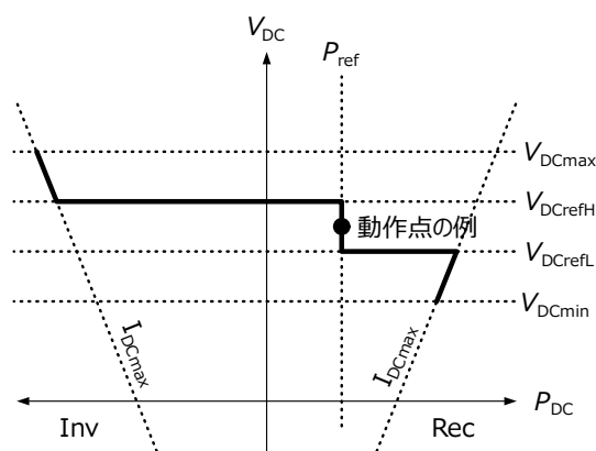
図4.3.4 2段AVR
