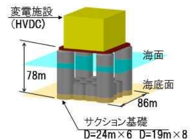
図3-9 概略設計例
