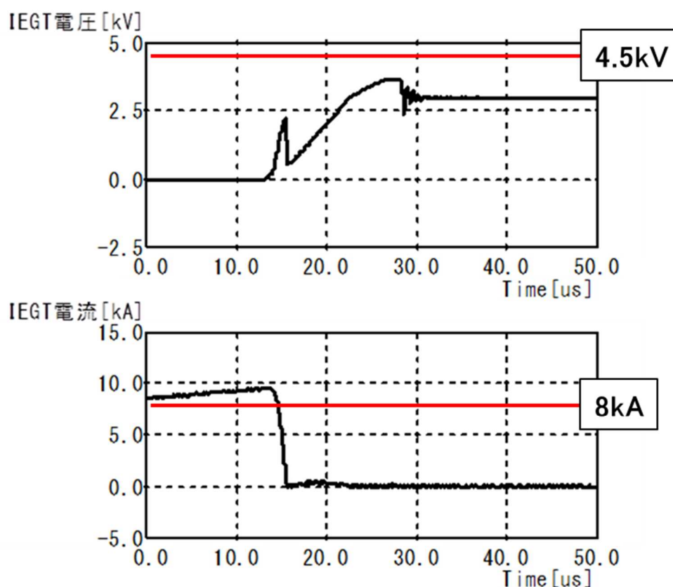
図 3-4-172 IEGT 単体遮断試験結果
