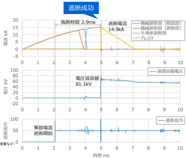
図3-7 遮断試験結果波形
