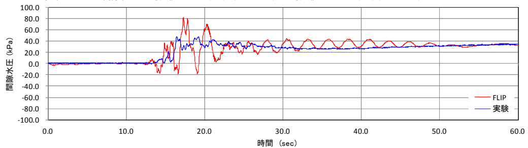
図 3-6-76 スカート内と地盤内の間隙水圧の時刻歴
