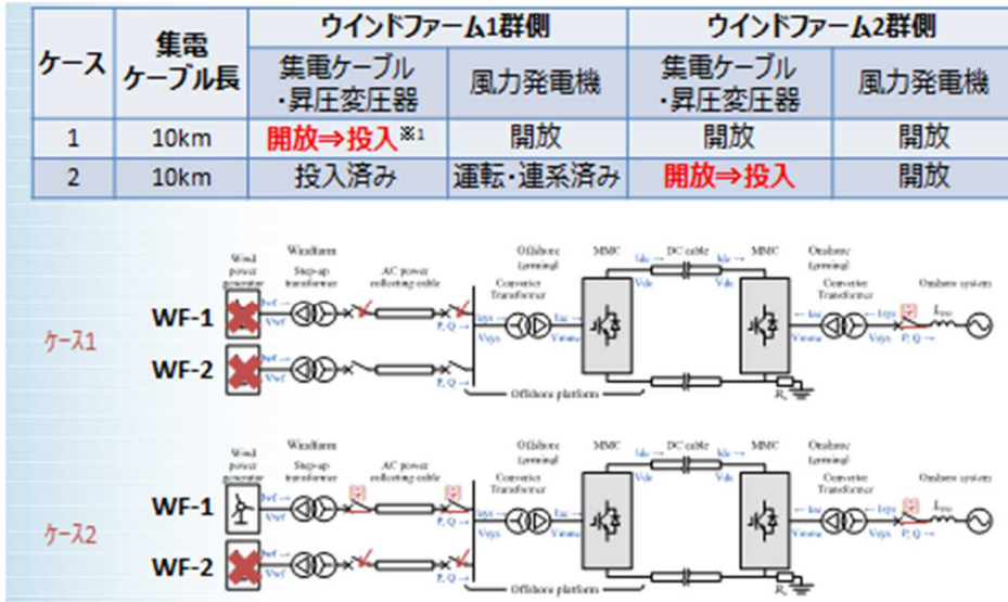
図 3-2-38 解析ケース
