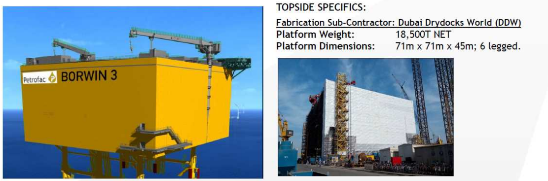
図 3-2-53 視察を実施した構築中 (2018 年 2 月時点) の洋上 PF
