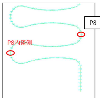
図 3-4-13 応力評価位置（固定側）
