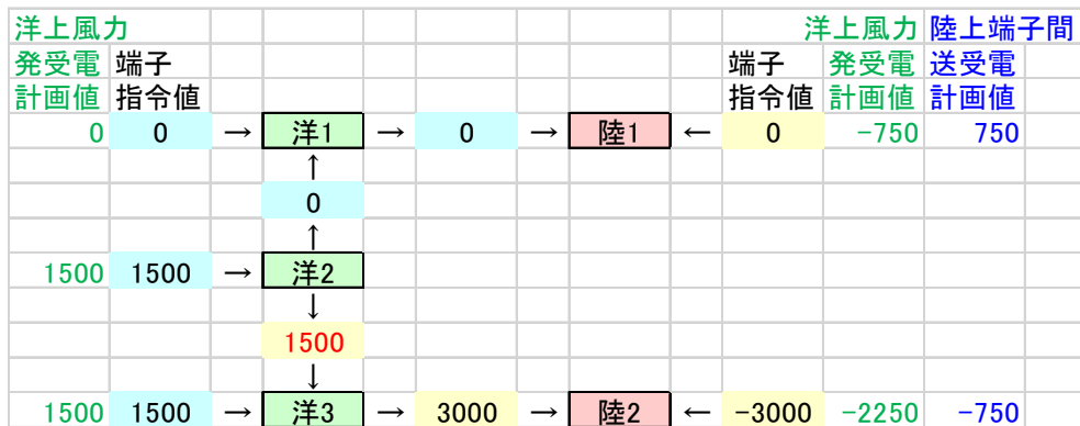
図7.22 パターン3：洋上風力発電計画および陸上端子間送受電計画優先（脱落設備近傍順抑制）
