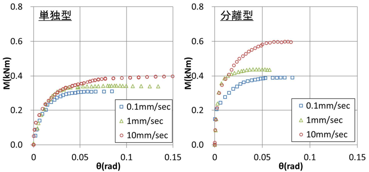
図 3-6-20 頂版位置での作用モーメントー回転角
