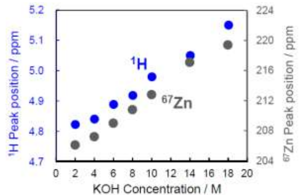
図 3.2-2-14 液中 KOH 濃度と NMR ピーク シフト
