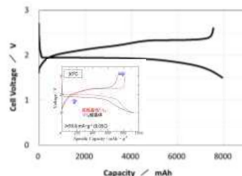
8Ah級試作セル
