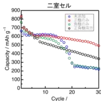
各電極へのLiDFOB添加効果
