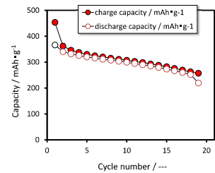
銅正極の容量維持率
