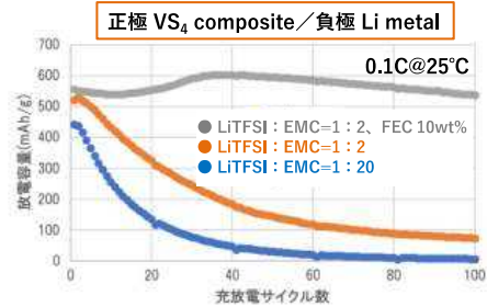
電解液種類とサイクル特性
