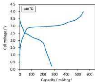
試作コイン形セル
