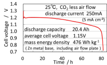
実セルの放電特性
