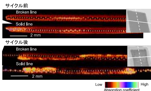
亜鉛電極断面のX線CT像
