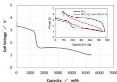
6Ah級試作セル
