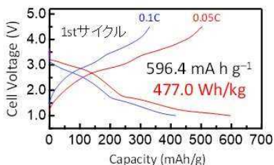
実セルの充放電特性
