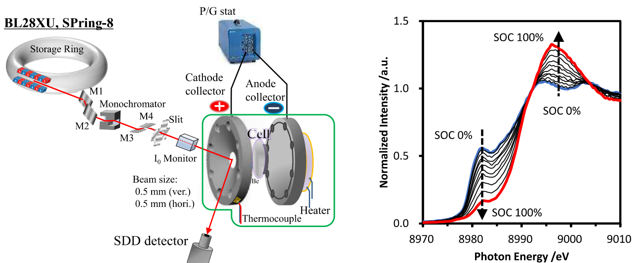
フッ化物電池のOperand解析装置概念図 (SPRING8/BL28)
