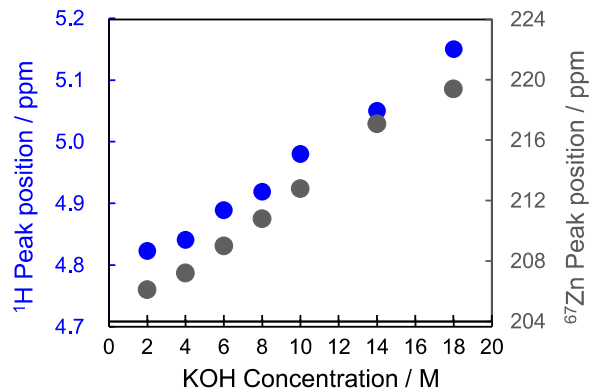
液中KOH濃度とNMRピークシフト
