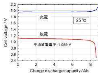
8Ah試作セル
