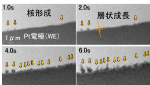
Pt電極上での亜鉛析出状態観察
