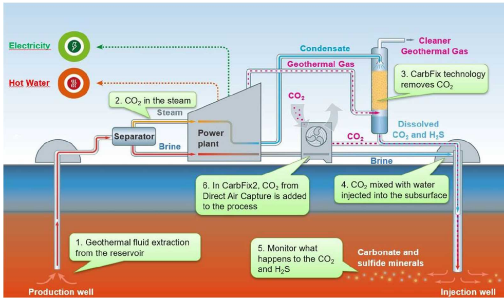
アイスランドでの試験の概念図 https://www.or.is/sites/or.is/files/pressfactsheet.pdf
