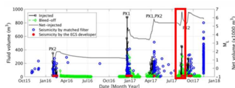
Pohangサイトでの水圧破砕履歴 (Kim et al. 2018)
