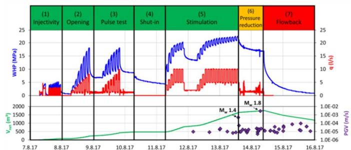
韓国Pohangでの水圧破砕実験結果 (Hofmann et al. 2018)。Cyclic stimulationを行うことにより, 誘発微小地震数, マグニチュードを抑制することに成功した。
