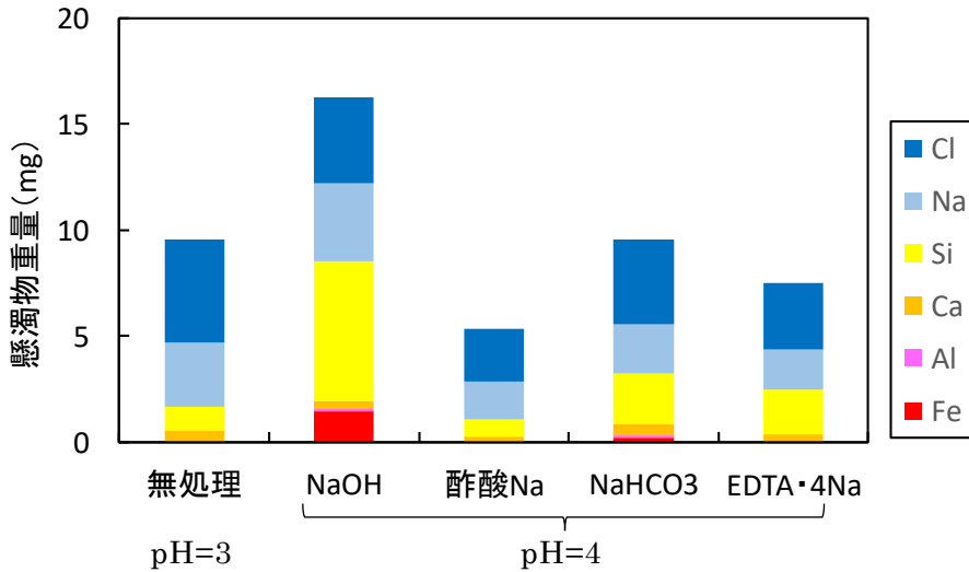
図Ⅲ-2 酸性熱水を各薬剤で中和処理した後のスケールの重量と化学組成
