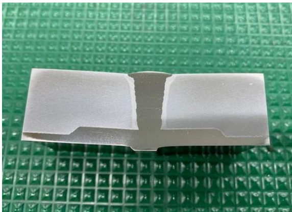
【溶接部断面】
