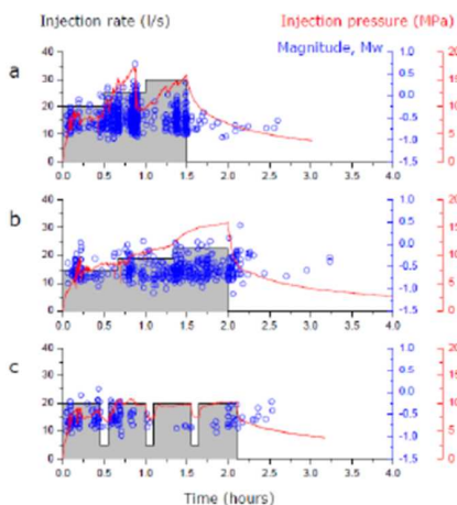
水圧破砕シミュレーション結果の例 (Farkas et al. 2018)。Cyclic stimulation (c)では誘発地震の発生数が少ないことがわかる。
