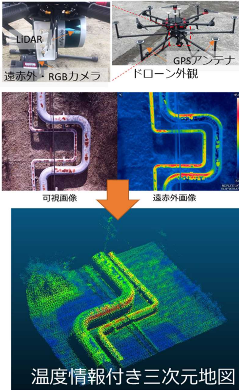
ドローンによる配管点検
