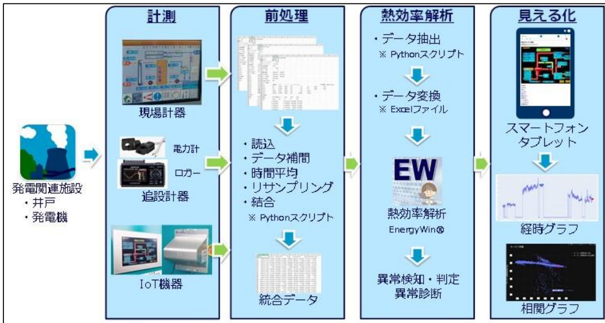
図Ⅲ-6 運転管理支援ツール(管理ツール)の概略図
