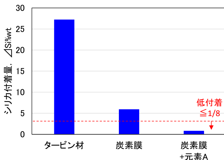
図Ⅲ-9 各材料におけるシリカ付着量
