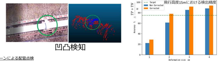
ドローンによる配管点検
