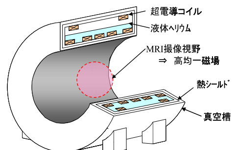
図2: MRI用超電導マグネット構成図 (現行機: 液体ヘリウム使用)
