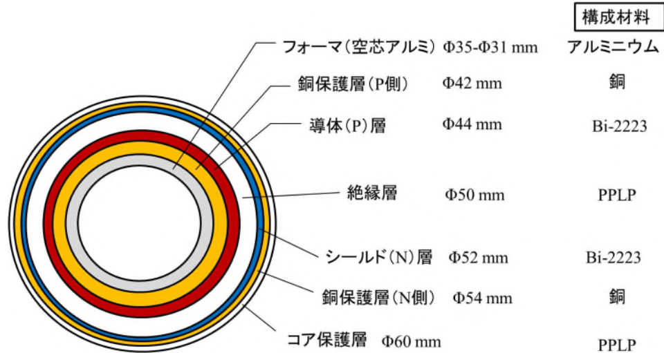
図 2.1.4-6 10 kA 級超電導ケーブルの解析モデル
