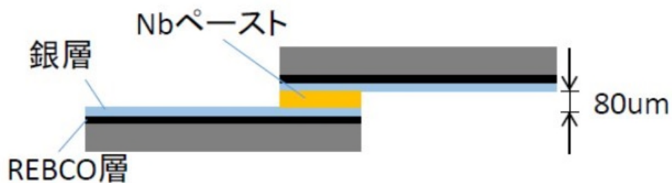
図 2.3.2-19 REBCO 高温超電導の対向接続模式図
