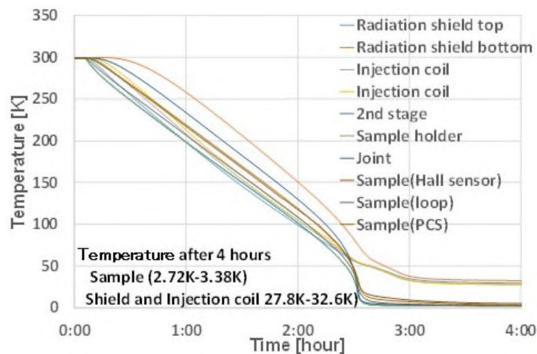
図 2.3.5-9* 室温からの初期冷却曲線
