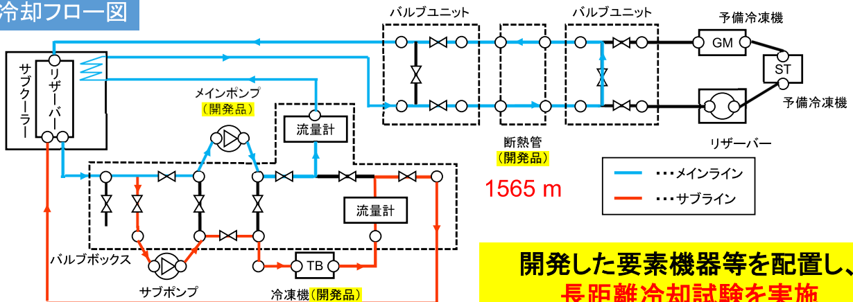
冷却システム(建屋内)
