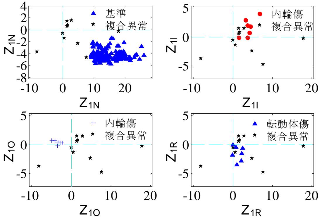
図 2.1.6-16 複合異常診断の例
