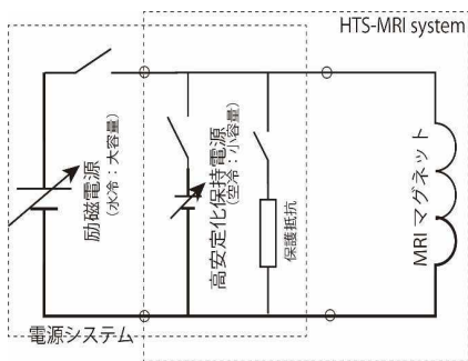
MRI用 省電力高安定励磁電源システム
