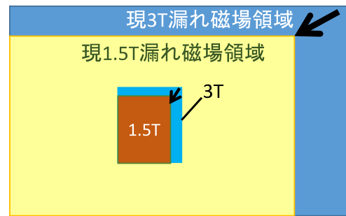
MRIマグネットの漏れ磁場、形状の概要 (HTS-3Tが現1.5T並みに)
