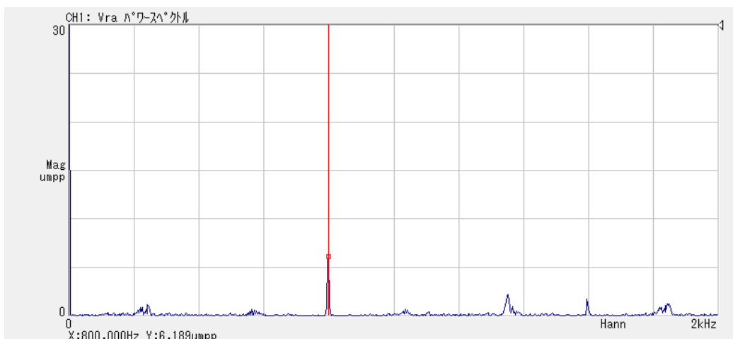
図 2.1.2-9 定格回転数（48,000rpm）におけるラジアル方向振動パワースペクトル
