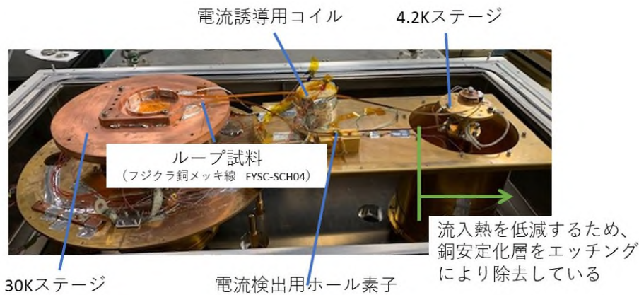
図 2.3.6-29 永久電流実証用ループ試料を取り付けた接続アシスト環境疑似モデル
