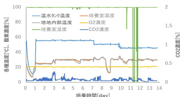
図 3.2.1.1.3.4-6 培養試験中の温度・湿度等の計測データ
