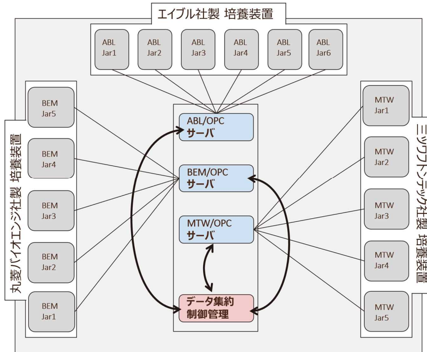
図 3.2.1.1.4.1-6 一元管理 PC による各社の培養槽との連携模式図
