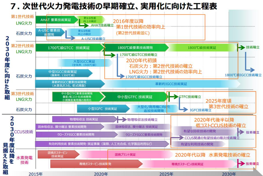
図1-5 カーボンリサイクル技術の実用化工程表
