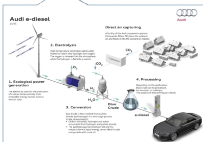
図2 アウディ社ラウフェンブルグのe-dieselプラント (イメージ)
