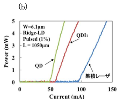
図 1.2.1.1(イ)-8 1250 nm 帯量子ドット及び 2 種組成混合導波路集積レーザ特性 : (a) 素子断面模式図 (b)各領域と集積構造レーザの I-L 特性
