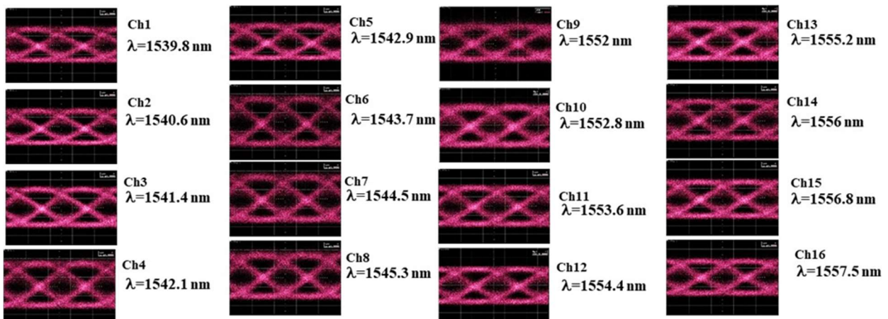
図 1.2.2.1(ア)-17 50 Gbps NRZ 変調信号の伝送特性
