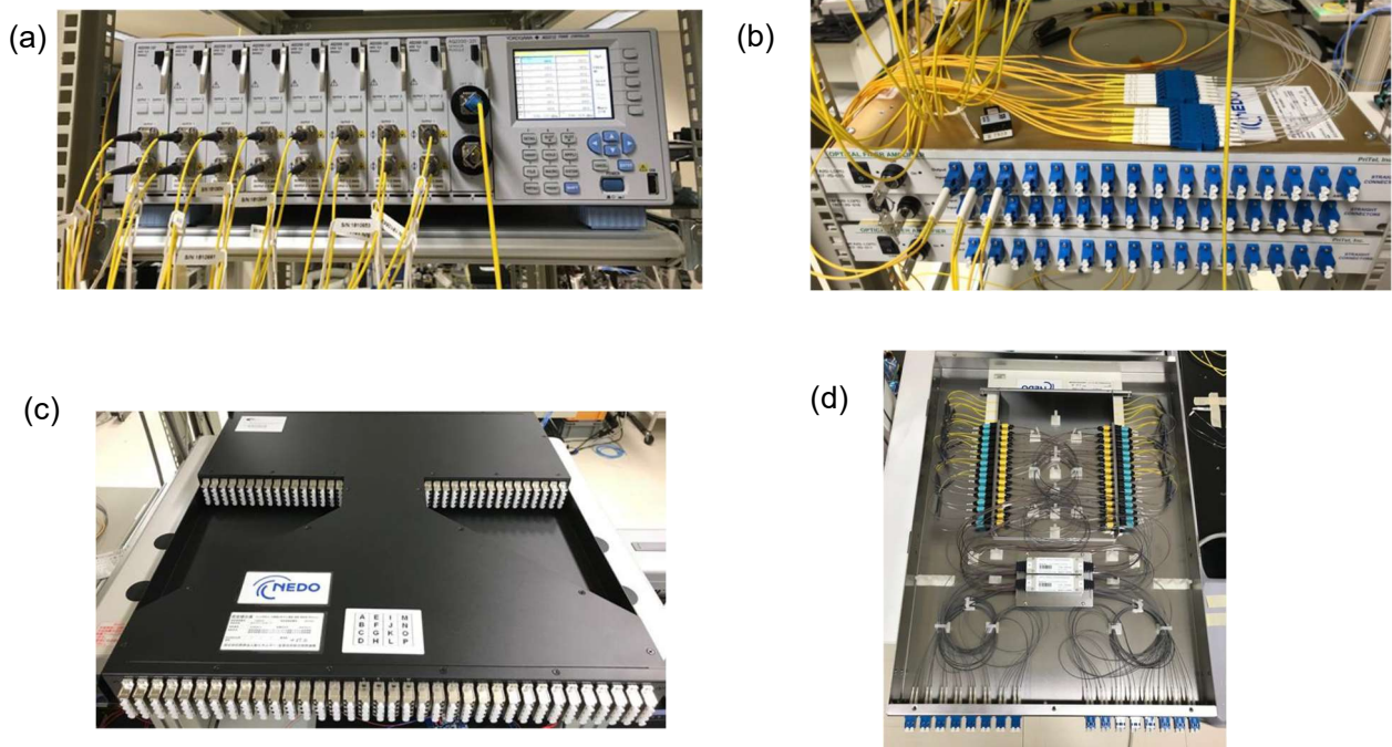
図 1.2.2.2(エ)②-34 波長多重ネットワークの主要構成部品の外観写真、(a)多波長光源、(b)EDFA 光アンプ、(c)光スプリッタボード、(d)波長ルータ・ボード
