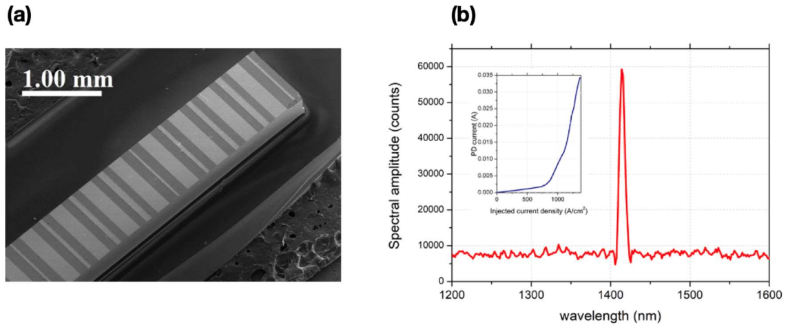
図 1.2.1.1(ア)-8 (a) シリコン基板に融着された長波長帯量子ドットレーザ (b) シリコン基板上長波長帯量子ドットレーザからのレーザ発振
