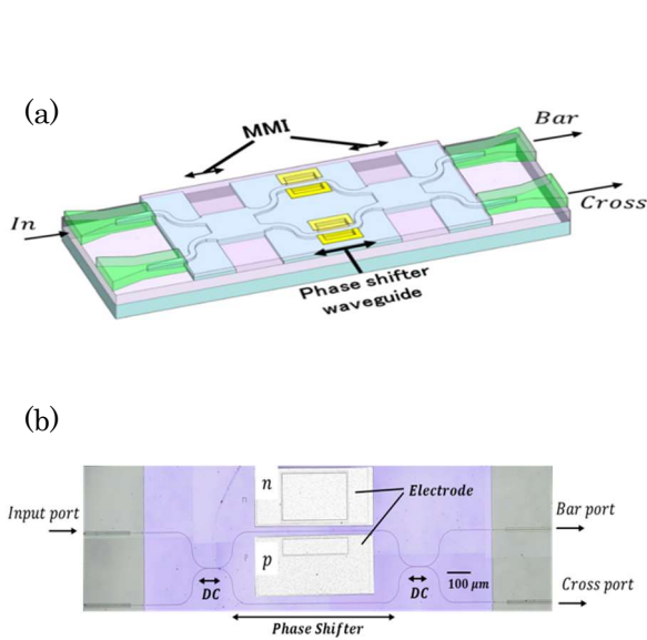
図 1.2.1.1(イ)-1 シリコン偏光無依存高速マッハツェンダ型光スイッチ： (a)素子構造模式図、(b)素子表面写真
