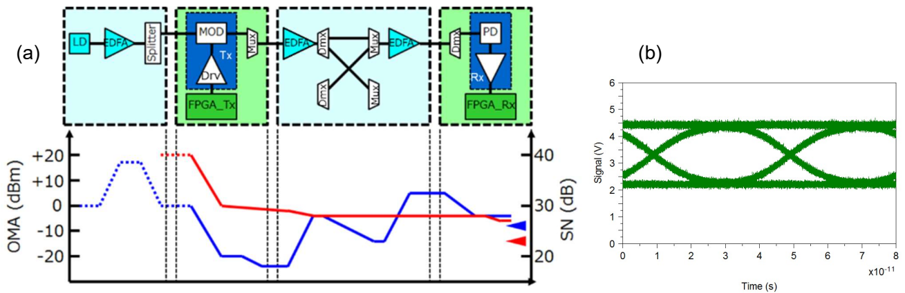
図 1.2.2.2(エ)②-4 ノード間波長多重ネットワークのリンク設計、(a)レベルダイアグラム、(b)25Gb/s 受信波のシミュレーション
