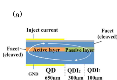
図 1.2.1.1(イ)-8 1250 nm 帯量子ドット及び 2 種組成混合導波路集積レーザ特性 : (a) 素子断面模式図 (b)各領域と集積構造レーザの I-L 特性
