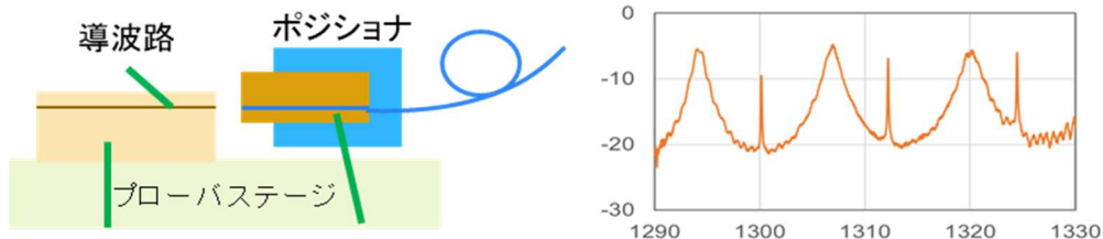
図 1.2.2.1(イ)-21 プローバを用いた端面光結合によるチップ特性評価のための構成図(左)、及びリング共振器のドロップポートスペクトル観測例(右)
