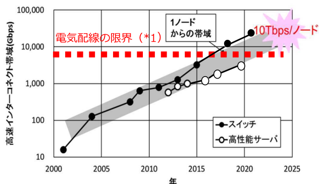
大容量LSIのインターコネクタ帯域トレンド
