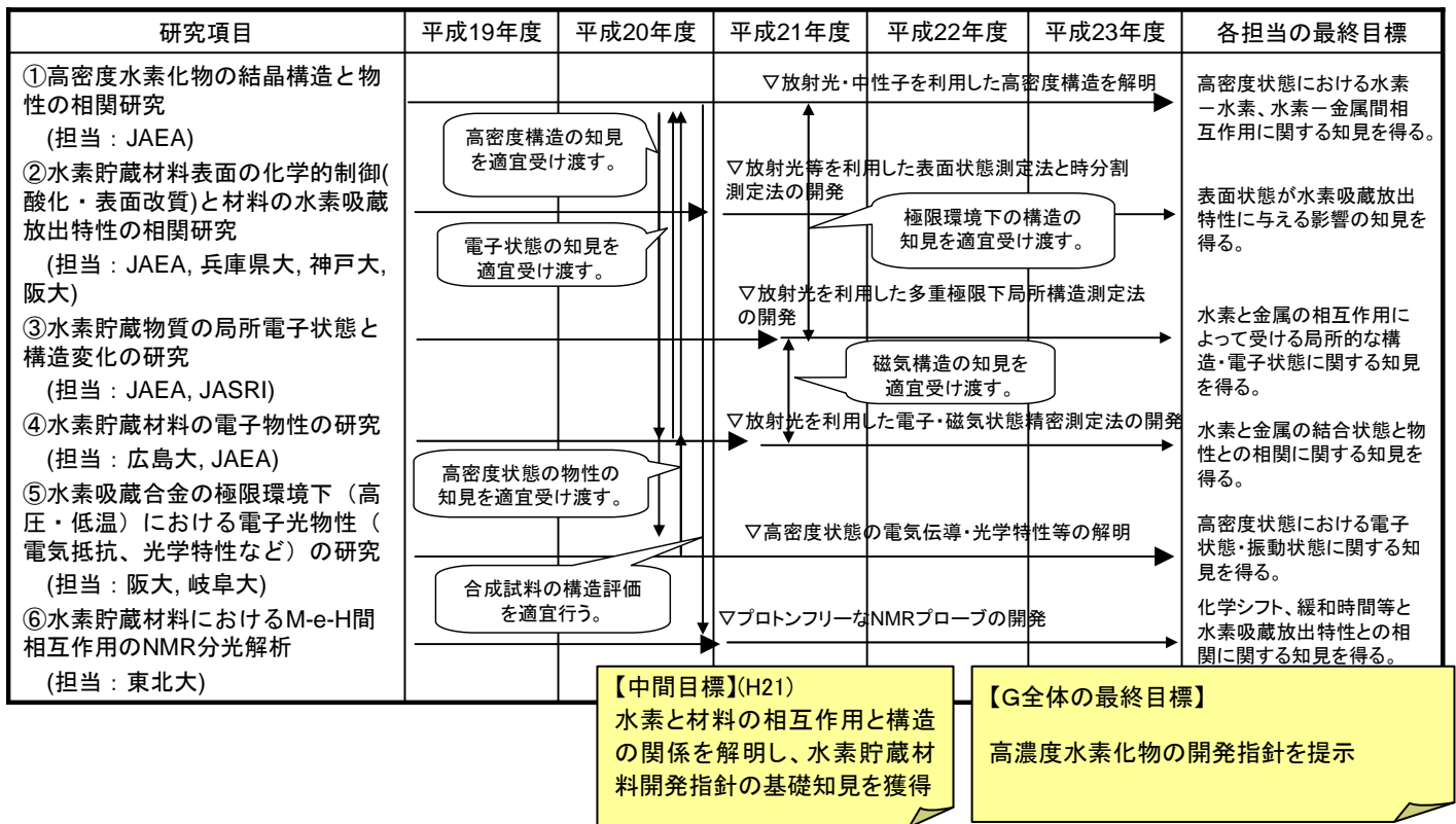
図 II-(5) ③「水素と材料の相互作用の実験的解明」の研究開発計画」
