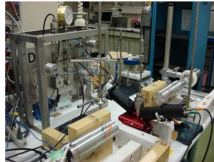
図IV1.1.3-(3) 高圧水素雰囲気中での陽電子消滅実験装置
