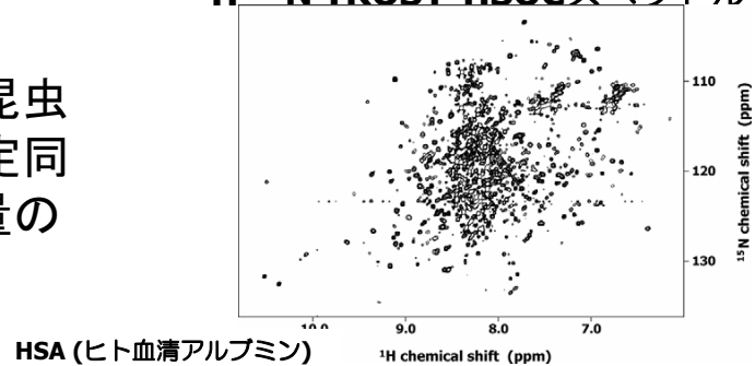
完全重水素化を施したHASの 1 H- 15 N TROSY-HSQCスペクトル
