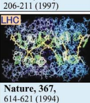
LHC Nature, 367, 614-621 (1994)
