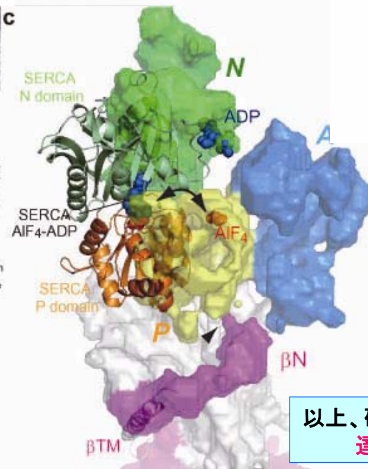
事業原簿 18ページ βサブユニットのラチェットモデル
