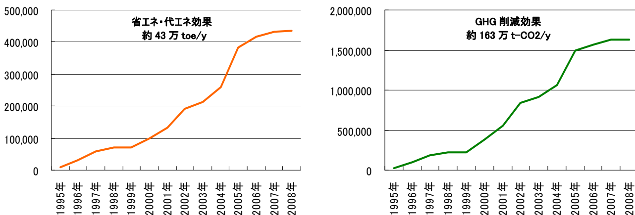
モデル事業設備（普及分は除く）による省エネ・代エネ効果目標値・GHG削減目標値（2009年までの累積値）
