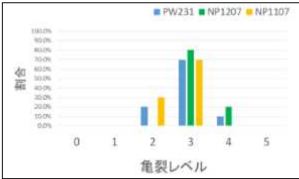
図III-2-①-(1)-24 INV基板 (糸半田) _2000cyc
