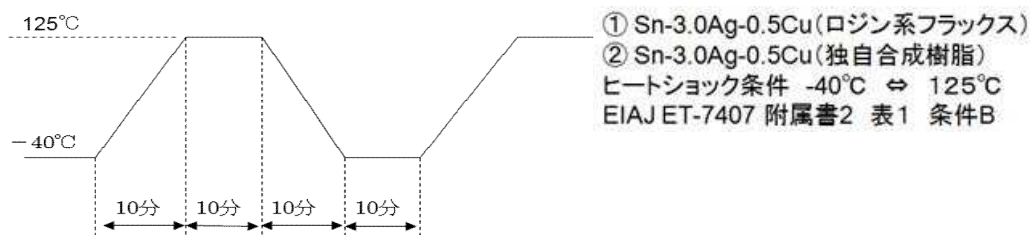
図Ⅲ-2-①-(2)-27 金属配線基板のヒートサイクル試験実施条件
