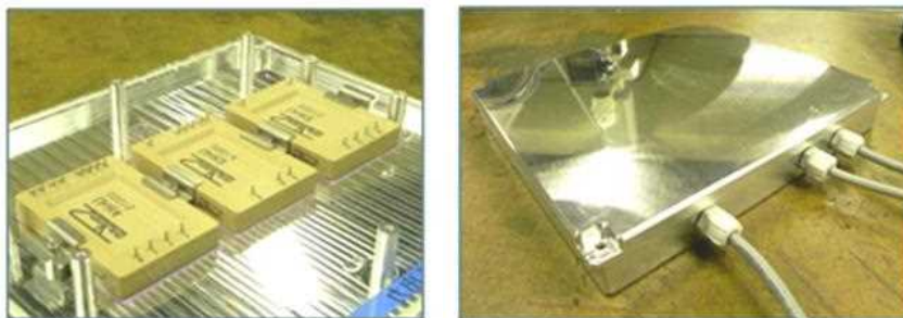
図Ⅲ-2-①-(2)-30 筐体気密評価用試作ユニット
