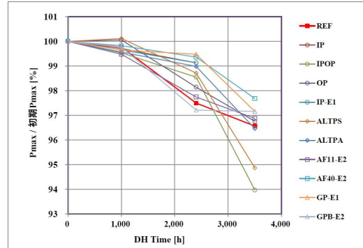
図 Ⅲ-2-①-(5)-7 DH 時間と Pmax/初期 Pmax の変化
