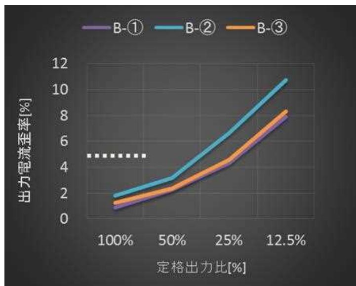
図Ⅲ-2-①-(1)-11 B-①～③の出力電流歪率特性
