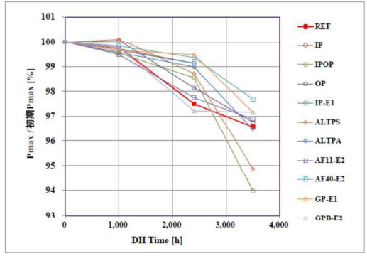
図 4.2-b) DH 時間と Pmax / 初期 Pmax の変化
