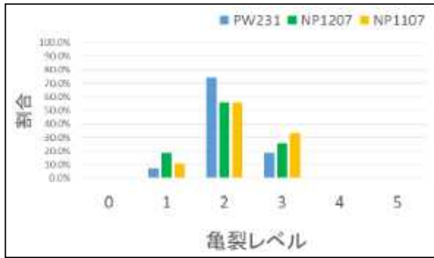
図III-2-①-(1)-25 CTL基板 (クリーム半田) _2000cyc
