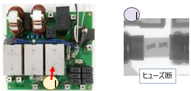
図Ⅲ-2-①-(1)-15 AC 基板のヒューズ
