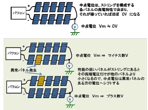
中点電位モニタリングのイメージ 34/51
