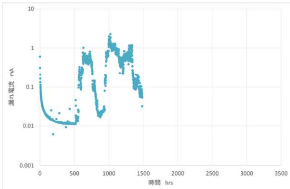
図Ⅲ-2-①-(1)-41 パターン C の漏れ電流推移
