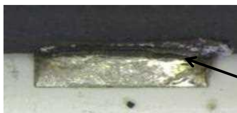
図Ⅲ-2-①-(2)-28 金属基板への大型面実装部品のヒートサイクル試験によるはんだクラックの発生
