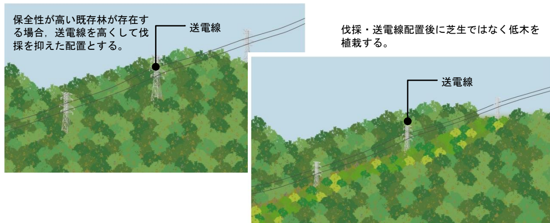
図 5.120 足元に緑のある送電線配置
