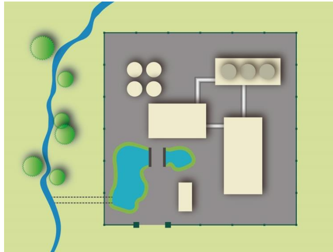
図 5.58 一時貯留池を含んだ配置計画
