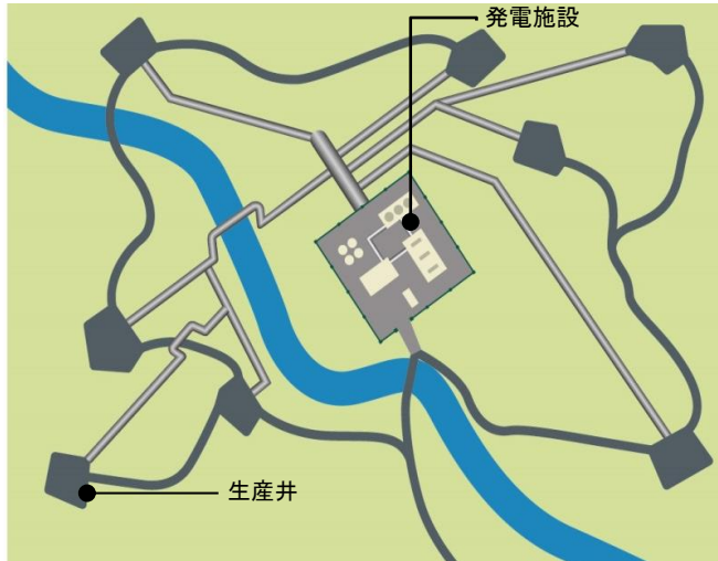
図 5.177 一般的な発電施設と生産・還元井計画
