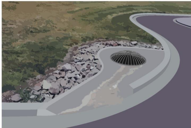
図 5.190 栗石を用いた側溝
