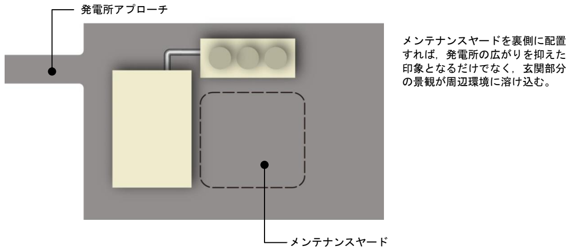
図 5.82 建屋の裏側に配置したメンテナンスヤード
