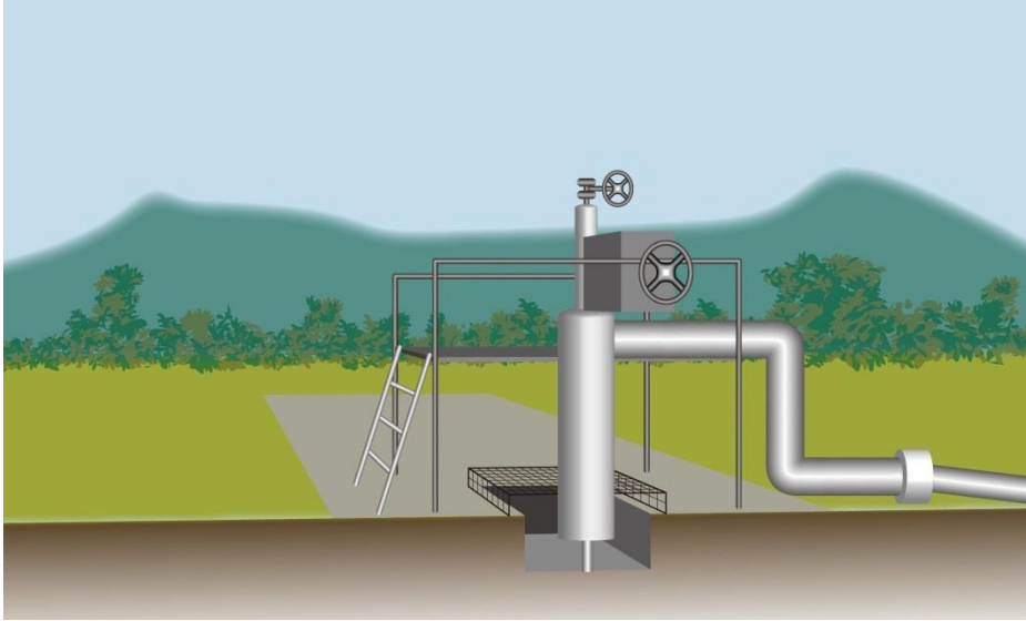
図 5.17 一般的な還元井の設置
