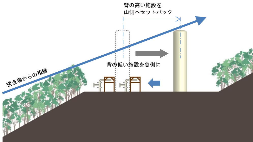
図 5.16 視線に配慮して背の高い施設を山側に配置した計画
