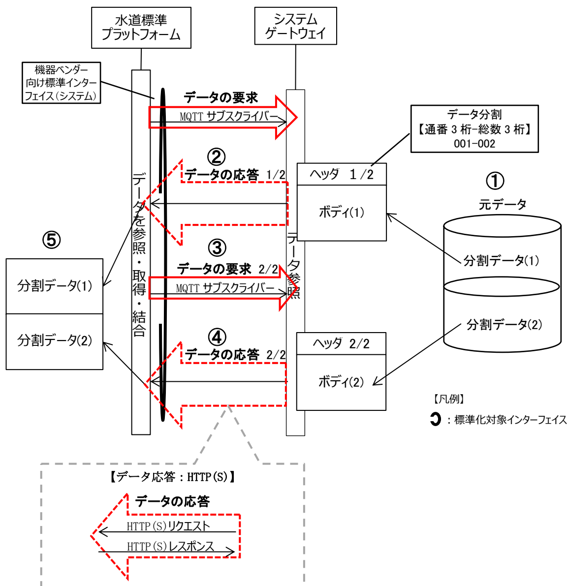
図 3-7: データの分割送信
