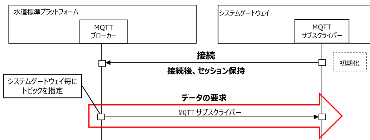
図 3-2: MQTT の接続シーケンス (要求データ取得)
