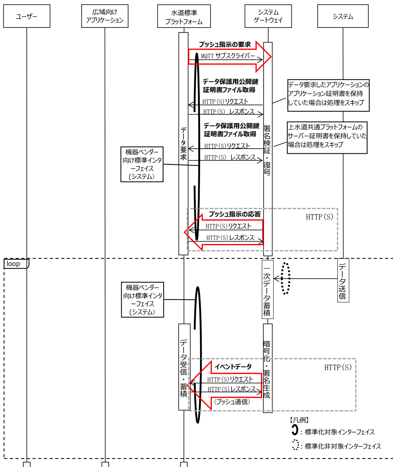
図 4-5: 定周期データ蓄積の接続シーケンス
