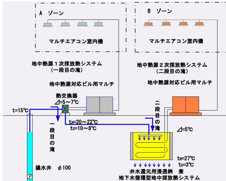
図IV(2.1)-1 Heat-Gw-Power CASCADE のイメージ図
