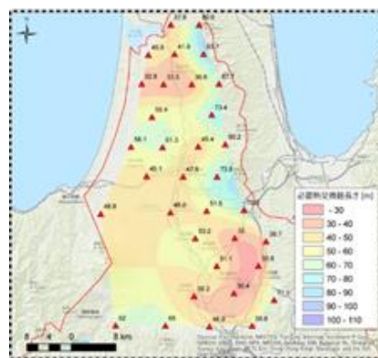
図Ⅲ(2.8)-2 ポテンシャルマップの一例 (クローズドループシステムにおける必要熱交換器長さの分布)
