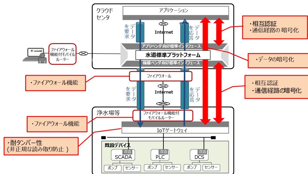
図7 セキュリティ対策の概要
