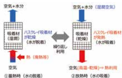
▲吸着材蓄熱の蓄熱・放熱の原理
