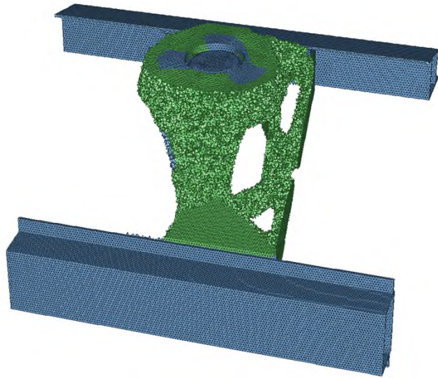
2材料の最適化： 鋼，アルミニウム
