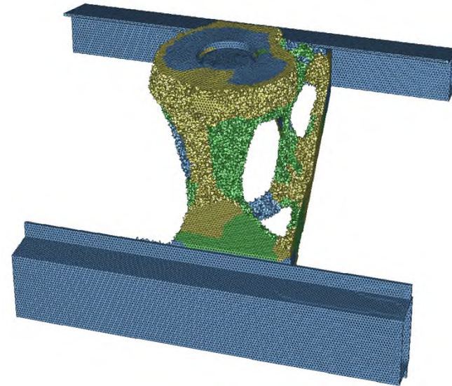
3材料の最適化： 鋼，アルミニウム，マグネシウム
