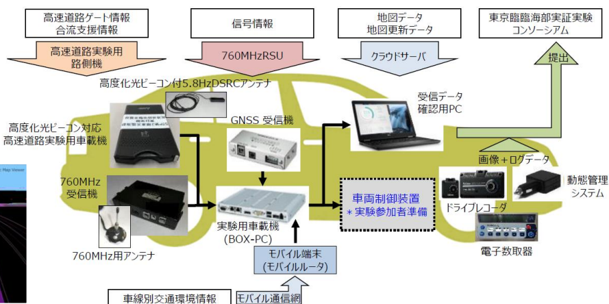
実証実験用車載器システム構成図
