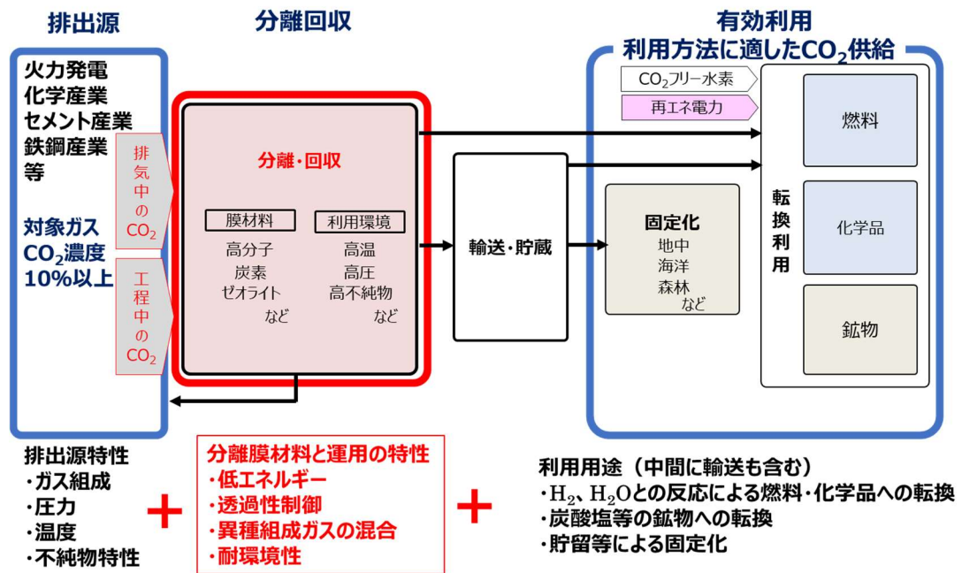
図1 排出源特性やCO 2 利用方法と連携したCO 2 膜分離システムの例示
