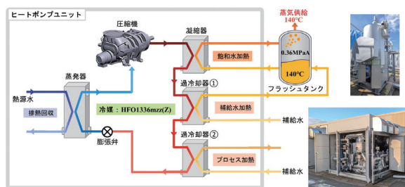
図：技術開発の事業化概念図と開発した超高効率スクロール式膨張機
