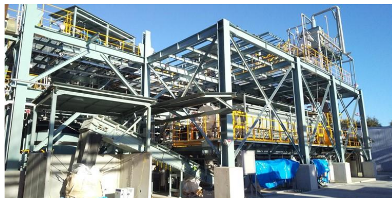
CO 2 有効利用設備
