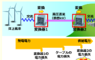
高圧直流送電用変換器の効果
