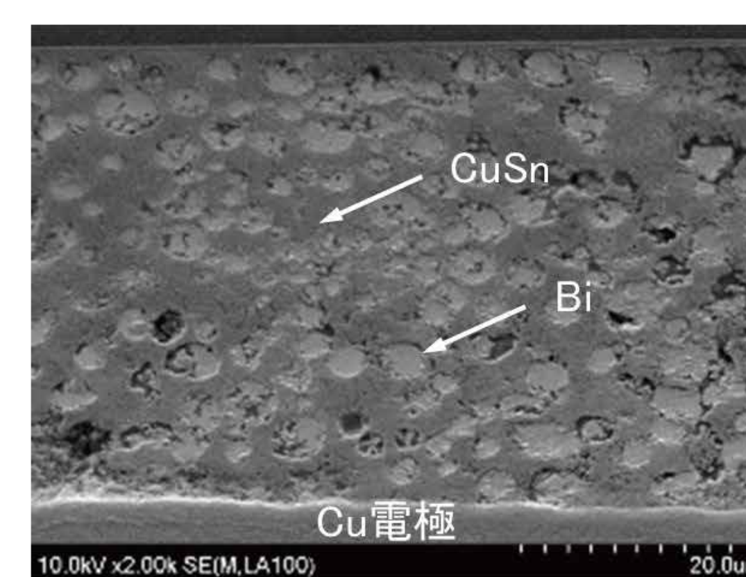
接合断面構造
