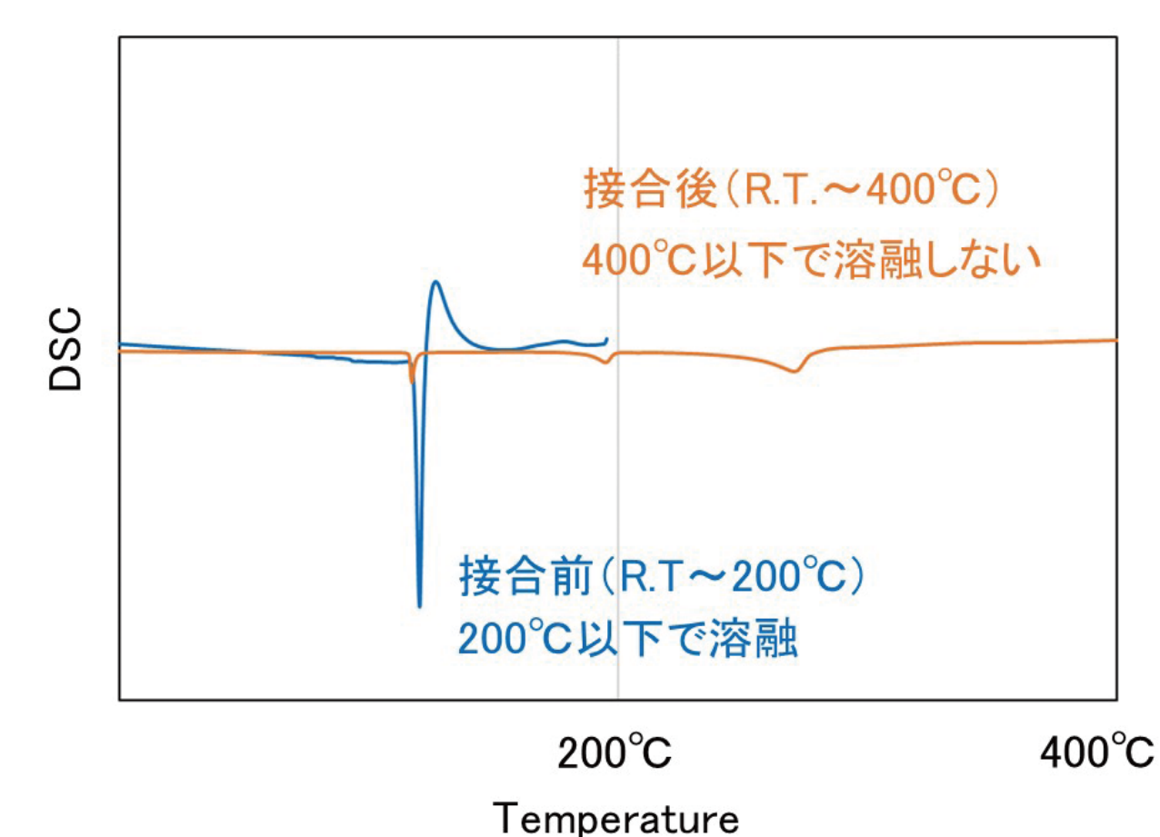
熱分析結果
