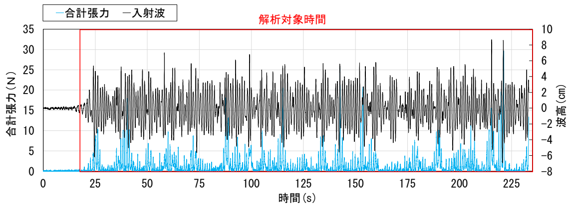
(b) 不規則波実験における張力の解析対象時間 (ケース名 : F6_10-085)
