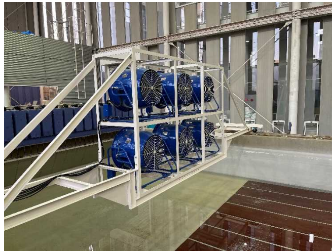
図 3-2 送風機
