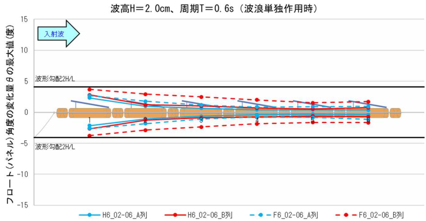
図 5-18 短周期のケースにおけるフロート(パネル)の傾斜角と波形勾配の比較(波高 2.0cm)
