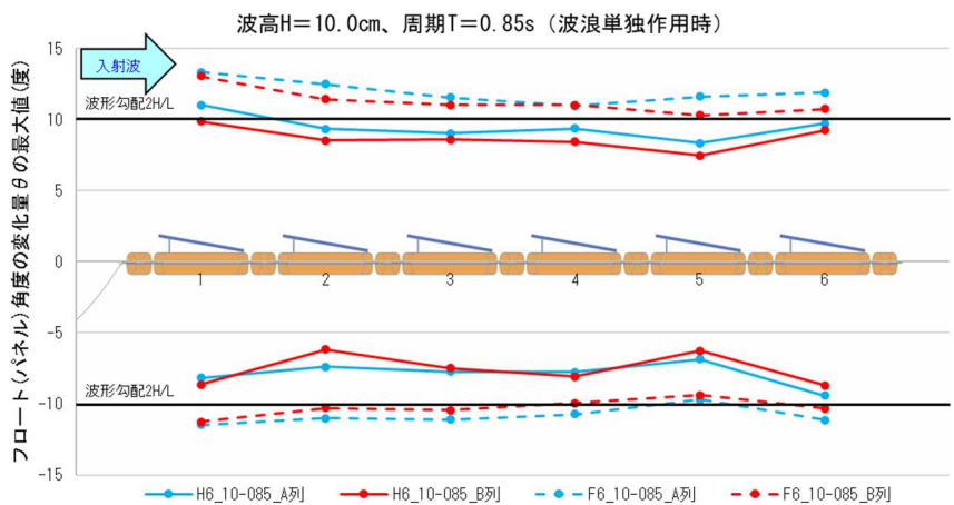
図 5-20 短周期のケースにおけるフロート(パネル)の傾斜角と波形勾配の比較(波高 10.0cm)
