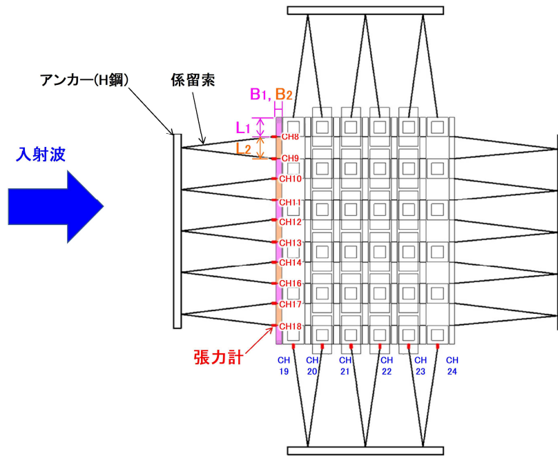
(a) 矩形アイランドでの波力算定方式の模式図 (平面図)
