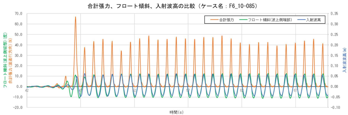
(a) 被災波相当波浪（F6_10-085）における合計張力、フロート傾斜、入射波高の比較結果（矩形アイランド）
