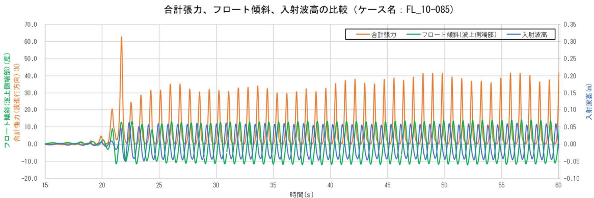
(b) 被災波相当波浪（FL_10-085）における合計張力、フロート傾斜、入射波高の比較結果（L字アイランド）
