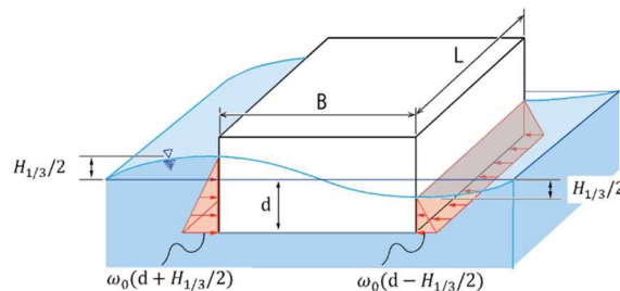
図5-2 浅喫水の小型浮体に対する波力算定式および模式図
