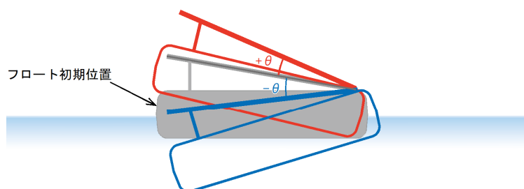
図 5-15 フロート（パネル）の傾斜角
