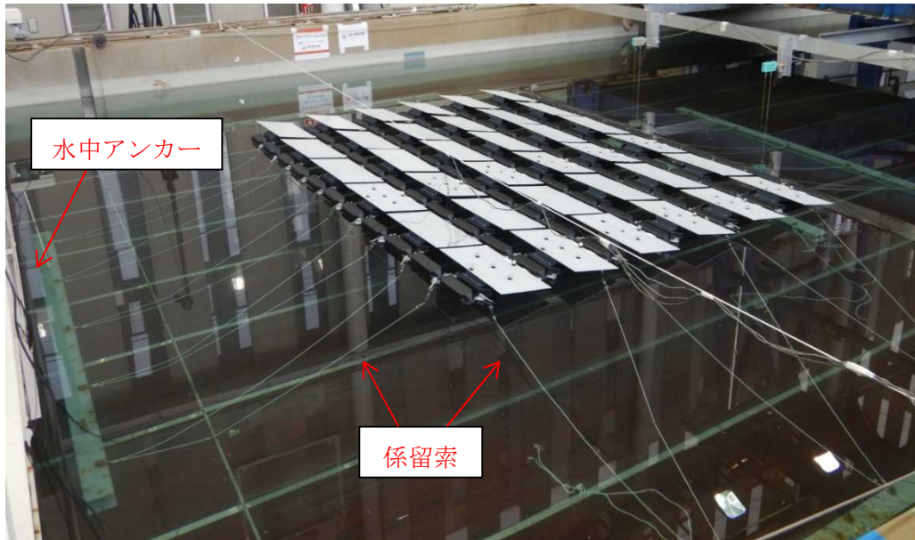
(a) アイランドの係留状況(矩形アイランド)
