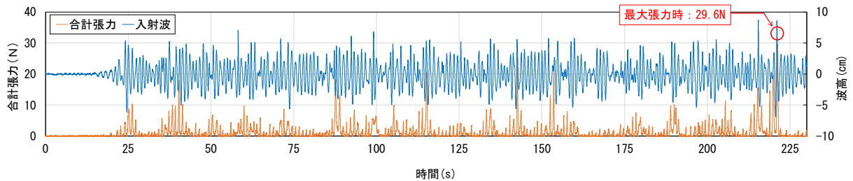
(a) 時系列の合計張力と入射波（ケース名：F6_IW08-10）
