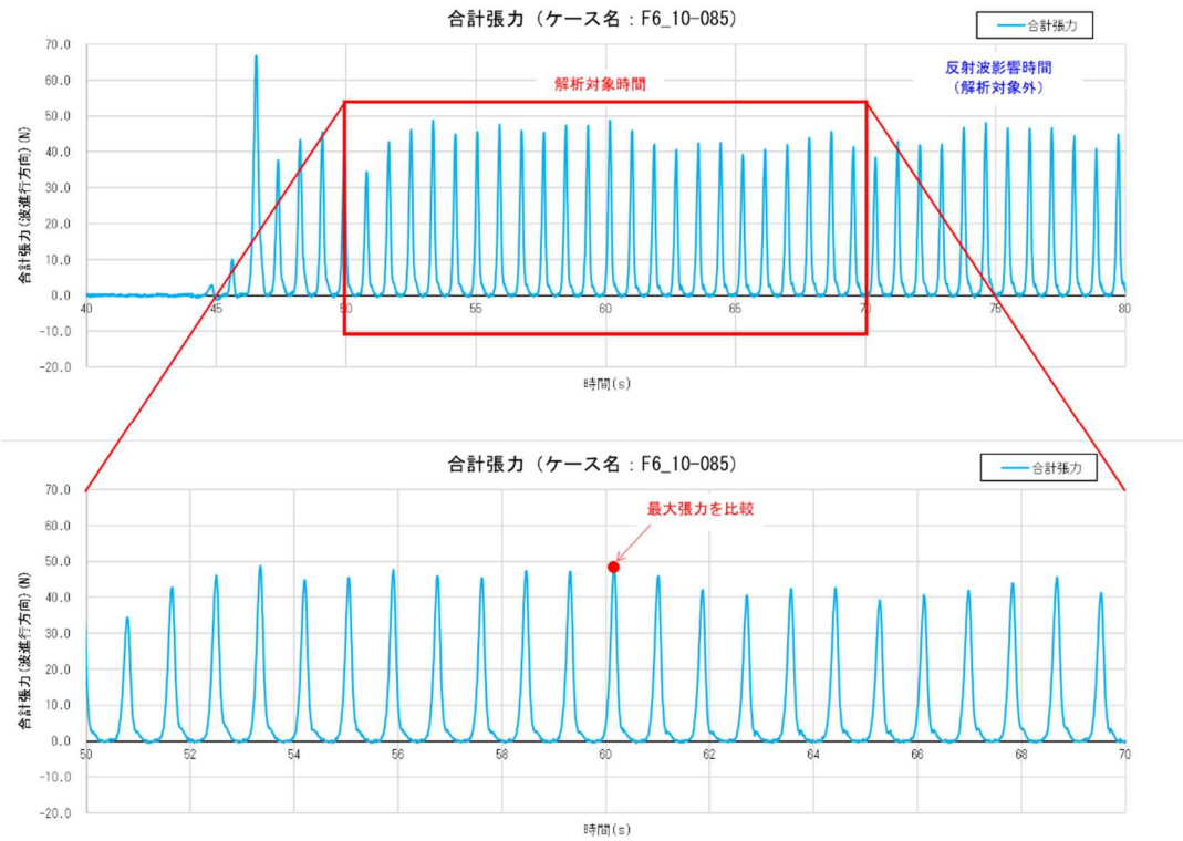
(a) 規則波実験における張力の解析対象時間 (ケース名 : F6_10-085)
