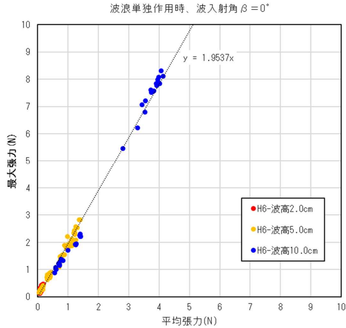
図 5-11 波浪単独作用時の最大張力と平均張力の比較
