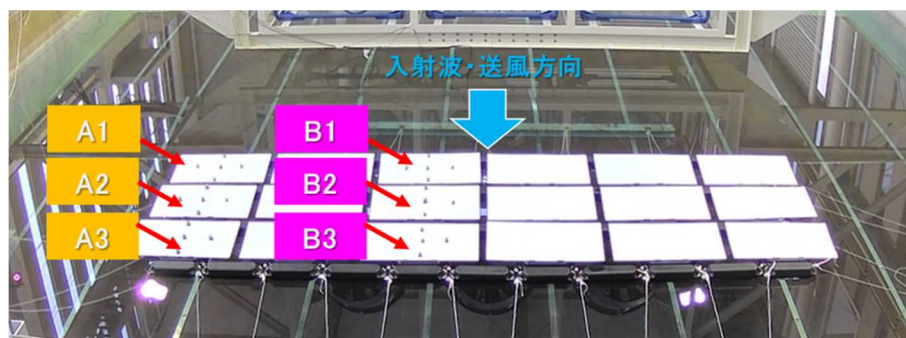
図 5-16 (2/2) トラッカーの設置箇所(フロート 3 列)
