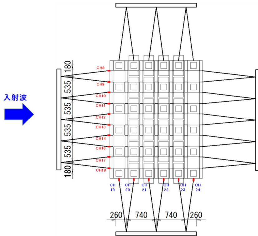
(a) 矩形アイランドでの張力計（リングゲージ）設置箇所
