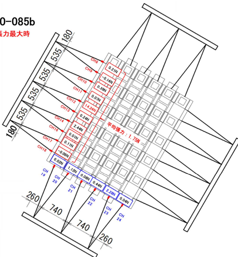
図 5-12 被災波相当波浪の波入射角 \beta = 30^\circ (H6_10-085b) における張力の分散状況
