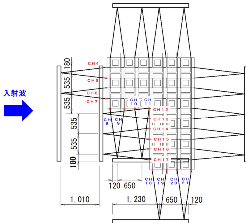
(b) L字型アイランドでの張力計（リングゲージ）設置箇所
