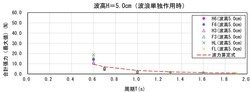
図 5-5 計測値と計算値の比較結果（波高 H=5.0cm）
