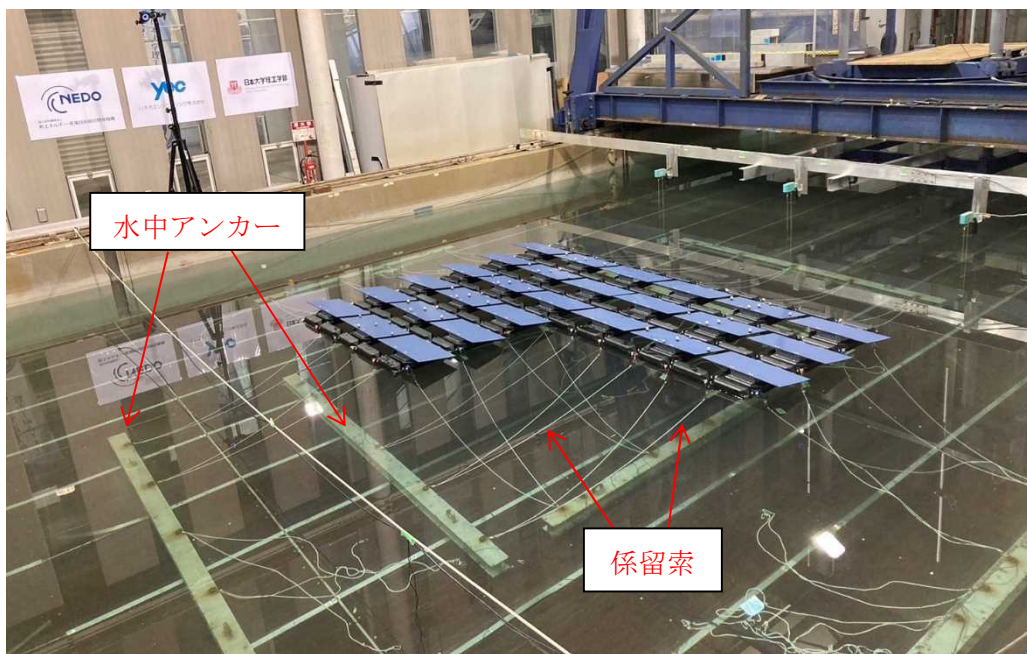
(b) アイランドの係留状況(L字型アイランド)
