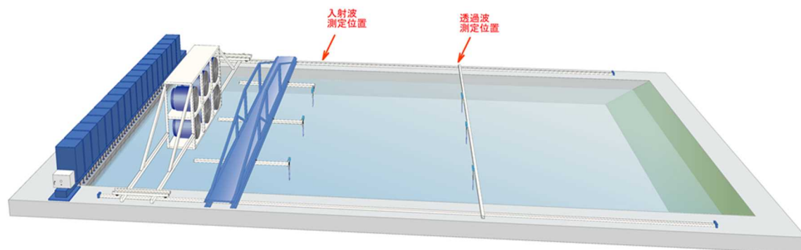
図 4-1 波高検定イメージ
