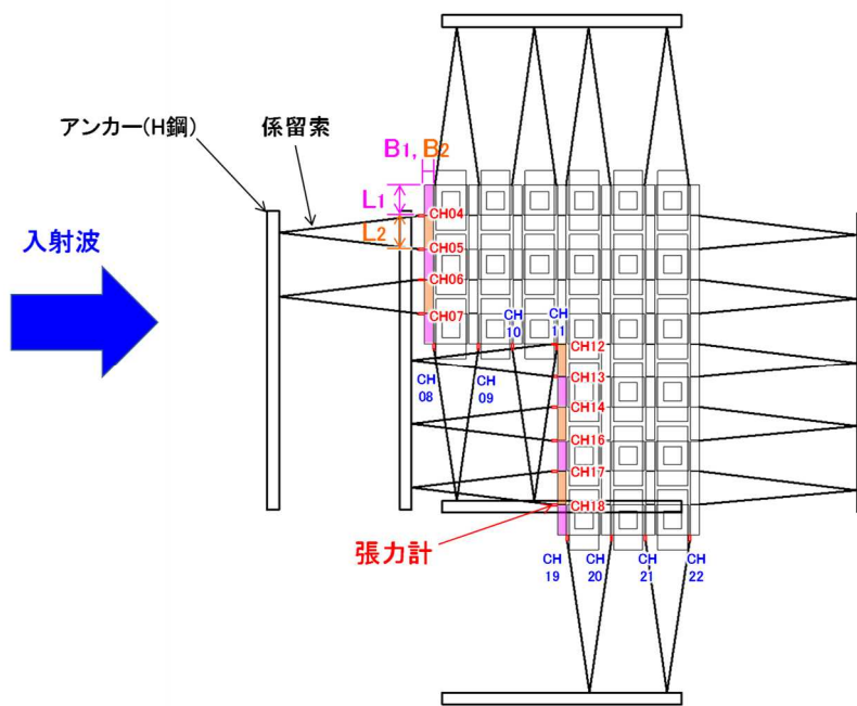
(b) L字型アイランドでの波力算定方式の模式図 (平面図)
