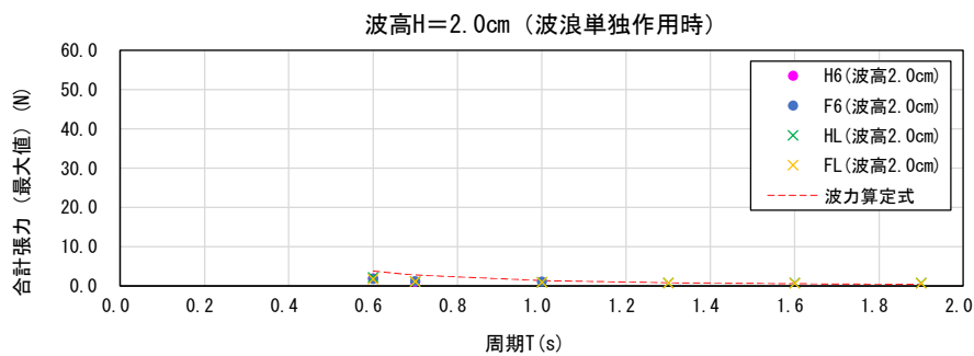
図 5-4 計測値と計算値の比較結果（波高 H=2.0cm）
