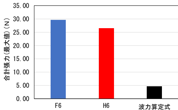
図 5-13 計測値と計算値の比較結果
