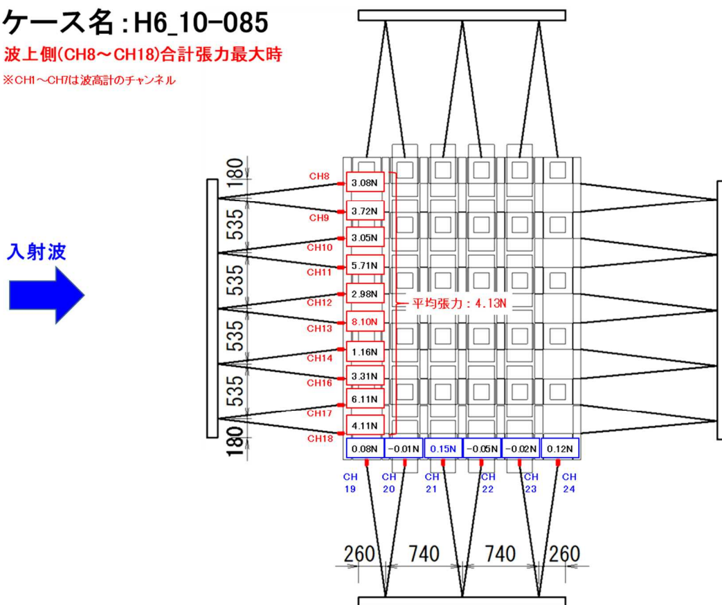
図 5-10 被災波相当波浪 (H6_10-085) における張力の分散状況
