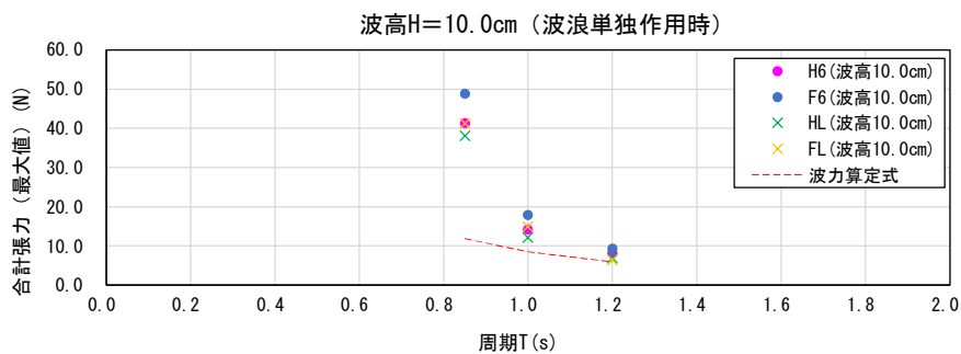
図 5-6 計測値と計算値の比較結果（波高 H=10.0cm）
