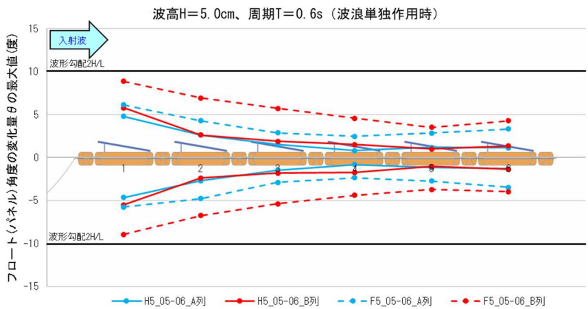
図 5-19 短周期のケースにおけるフロート(パネル)の傾斜角と波形勾配の比較(波高 5.0cm)
