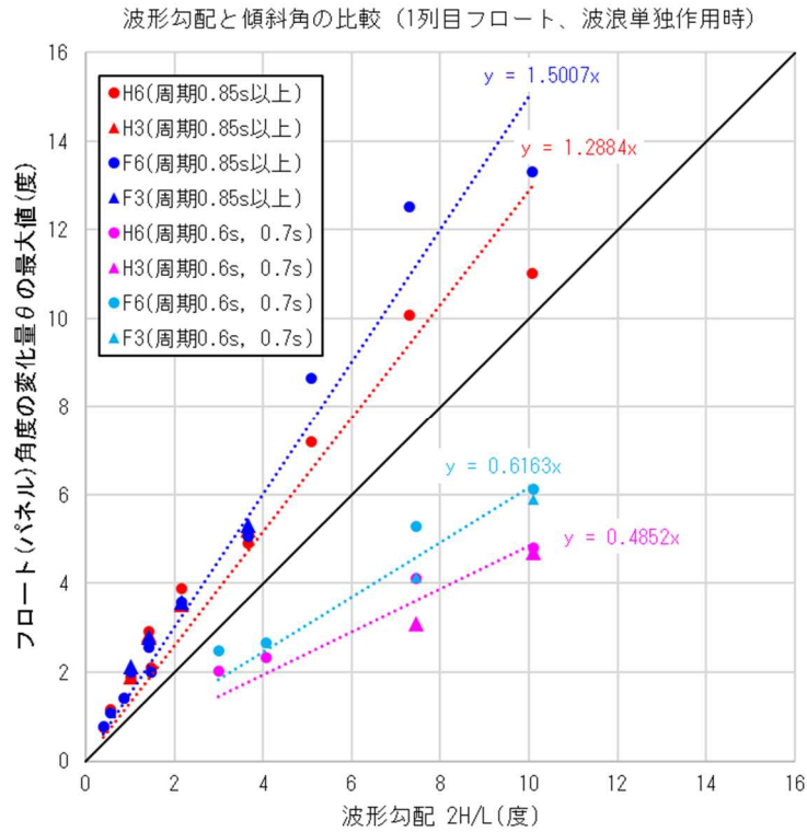
図 5-22 波上側 1 列目におけるフロート（パネル）の傾斜角と波形勾配の比較
