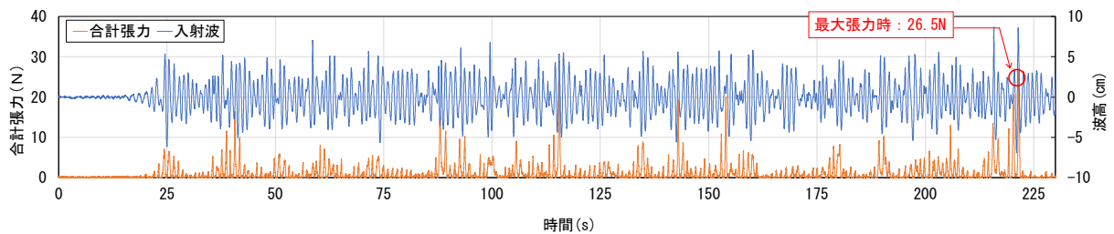
(b) 時系列の合計張力と入射波（ケース名：H6_IW08-10）
