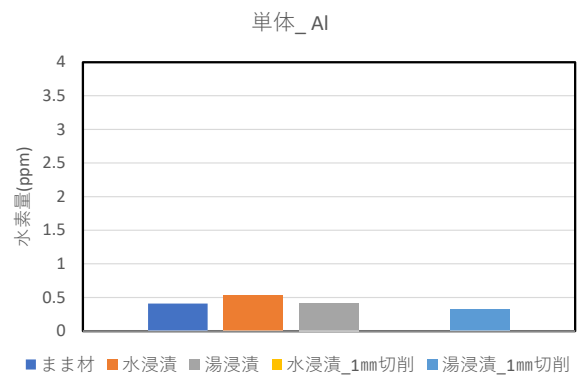
図 3-2.9.3-18 Al合金単体浸漬時の水素量
