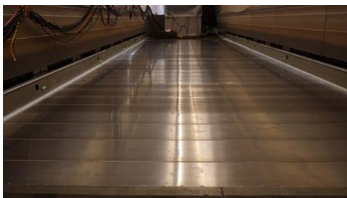
図 3-2.9.4①-8 実車両に適用された難燃性マグネシウム合金製客室床（幅 3m、長さ 9m）
