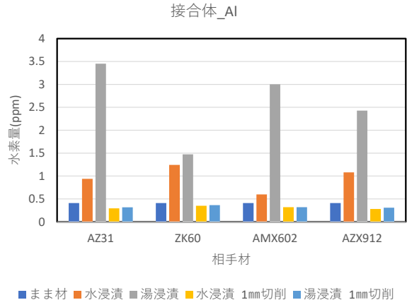
図 3-2.9.3-20 Mg-Al 接合体浸漬時の水素量
