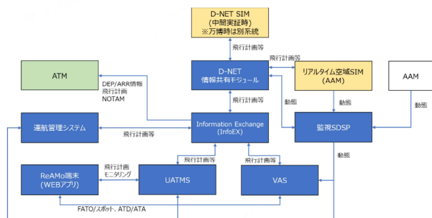
UATMシステム構成
