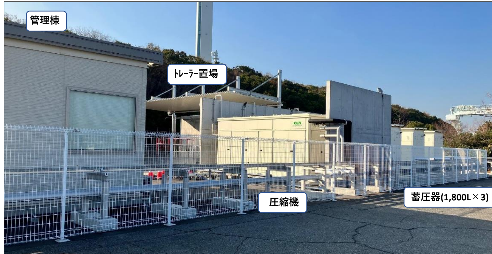
水素ステーション (トレーラー置場、圧縮機、蓄圧器など)
