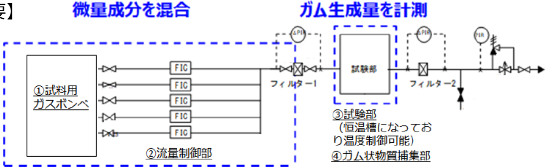
図 試験装置(イメージ図)
