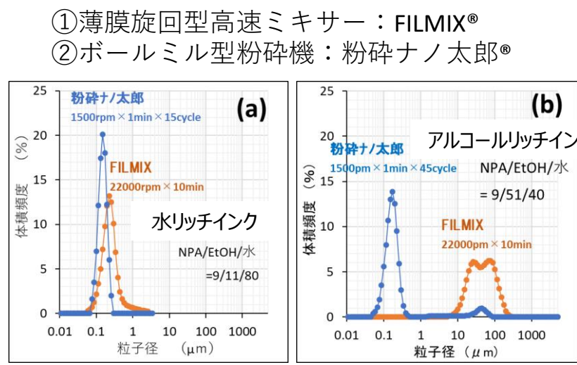
攪拌装置違いのインク粒度分布比較 (a) 水リッチインク (b) アルコールリッチインク
