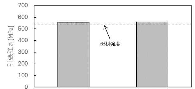
引張試験結果
