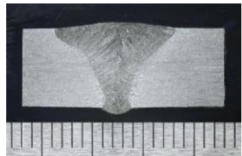
プラズマ溶接試験
