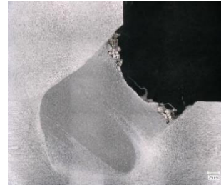
すみ肉断面
