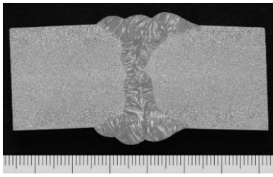
両面SAW溶接工法
