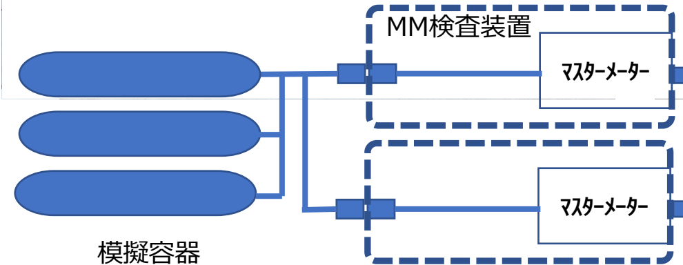
計量試験時概略フロー
