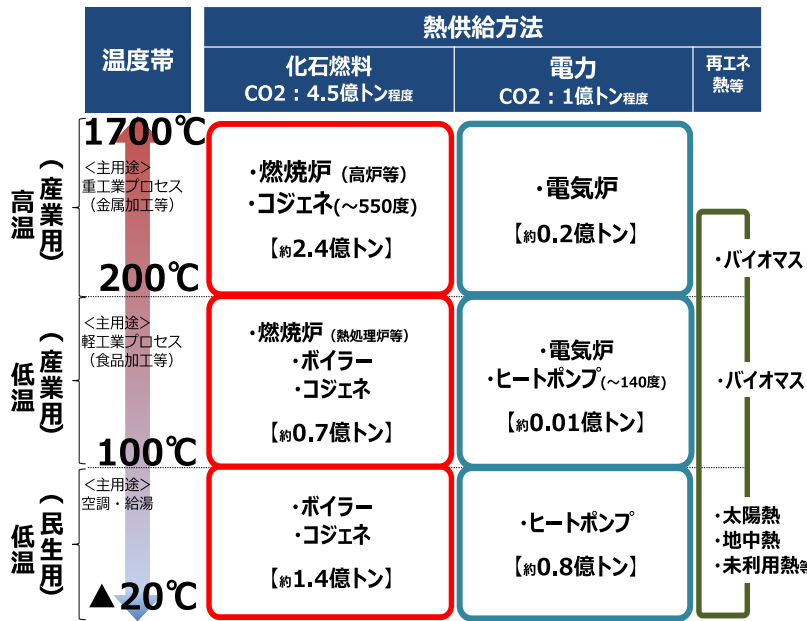
図 熱供給の温度とCO 2 排出量の関係 出所：資源エネルギー庁 第23回基本政策分科会「資料1. 2030年エネルギーミックス実現のための対策 ~原子力・火力・化石燃料・熱~」(2017年) p.56を基にNEDO技術戦略センター作成
