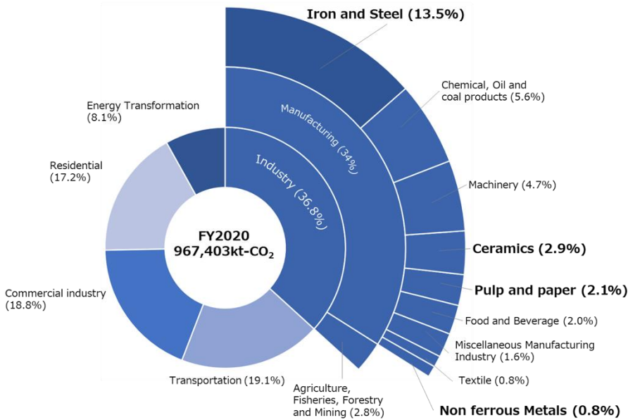
図 日本のCO 2 排出量の内訳 2020年度の国内のCO 2 排出量は1,044百万t エネルギー起源は967百万t 工業プロセスから排出されるCO 2 は186百万t(約19%)
