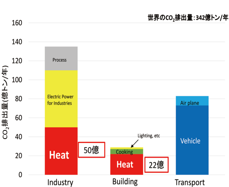
図 世界のCO 2 排出量の内訳 出所：IEA「Energy Technology Perspectives 2017」等を 基に NEDO 技術戦略研究センター作成
