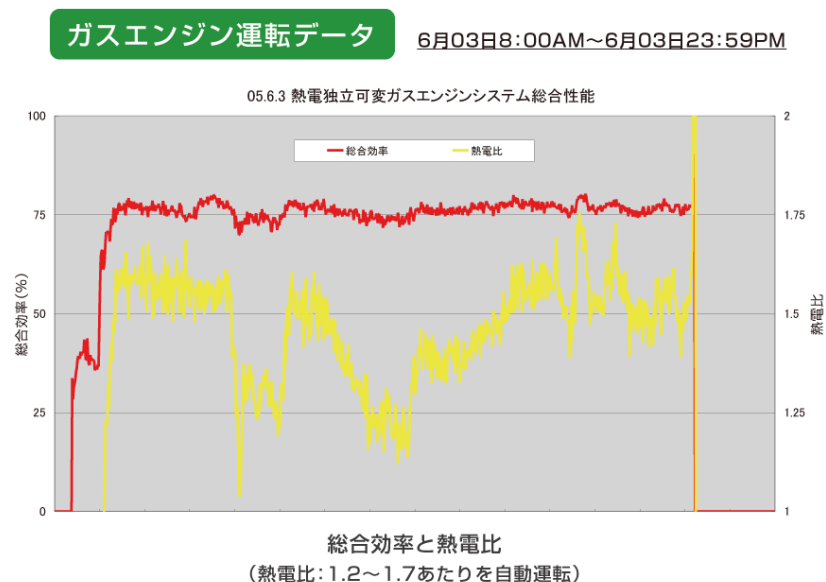
図10 6月に実施した試験運転での総合効率と熱電比の時間変化。8時～24時までの間に、熱電比1.2～1.7あたりで変動している。
