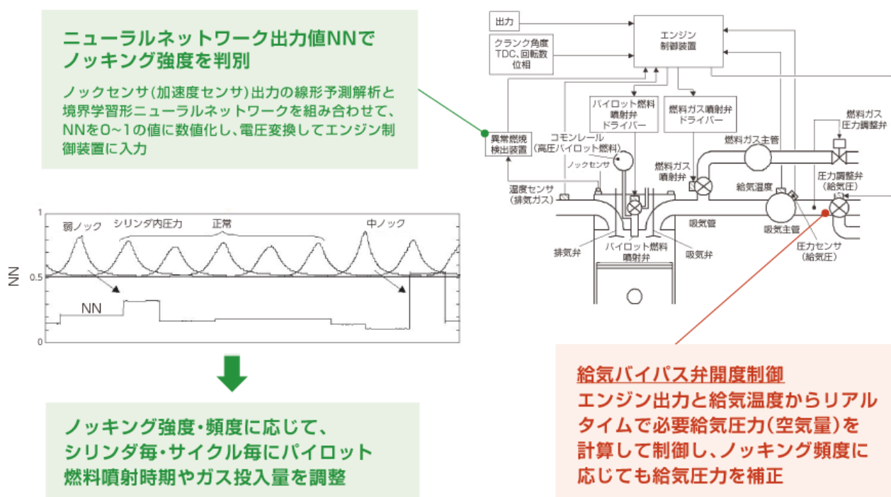
図8 ノッキング防止技術
