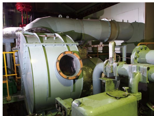
過給機の空気取り入れ口
