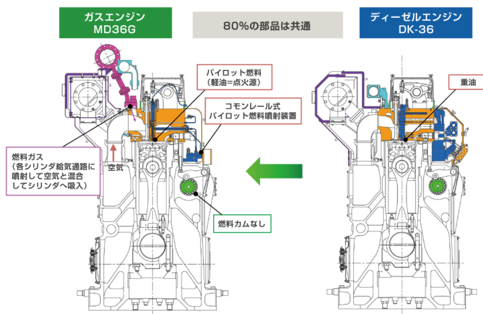
図A ガスエンジンとディーゼルエンジンの構造比較。
