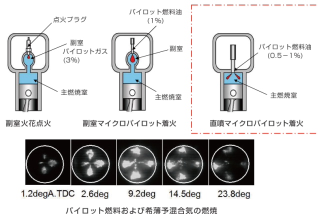
図4 ガスエンジンの着火方式
