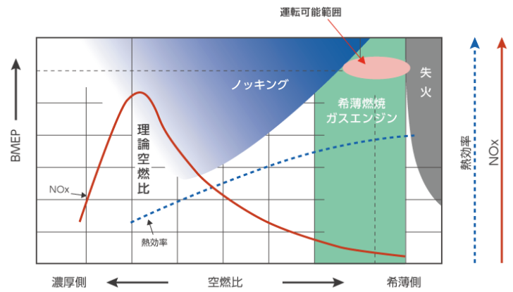
図9 ノッキングの発生頻度を低く抑えるための運転条件。 ノッキング頻発条件と失火条件の中間部分にある、極めて 狭い範囲で空燃比を安定させることで、エンジンの出力を 落とすことなくノッキングの頻度を抑え込むことに成功
