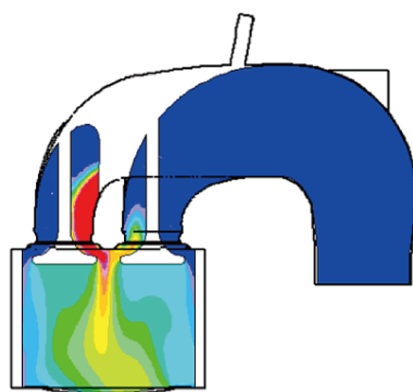
図5 吸入工程における燃料ガスと 空気の混合の解析例
