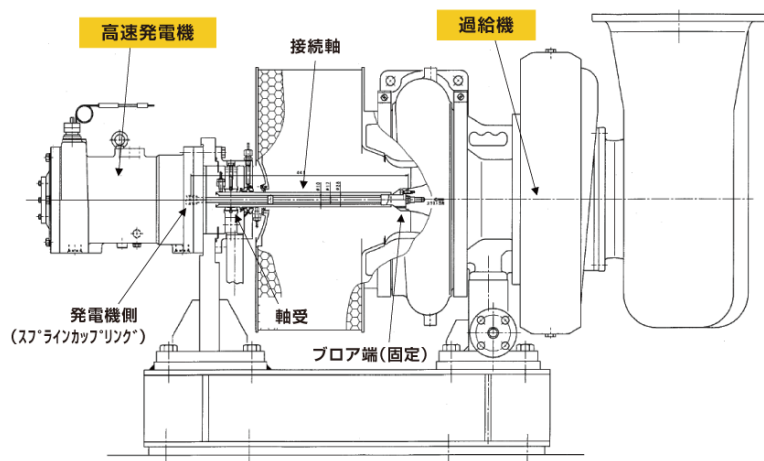
図7 過給機に直接発電機を接続した排気エネルギー回収システム
