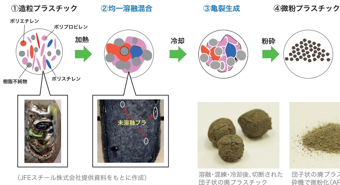
図7 プラスチックの脆性破壊のメカニズム
