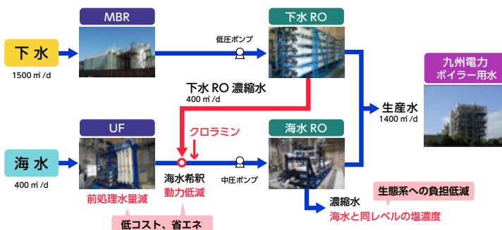
図 1 「海淡・下水再利用統合システム」全体の工程（資料提供：GWSTA）
