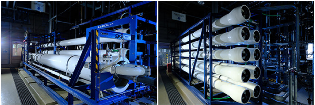
写真4 「ウォータープラザ北九州」に設置された海水RO膜(左)と、下水RO膜(右)
